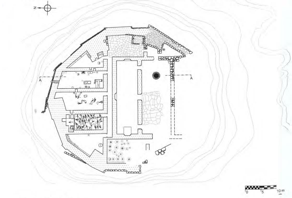
Çizim 6. 6. Giriktepe Sarayı Planı (Schachner, 2021: Res. 4)
