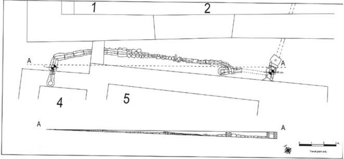
Çizim 6. 4. Yamuk Planlı Avludaki Kanaletin Plan ve Kesit Çizimi (Karaosmanoğlu ve Yılmaz, 2012: Fig. 6)
