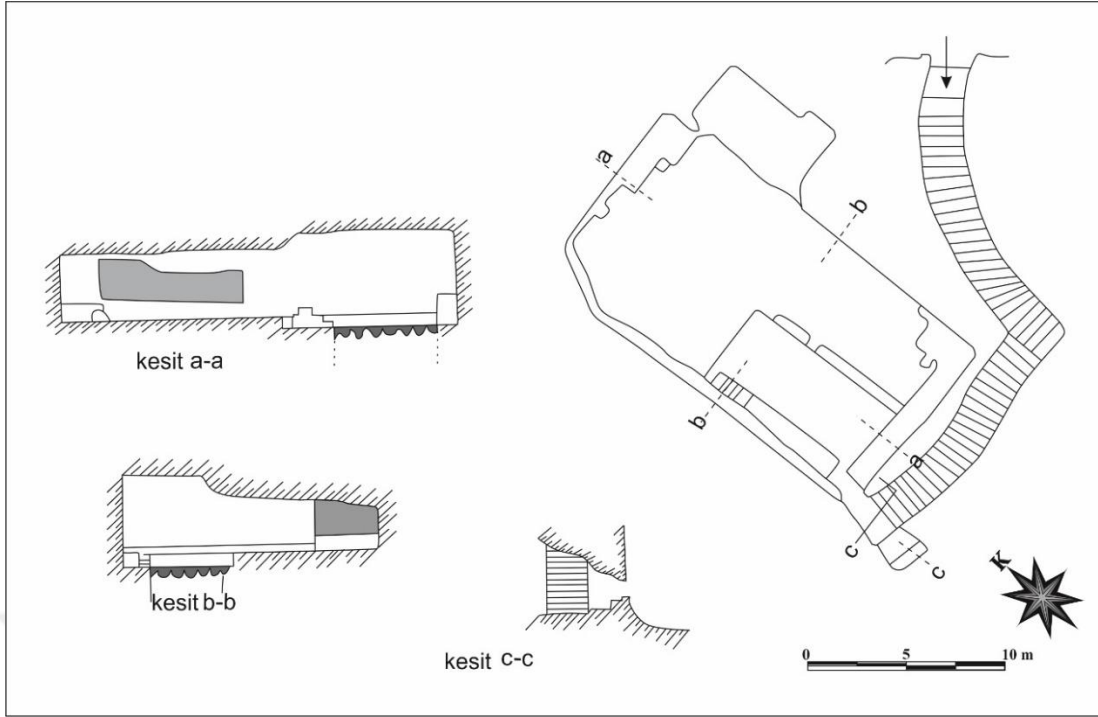
Çizim 6. 10. Toprakkale Sarnıcı Plan ve Kesitleri (Erzen, 1977: Res. 19'dan düzenlenmiş çizim)
