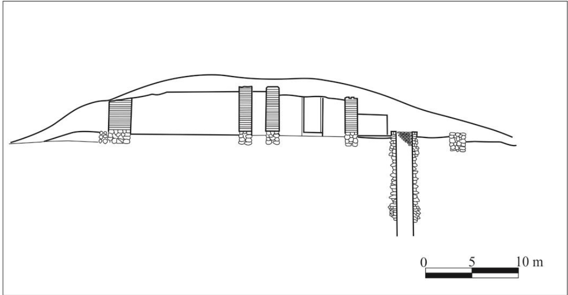
Çizim 6. 7. Giriktepe Sarayı Planı Kesiti (Schachner, 2021: Res. 5'den düzenlenmiş çizim)
