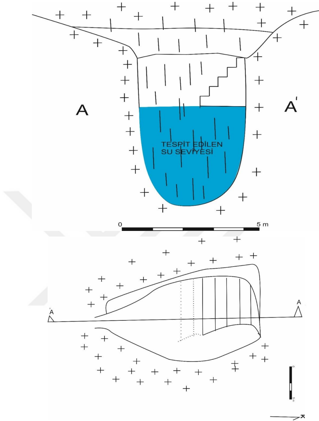
Çizim 6. 9. Bostankaya Kalesi Doğu Sarnıcı Çizim ve Kesiti
