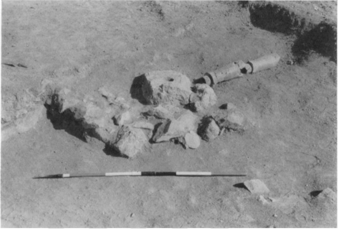
Resim 6. 16. Kayalıdere Kalesi Drenaj Boruları ve Taşı ( in situ ) (Burney, 1966: Pl. XIIIb)
