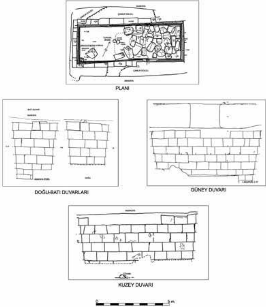
Çizim 7. 3. Çavuştepe 1 No'lu Sarnıç Duvarları (Çavuşoğlu ve ark. 2016: Çiz. 3)
