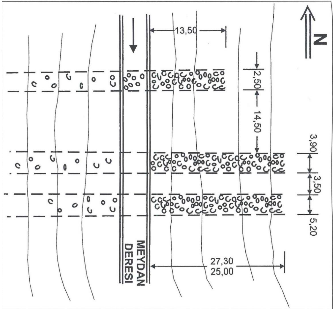
Çizim 6. 17. Airi Baraj Göleti Bendini Oluşturan Duvarlar ve Dolgu (Garbrecht, 2004:
