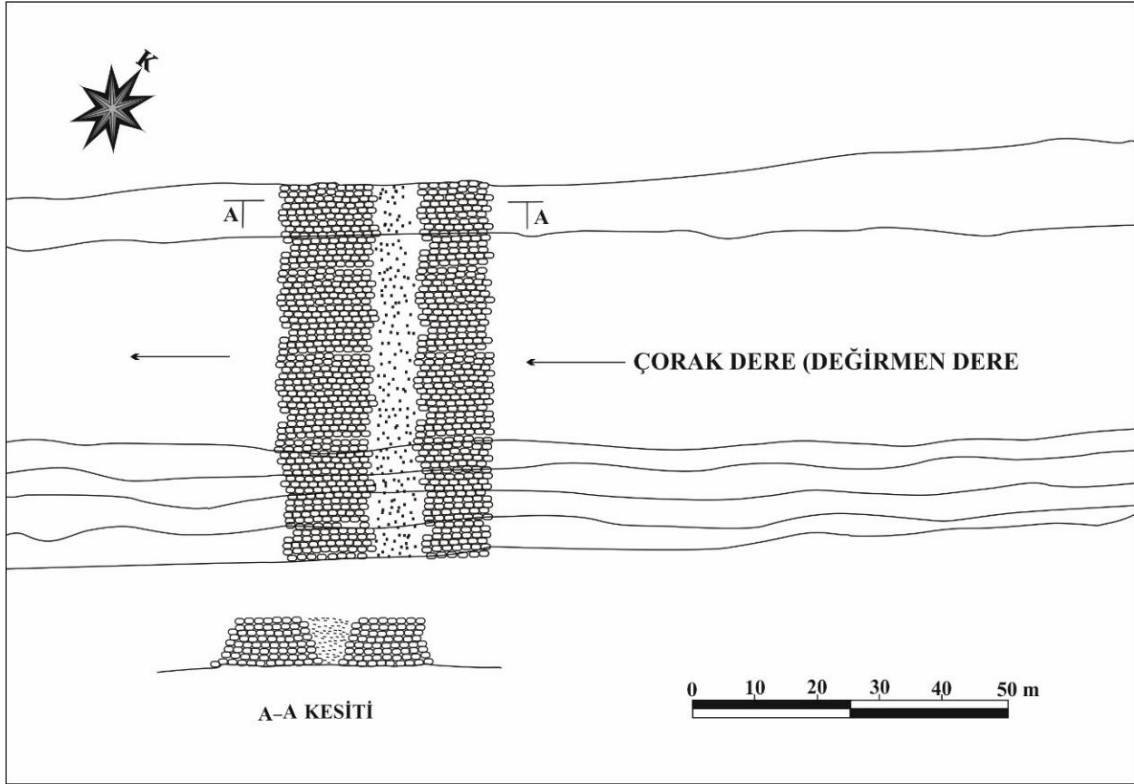
Çizim 6. 19. Köşebaşı Baraj Bendi ve Kesiti (Belli, 1997b: Çiz. 4'ten düzeltilmiş çizim)
