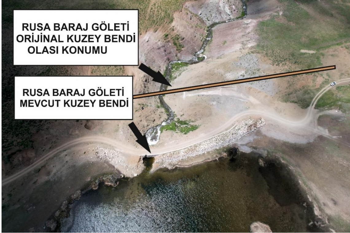
Resim 6. 66. Rusa Baraj Göleti Kuzey Bendi (Hava Fotoğrafı)
