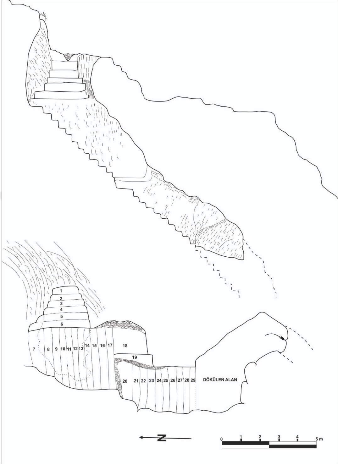
Çizim 6. 11. Qal'eh Heydari Kayaya Açılan Basamaklı Tüneli (Kleiss, 1976: Abb. 7'den düzenlenmiş çizim)
