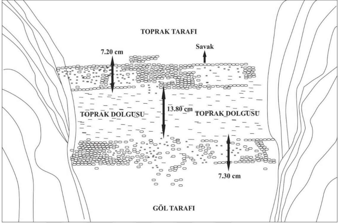
Çizim 6. 16. Rusa Baraj Göleti Batı Bendi
