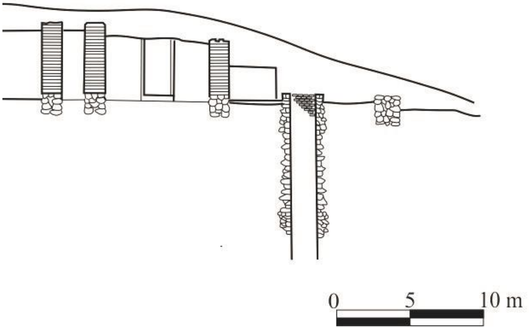
Çizim 7. 3. Giriktepe Sarayı Su Kuyusu Kesiti (Schachner, 2021: Res. 5)
