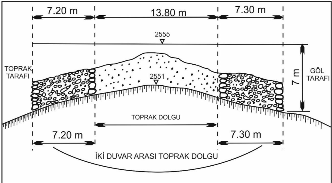
Çizim 7. 1. Rusa Barajı Batı Bendi Kesiti
