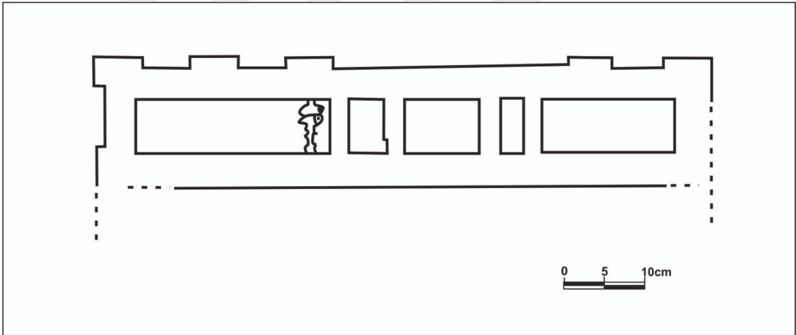
Çizim 6. 5. Keçikıran Kalesi Batı Etekteki Yapının Planı ve Drenaj Sistemi (Sevin, 2006: Res. 19'dan düzenlenmiş çizim)
