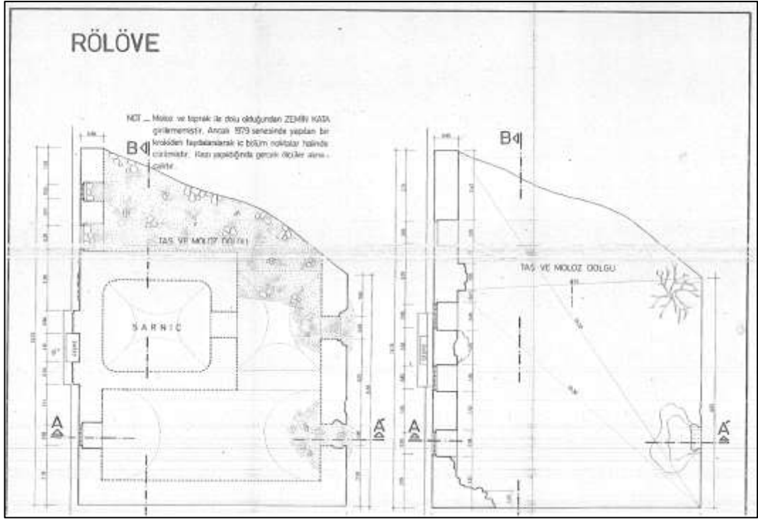
Şekil 6.10. 18.10.1990 tarih ve 2417 sayılı III numaralı KVTVKK onaylı rölöve planı [32].
