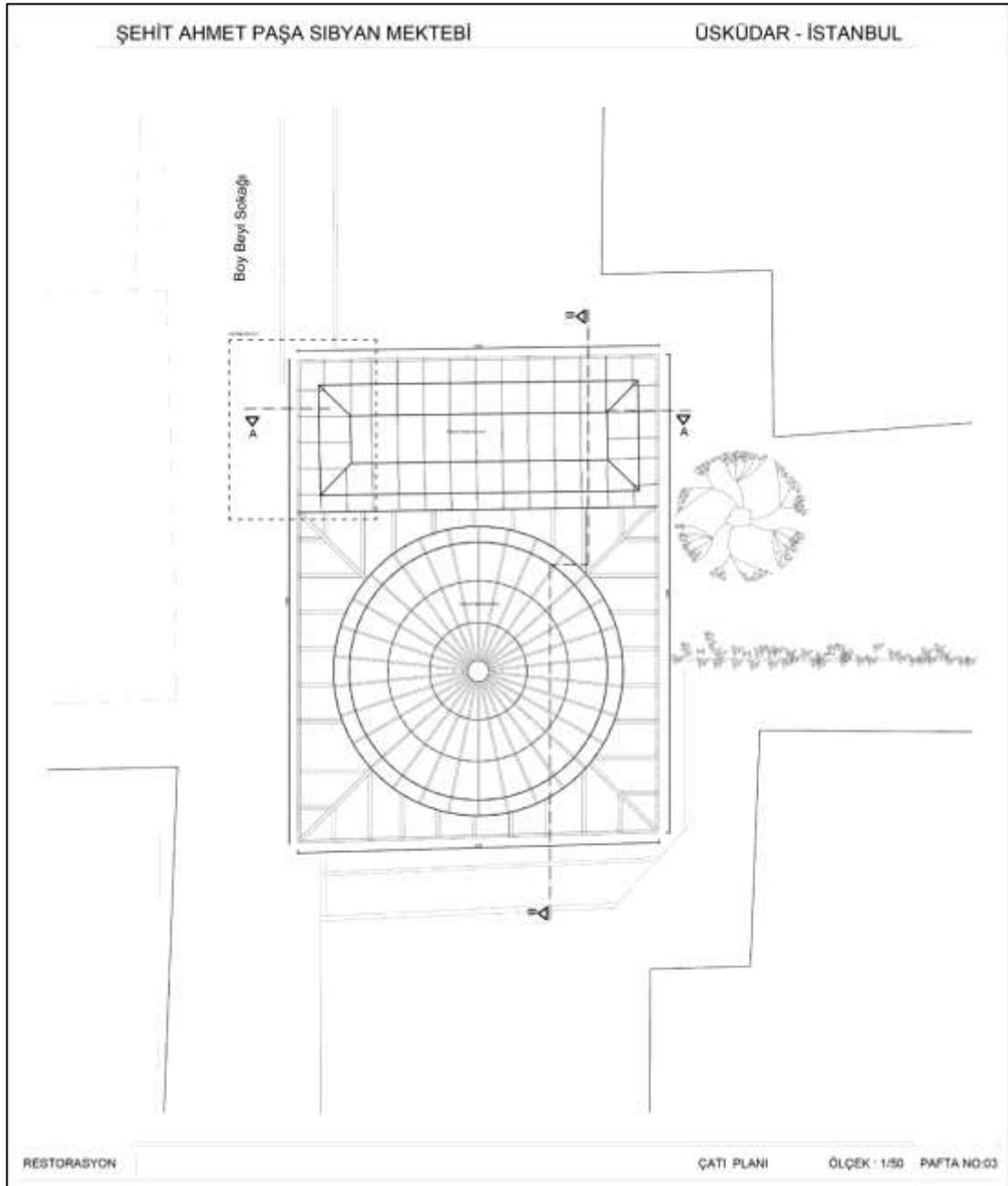
Şekil 7.18. Çatı planı.
