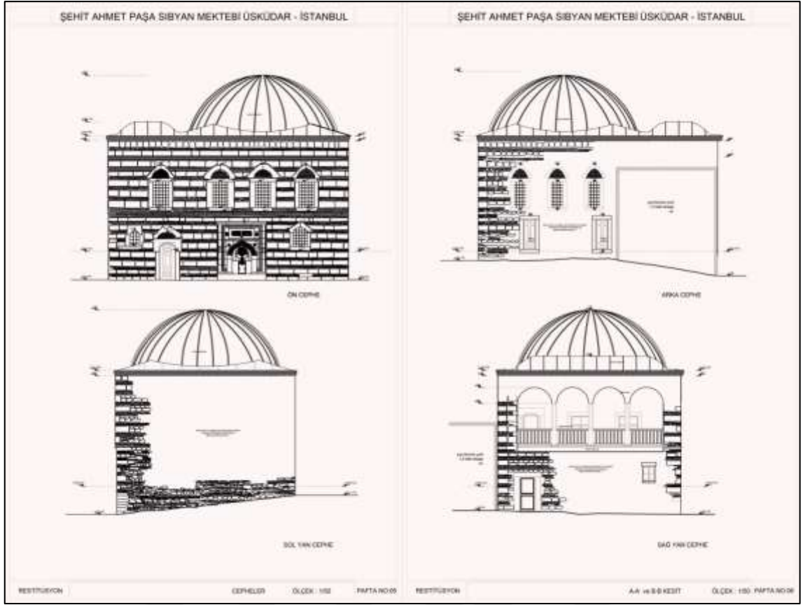
Şekil 7.28. Restitüsyon cephe çizimi.
