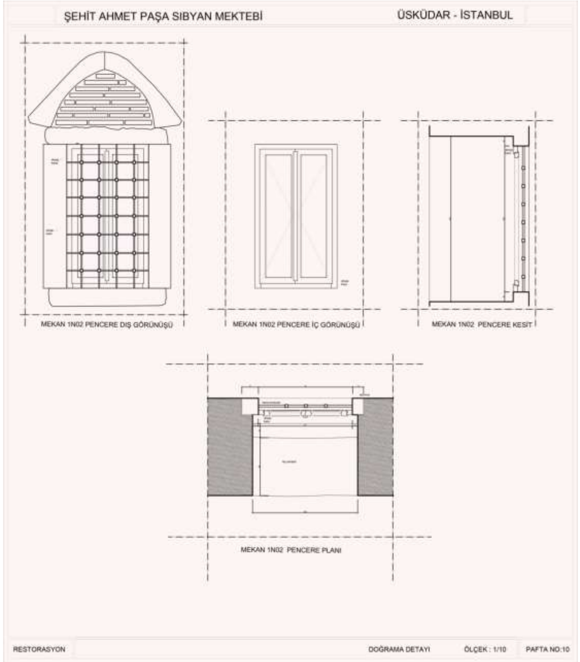
Şekil 8.24. Restorasyon projesi doğrama detayı.
