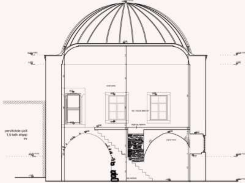
A - A KESİTİ
