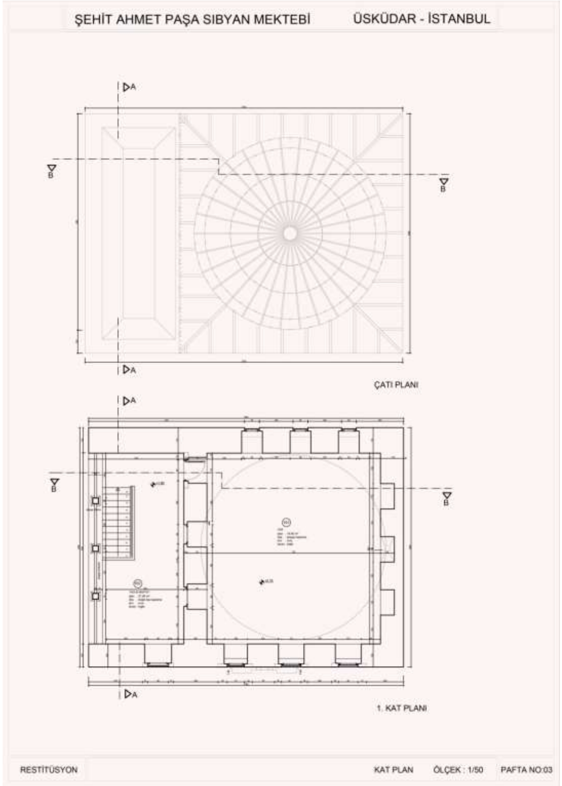
Şekil 7.26. Restitüsyon üst kat planı.
