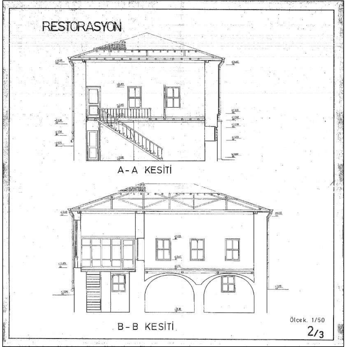
Şekil 7.12. 1994 yılına ait KVTVKK onaylı restorasyon projesi kesitler [32].
