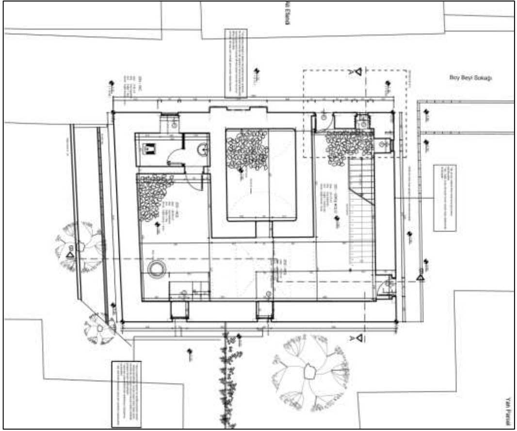
Şekil 8.29. Vaziyet planı.
