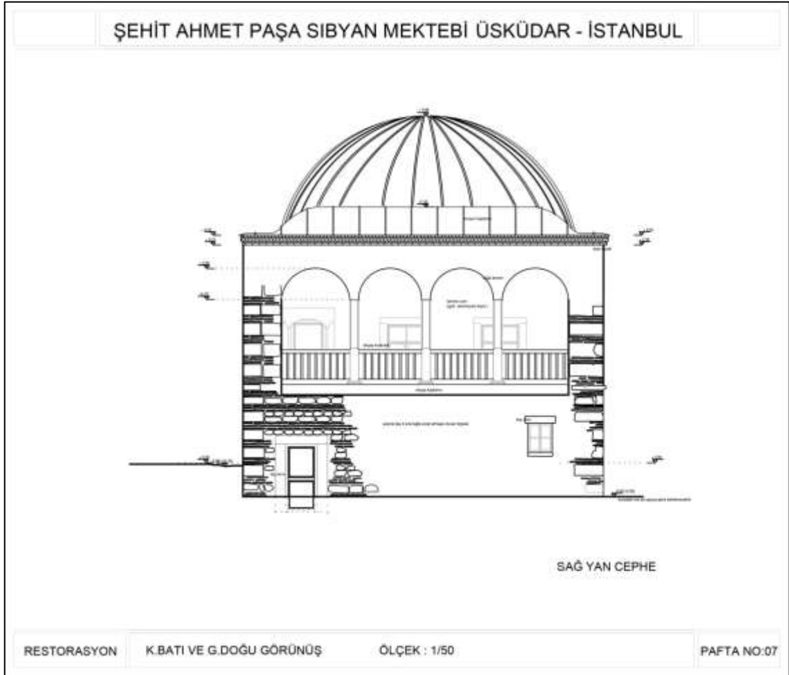
Şekil 7.22. Sağ yan cephe çizimi.
