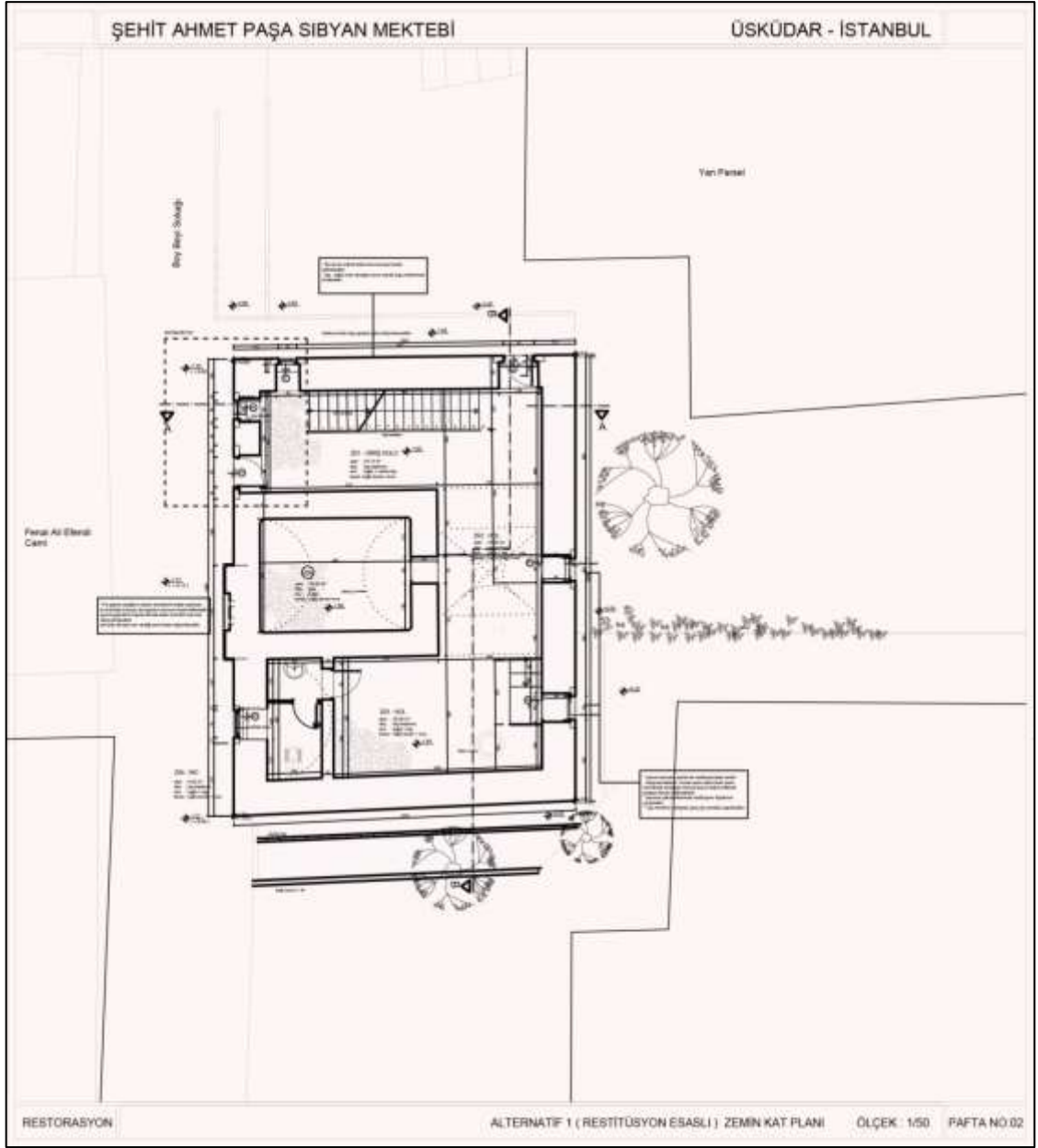
Şekil 7.15. Zemin kat planı.
