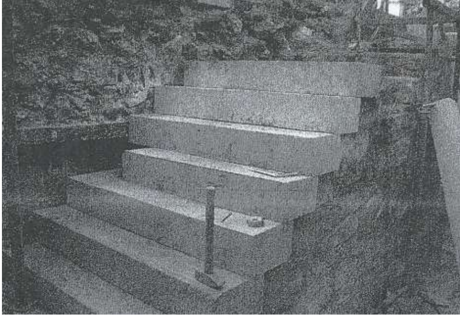
Şekil 8.21. 2013 yılı onarımı kesme taş merdiven uygulaması.
