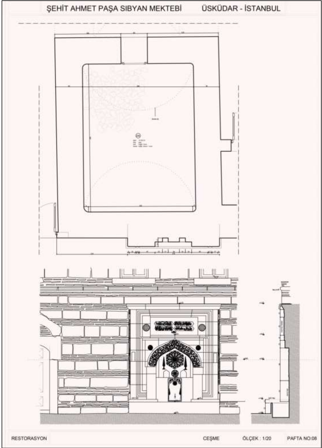
Şekil 6.4. Restorasyon projesi çeşme plan ve ön cephe çizimi.
