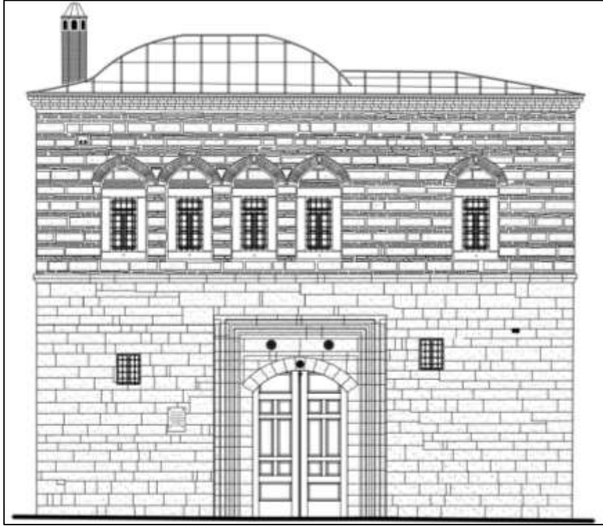
Şekil 4.2. Balaban Ağa caddesi cephesi.
