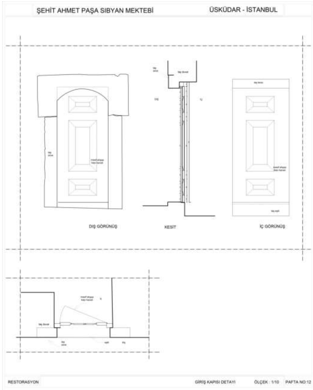
Şekil 8.25. Restorasyon projesi giriş kapısı detayı.
