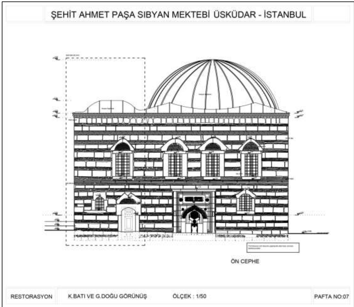
Şekil 7.19. Ön cephe çizimi.
