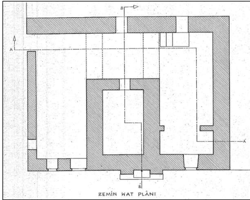
Şekil 7.9. 1961 yılına ait mektebe ait restitüsyon çizimi [32].
