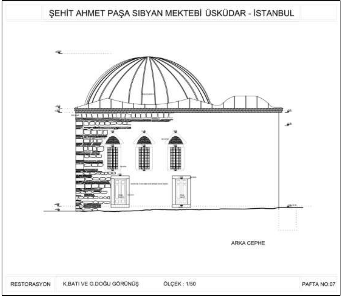
Şekil 7.22. Arka cephe çizimi.
