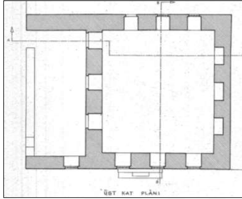
Şekil 7.10. 1961 yılına ait mektebe ait restitüsyon çizimi [32].
