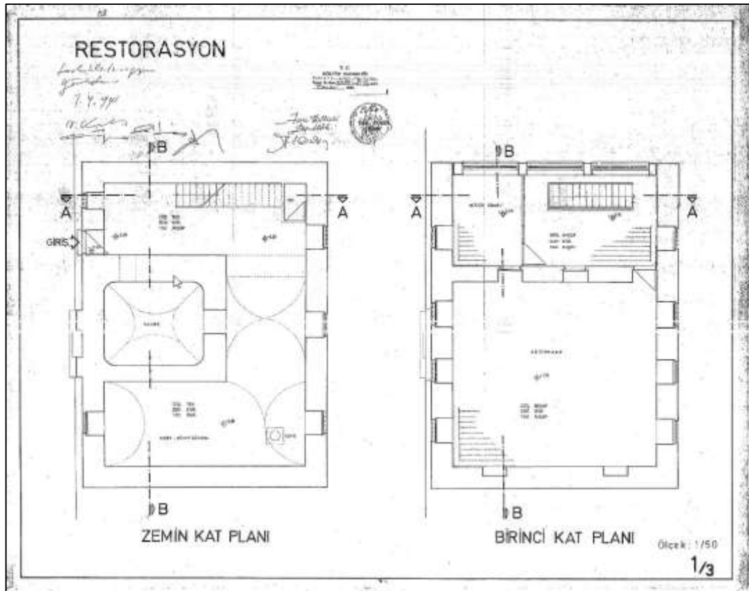
Şekil 7.11. 1994 yılına ait KTVKK onaylı restorasyon projesi kat planı [32].
