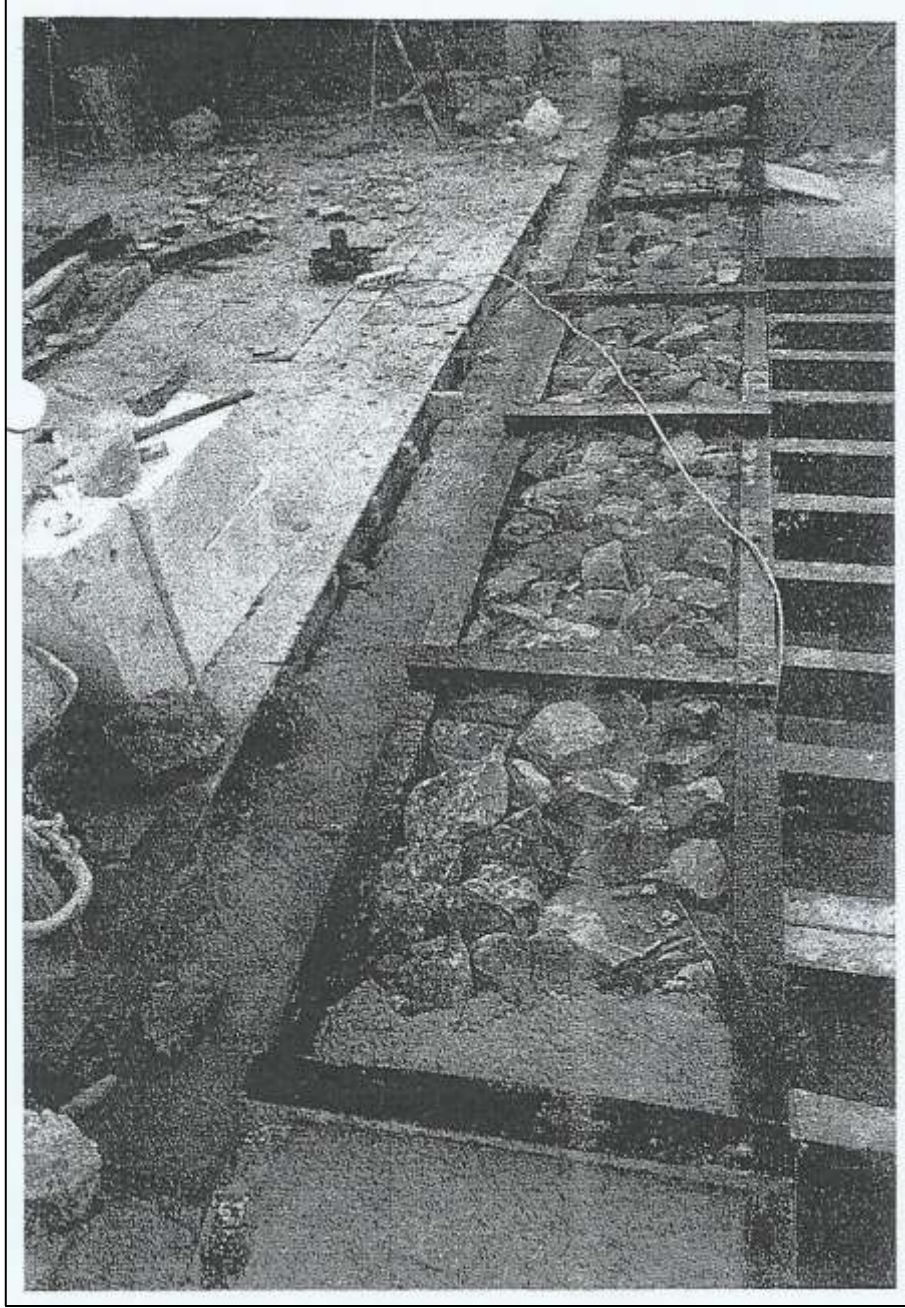
Şekil 8.6. 2013 yılı onarım sırasında uygulanan ahşap hatıllar.
