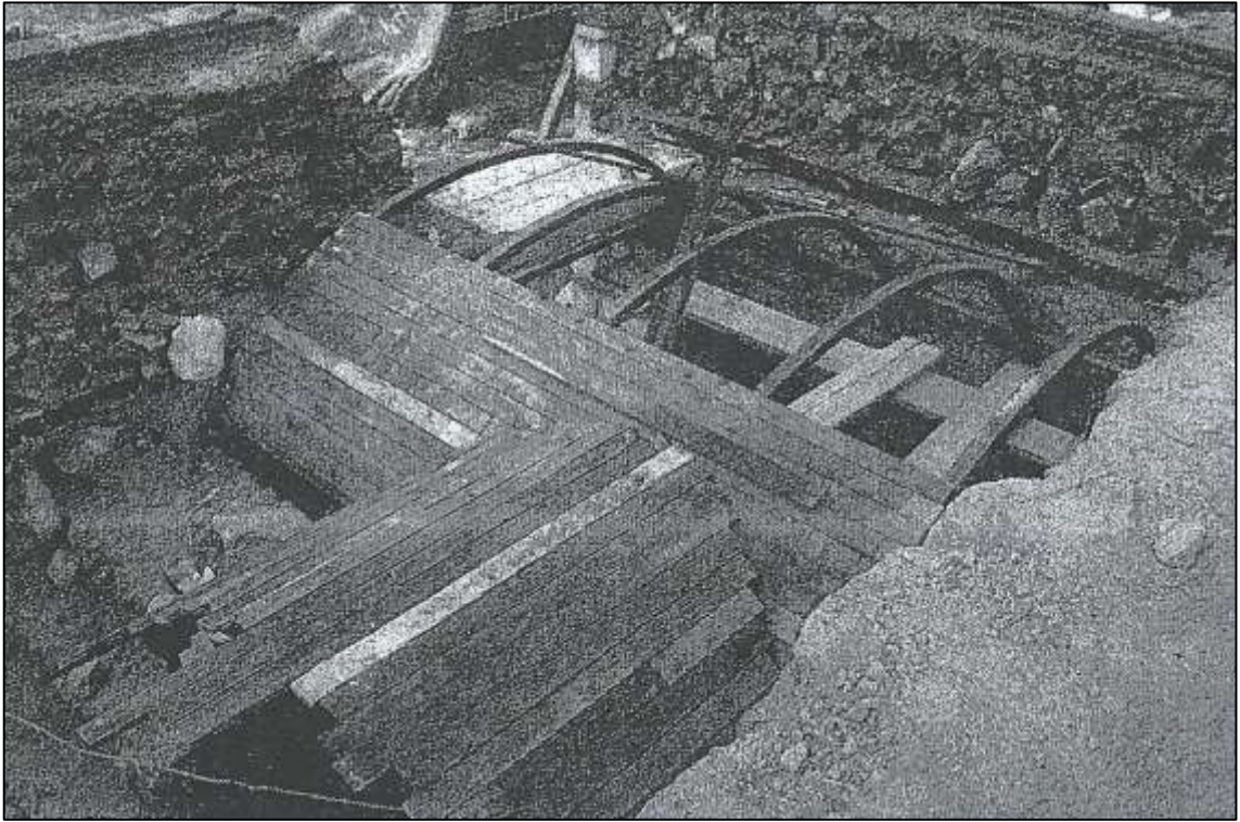
Şekil 8.12. 2013 yılı onarımı zemin kat tonozları kalıbı.
