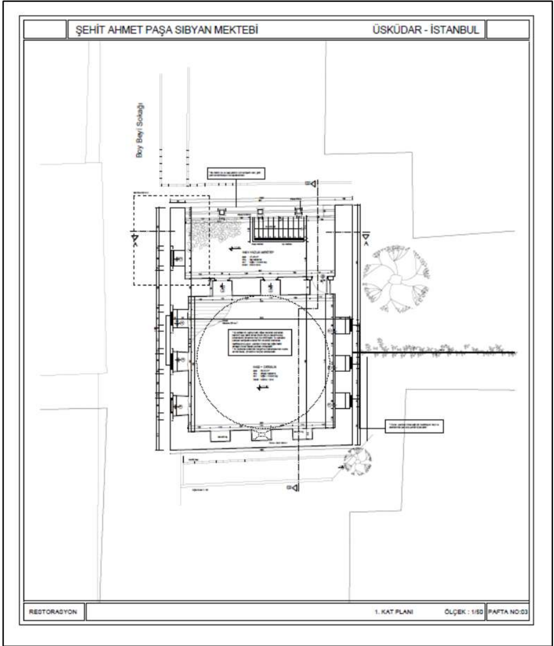
Şekil 7.17. Üst kat planı.
