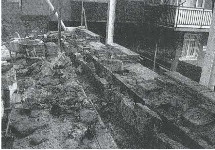
Şekil 8.19. 2013 yılı onarımı kirpi saçak örümü.
