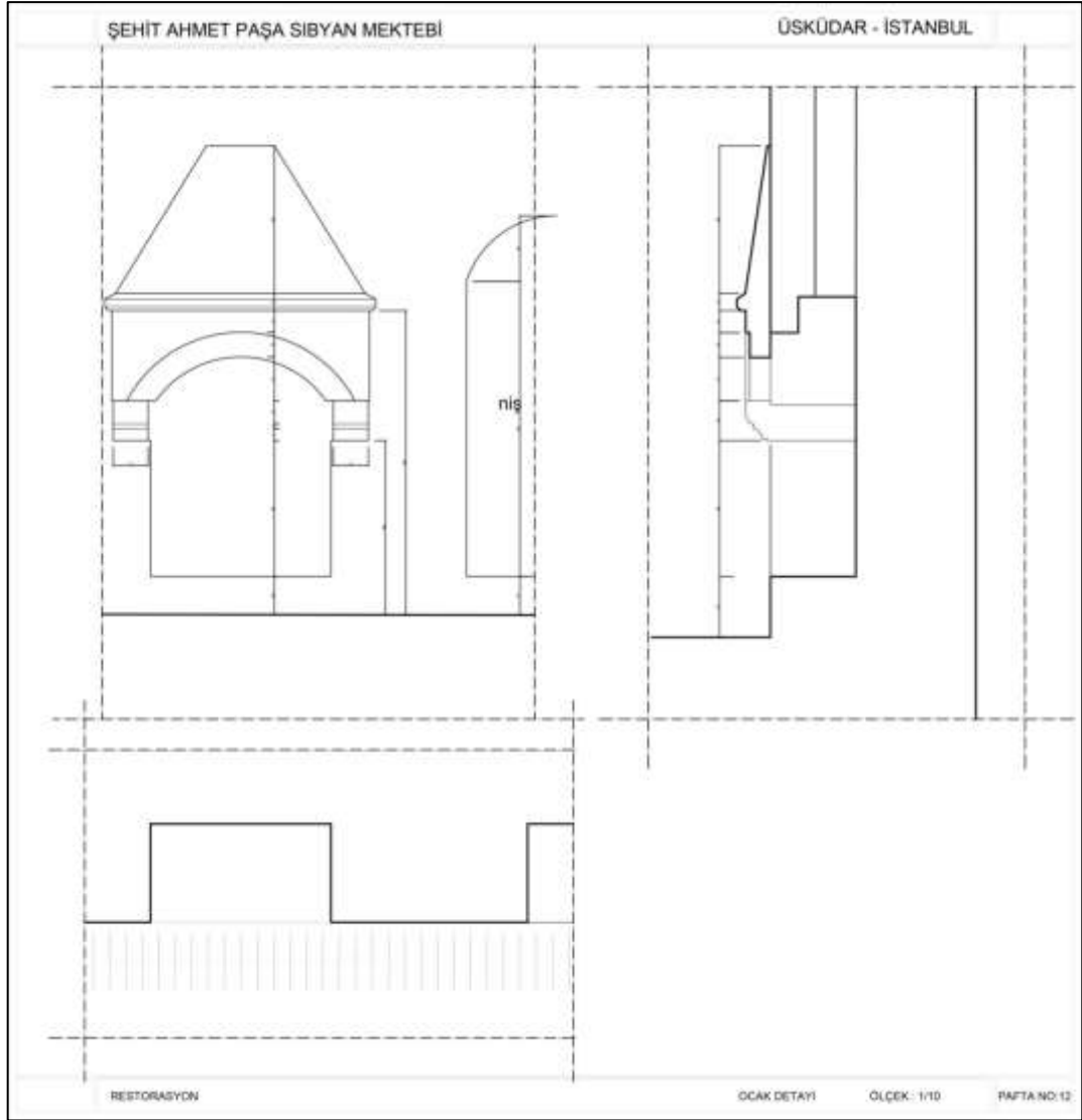
Şekil 8.26. Restorasyon projesi ocak ve yaşmak detayı.
