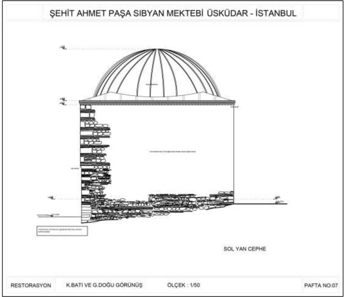
Şekil 7.20. Sol yan cephe çizimi.
