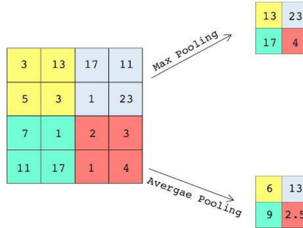
Şekil 2.27. Pooling İşlemi
