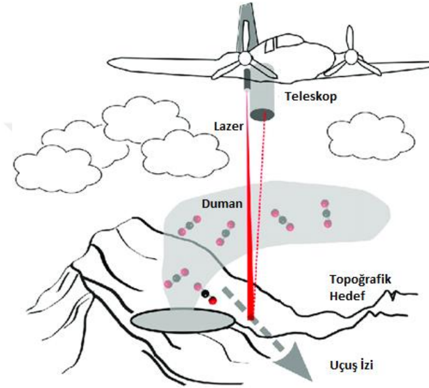
Şekil 2.3. Örnek Bir Hava Platformu Görünümü [16]
