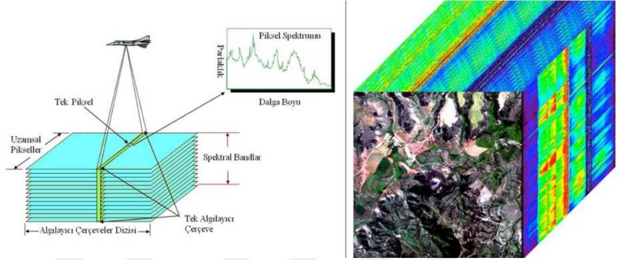
Şekil 2.7. Hiper-spektral Görüntü
