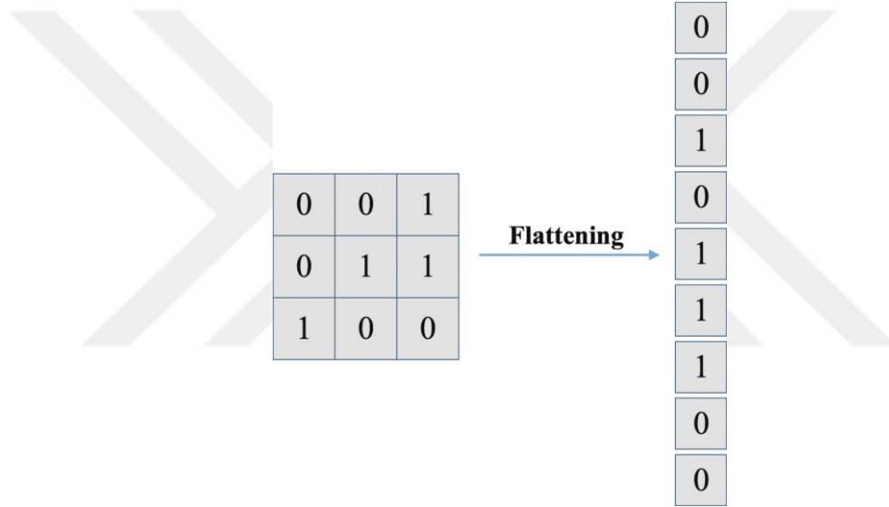
Şekil 2.28. Flattening İşlemi
