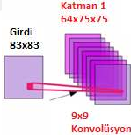
Şekil 2.24. Konvolüsyonel Çıktı
