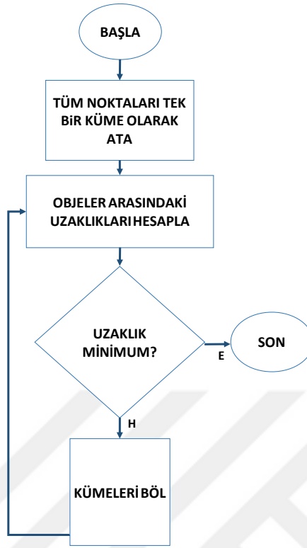
Şekil 3.6 Ayırıştırıcı hiyerarşik sınıflandırma (Roux, 2015)
