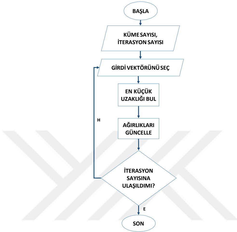
Şekil 3.10 SOM Algoritması (Anifah, Purnomo, Mengko, & Purnama, 2018)
