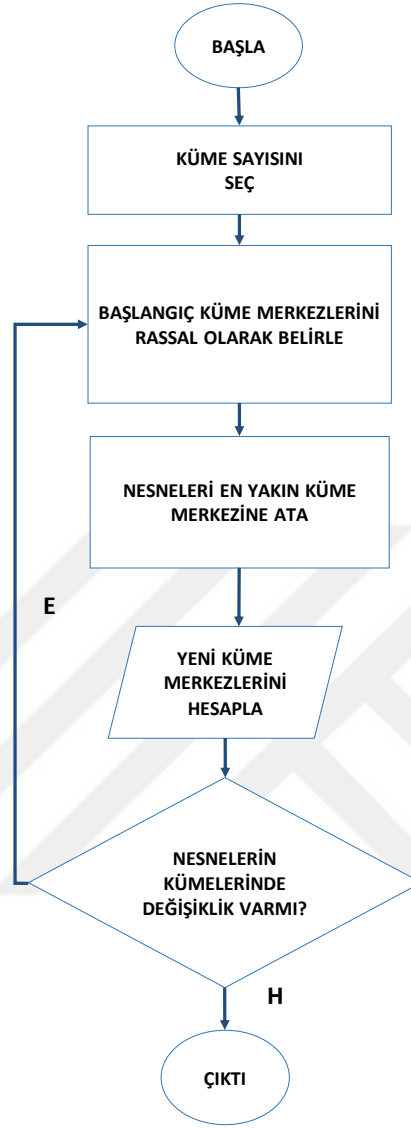
Şekil 3.8 K-Means Algoritması (Younus et al., 2015)
