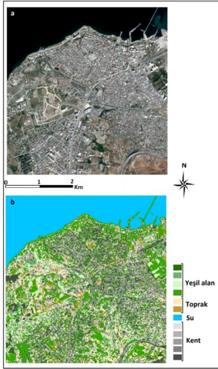
Şekil 6.7 Sonuç Haritası a) Uydu Görüntüsü b) Fuzzy C Means
