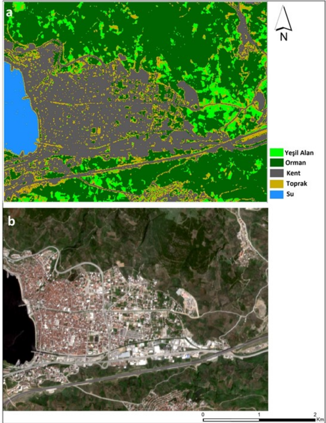
Şekil 6.14 Etiketleme Sonucu a) Uydu Görüntüsü b) Etiketleme Sonucu
