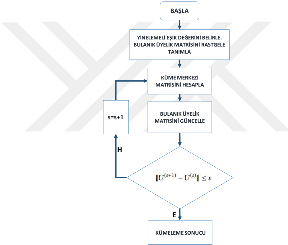
Şekil 3.14 Fuzzy C-Means Algoritması (Wang, Zhao, Wang, Tang, & Li, 2015)
