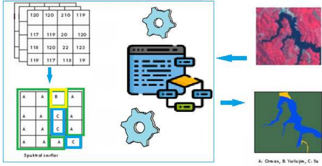
Şekil 3.4 Kontrolsüz Sınıflandırma
