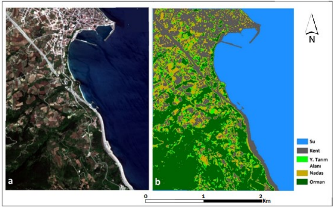
Şekil 6.13 Etiketleme Sonucu a) Uydu Görüntüsü b) Etiketleme Sonucu
