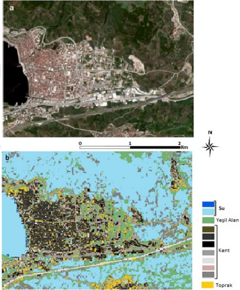
Şekil 6.10 Sonuç Haritası a) Uydu Görüntüsü b) ISODATA
