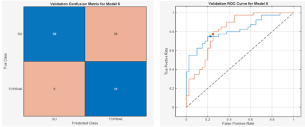
Şekil 4. 23. Kernel Algoritması 2016 Sonrası Yıllardaki Veri Seti Karışıklık Matrisi ve ROC Eğrisi
