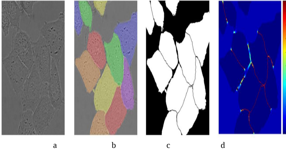
Şekil 3.12 HeLa hücreleri üzerinde UNet yapısı. a) Ham görüntü, b) HeLa hücrelerin farklı renklerde gösterimi, c) UNet tahmini sınıfları, d) Ağı sınır piksellerini öğrenmeye zorlamak için piksel olarak kayıp ağırlığına sahip harita.
