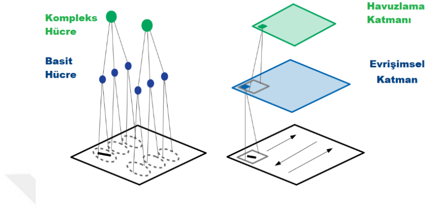
Şekil 3.6 Kedi görme sistemi hücreleri ile ESA katmanlarının karşılaştırılması.
