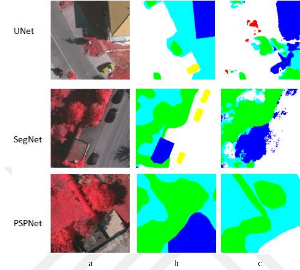
Şekil 6.1 Vaihingen veri seti için, mimarilerde karıştırılan sınıflara ait karşılaştırma. a) Ortofoto görüntü, b) Gerçek zemin görüntüsü, c) Mimari tahmin görüntüsü.
