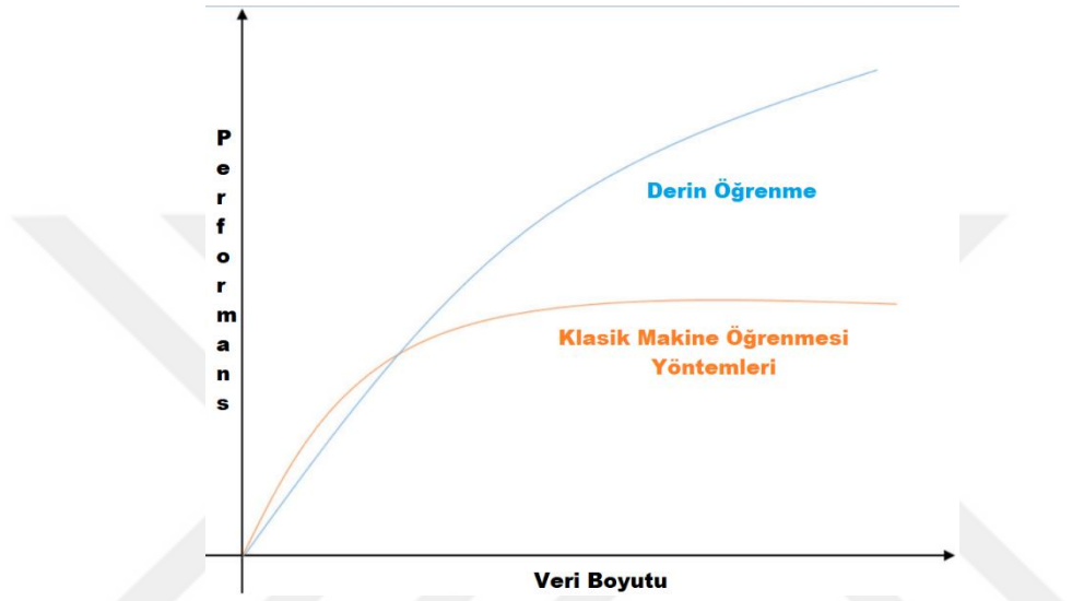
Şekil 3.4 Derin öğrenme ve klasik makine öğrenmesi veri boyutuna göre performansları.
