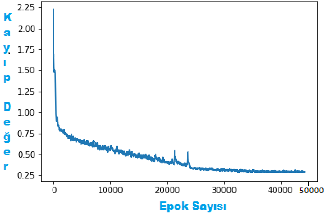
Şekil 5.1 UNet için Vaihingen veri seti kayıp değeri grafiği.
