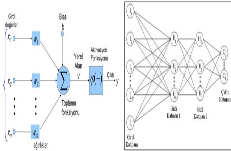
Şekil 3.2 Algılayıcı ve çok katmanlı sinir ağı.
