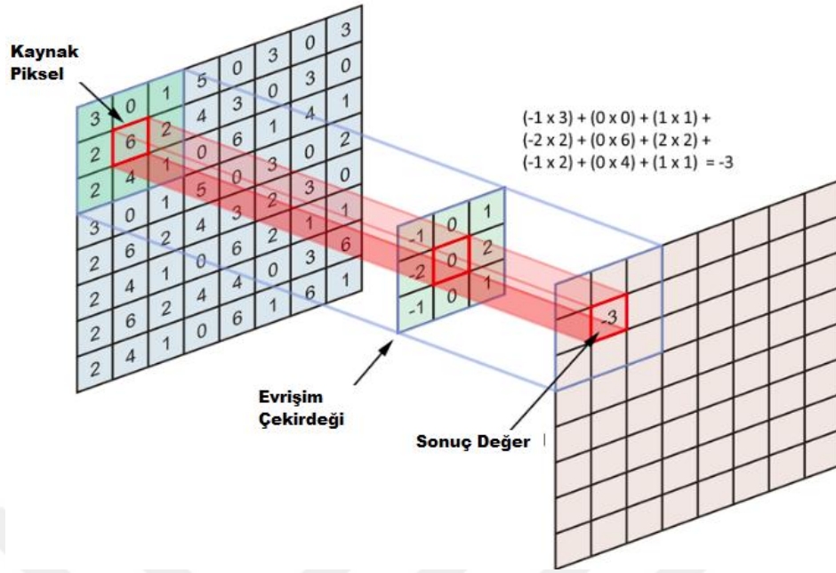
řekil 3.9 Evriřim katmanında yapılan filtreleme işlemlerinin genel bir temsili.
