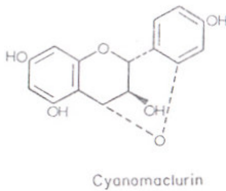
Şekil 4.15 Cyanomaclurin yapısı
