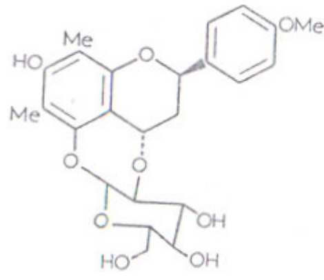
erubin A
