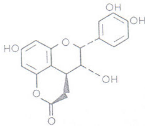
Dryopterin
