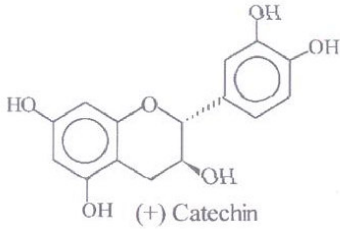
Şekil 4.22 (+)Catechin yapısı
