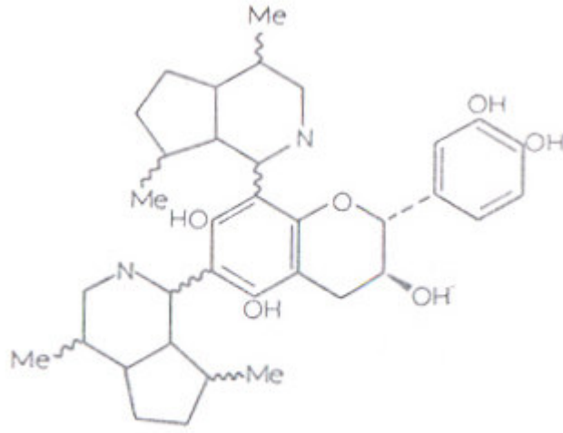
kopsirachin
