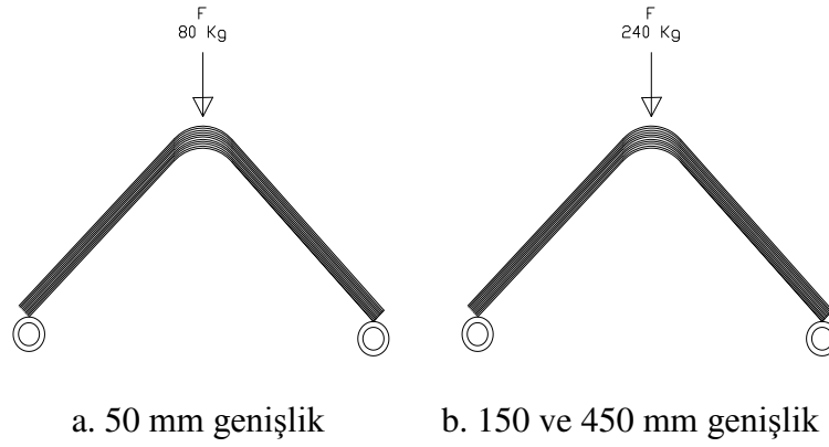
Şekil 3.7. Yorma direnci deneyinde uygulanan yükler
