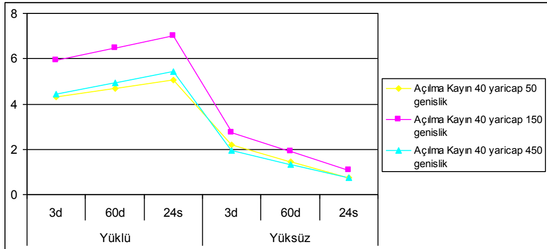
Şekil 4.25. 40 mm yarıçaplı doğu kayınında genişliğe göre açılma miktarları grafiği
