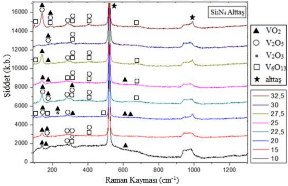
Şekil 3. 36. \text{Si}_3\text{N}_4 alttaş üzerine büyütülen numunelerin Raman spektrumu
