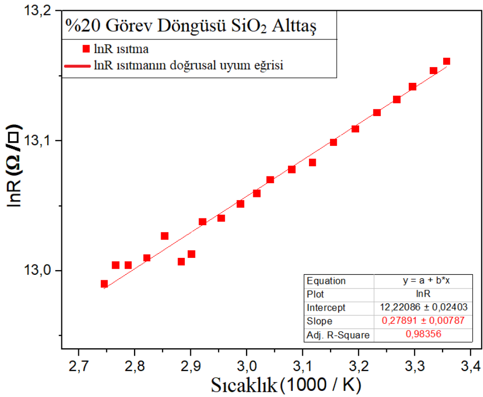
Şekil 3. 7. SiO 2 alttaşı üzerine büyütülen %20 görev döngüsü değerli numune için sıcaklığa bağlı \ln R(1000/T) değişim eğrisi
