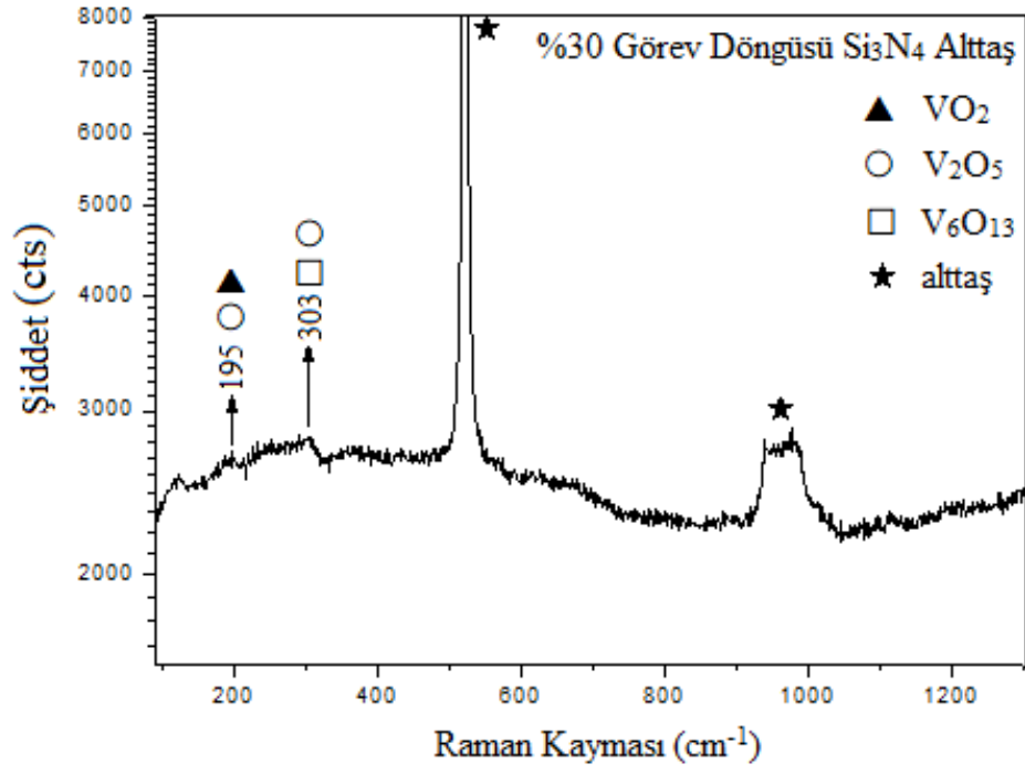
Şekil 3. 32. \text{Si}_3\text{N}_4 alıttaş üzerine büyütülen %30 görev döngüsü değerli numune için Raman spektrumu
