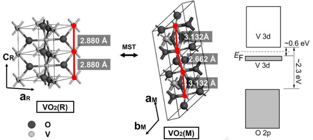
Şekil 1.4. \text{VO}_2(\text{M}) ve \text{VO}_2(\text{R}) 'nin kristalografik yapısı [17] ve \text{VO}_2 kristalinin enerji band sistemi şeması [11]
