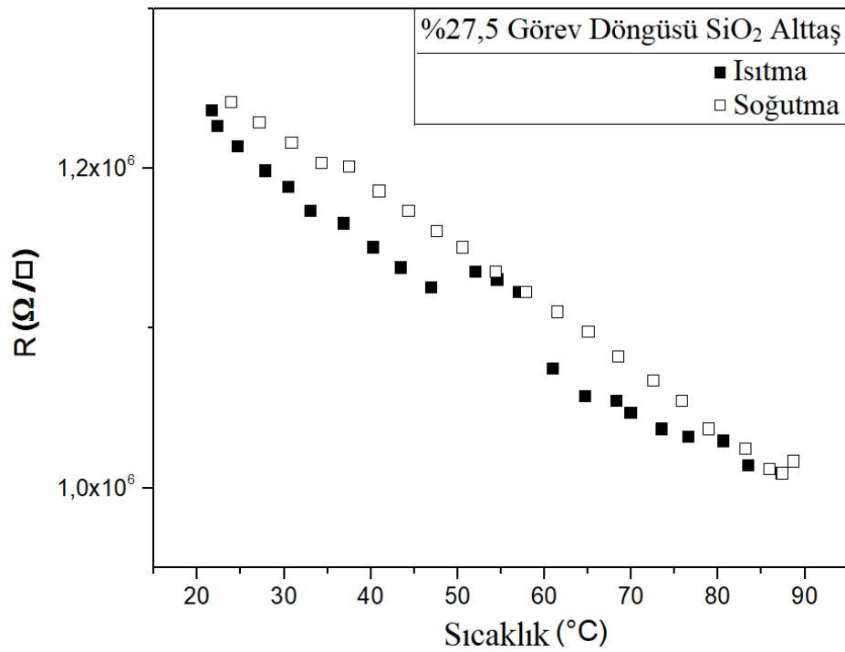
EK – 10. \text{SiO}_2 alttaş üzerine büyütülen %27,5 duty cycle değerli numune için sıcaklığa bağlı R(T) değişim eğrisi [38]
