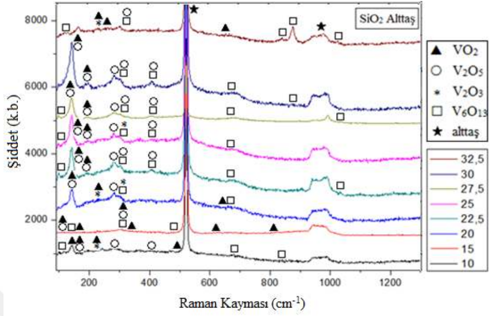
Şekil 3. 35. \text{SiO}_2 alttaş üzerine büyütülen numunelerin Raman spektrumu
