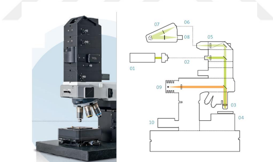
Şekil 2.7. Raman spektroskopisi cihazının kısımları; (1) Uyarıcı lazeri, (2) Optik fiber, (3) Objektif, (4) Tarama kademesi ve / veya motorlu konumlandırma kademesi, (5) Filtre seti, (6) Fotonik fiber, (7) Lens tabanlı UHTS Raman spektrometre serileri, (8) CCD dedektör, (9) Köhler beyaz ışıklı aydınlatma, (10) Odaklama için Z-kademesi [51]
