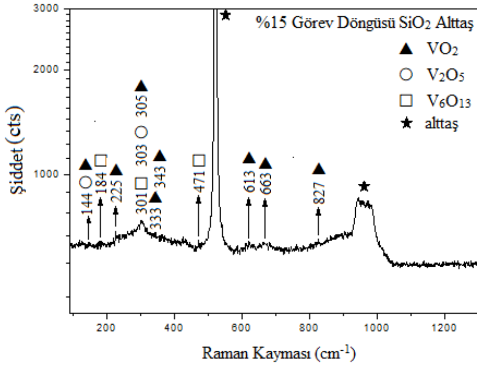
Şekil 3. 21. SiO 2 alttaşı üzerine büyütülen %15 görev döngüsü değerli numune için Raman spektrumu
