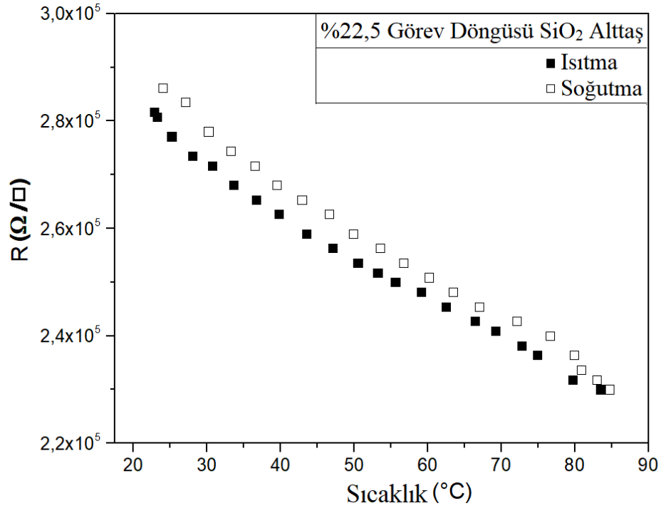
EK – 6. \text{SiO}_2 alttaş üzerine büyütülen %22,5 duty cycle değerli numune için sıcaklığa bağlı R(T) değişim eğrisi [38]
