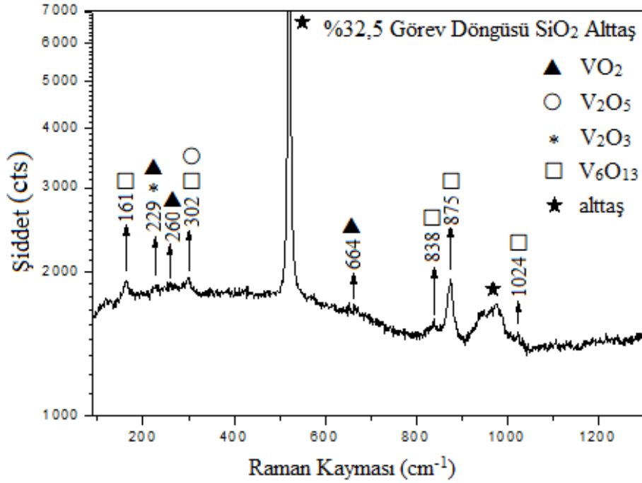
Şekil 3. 33. \text{SiO}_2 alıttaş üzerine büyütülen %32,5 görev döngüsü değerli numune için Raman spektrumu
