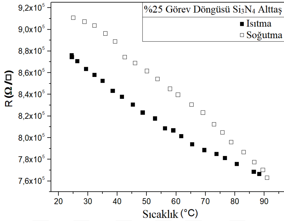
EK – 9. \text{Si}_3\text{N}_4 alttaş üzerine büyütülen %25 duty cycle değerli numune için sıcaklığa bağlı R(T) değişim eğrisi [38]
