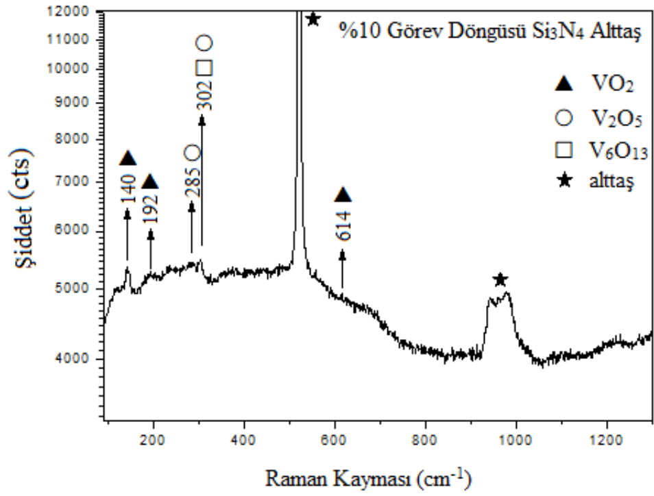
Şekil 3. 20. Si 3 N 4 alttaşı üzerine büyütülen %10 görev döngüsü değerli numune için Raman spektrumu
