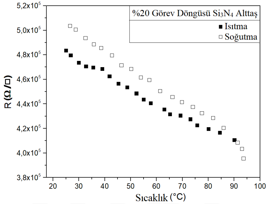
EK – 5. \text{Si}_3\text{N}_4 alttaş üzerine büyütülen %20 duty cycle değerli numune için sıcaklığa bağlı R(T) değişim eğrisi [38]
