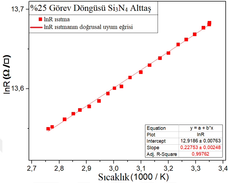
Şekil 3. 12. Si 3 N 4 altaş üzerine büyütülen %25 görev döngüsü değerli numune için sıcaklığa bağlı lnR(1000/T) değişim eğrisi
