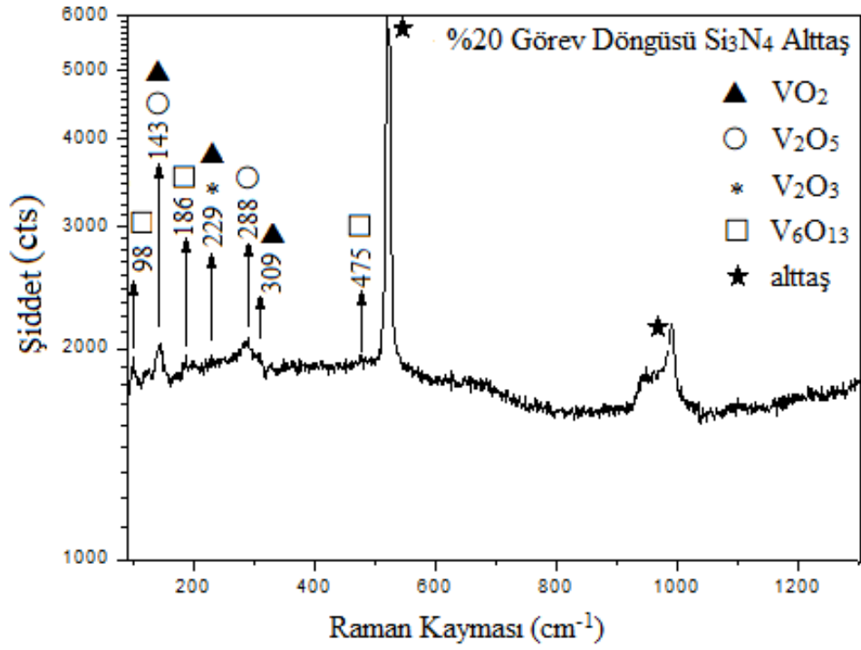
Şekil 3. 24. Si 3 N 4 alttaşı üzerine büyütülen %20 görev döngüsü değerli numune için Raman spektrumu
