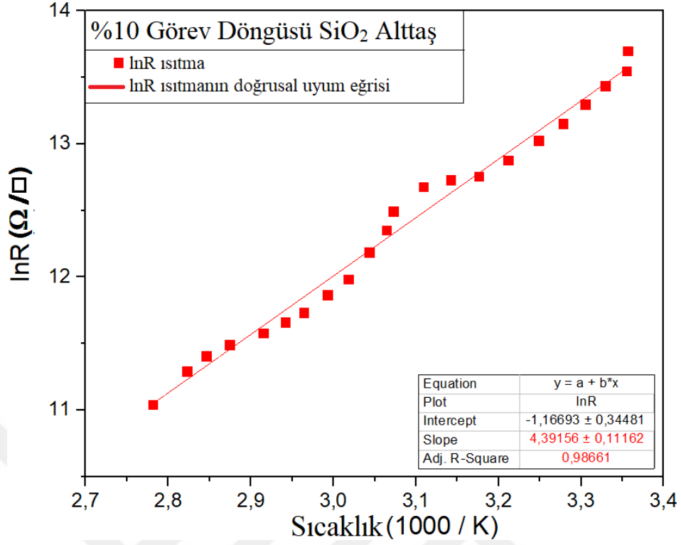
Şekil 3. 4. SiO 2 alttaşı üzerine büyütülen %10 görev döngüsü değerli numune için sıcaklığa bağlı \ln R(1000/T) değişim eğrisi
