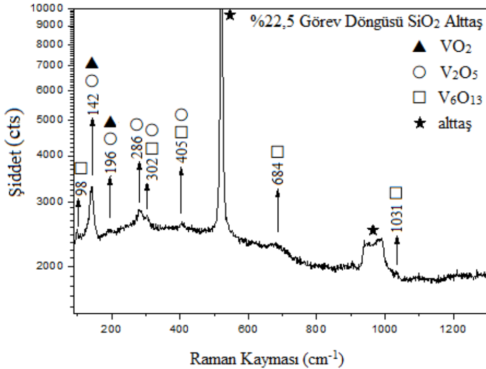
Şekil 3. 25. SiO 2 alttaşı üzerine büyütülen %22,5 görev döngüsü değerli numune için Raman spektrumu
