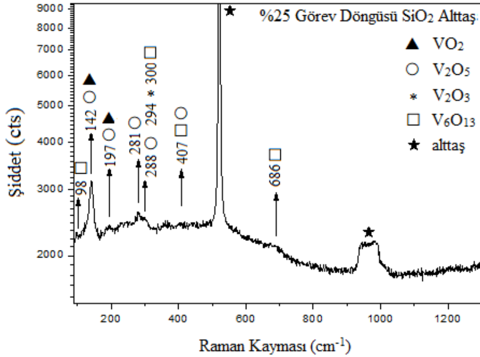
Şekil 3. 27. SiO 2 alttaşı üzerine büyütülen %25 görev döngüsü değerli numune için Raman spektrumu
