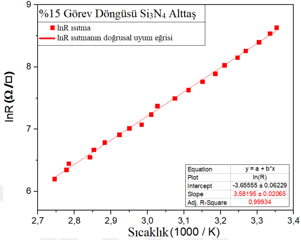
Şekil 3. 6. Si 3 N 4 alttaşı üzerine büyütülen %15 görev döngüsü değerli numune için sıcaklığa bağlı \ln R(1000/T) değişim eğrisi
