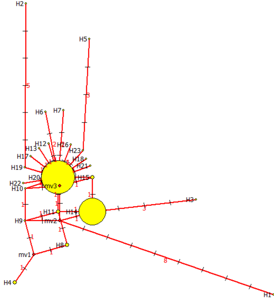
Şekil 4.10. V.destructor 'un mt-COI geninin 423 bp'lık bölgesine göre hazırlanan şebeke analiz sonucu. Dairelerin boyutu, her bir haplotipin frekansı ile orantılıdır. Haplotipleri ayıran mutasyonların sayısı, tire işaretleri ile gösterilmiştir. H: Haplotip
