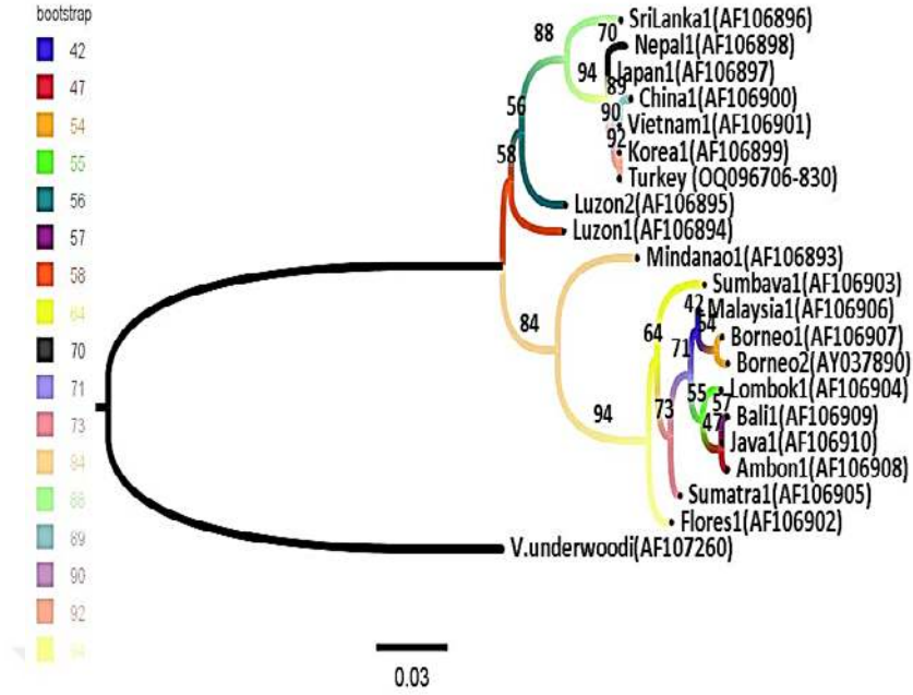
Şekil 4.8. V.destructor ve V.jacobsoni 'nin farklı haplogrupları ile Akdeniz Bölgesi izolatlarının [Turkey (OQ096706-830)] filogenetik ilişkilerini gösteren ağaç. Ağaç mt-COI geninin kısmi dizilerine (477 bp) göre Maximum Likelihood yöntemi ile hazırlanmış ve taksonların GenBank erişim numaraları parantez içerisinde belirtilmiştir. V.underwoodi dış grup olarak kullanılmıştır. Dallar bootstrap (5000 döngü) değerlerine göre renklendirilmiştir.
