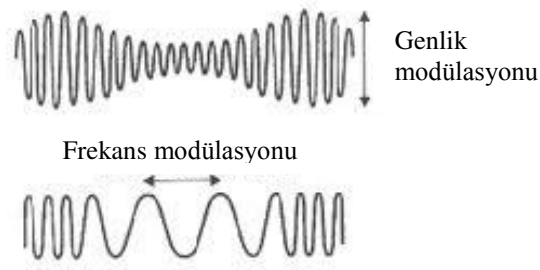
Şekil 4. Elektro manyetik bir dalganın değiştirilme (modülasyon) teknikleri
