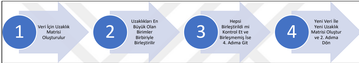
Şekil 3.6. Tam Bağıntı Kümeleme Yöntemi Algoritması
