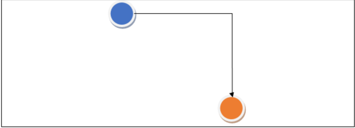
Şekil 3.2. Manhattan ( City – Block ) Uzaklık Ölçütü Şema Çizimi
