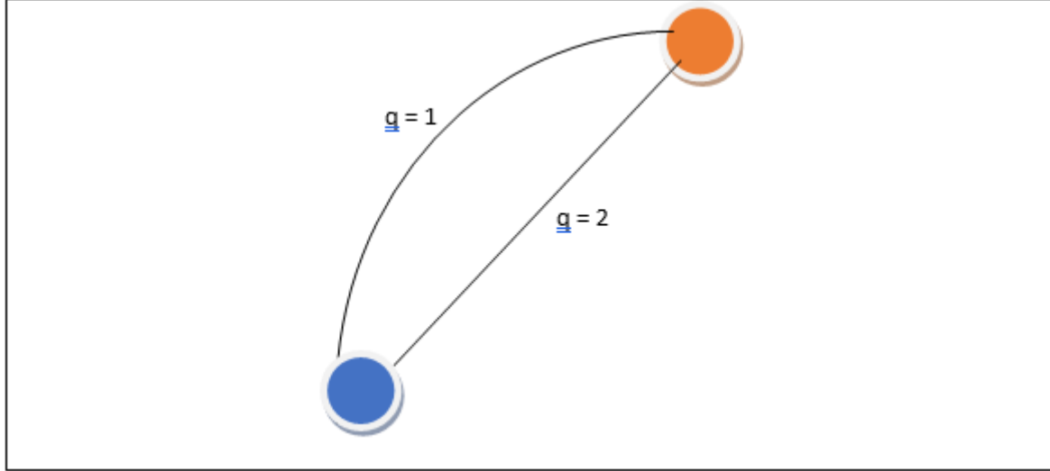
Şekil 3.1. Minkowski Uzaklık Ölçütü Şema Çizimi
