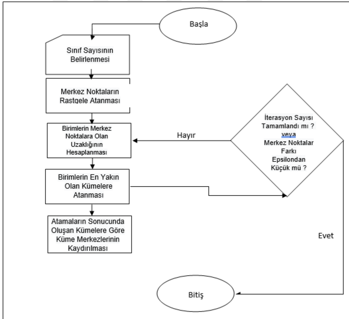
Şekil 3.8. K – Ortalamalar Kümeleme Yöntemi Algoritması
