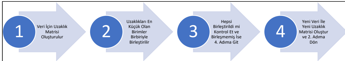
Şekil 3.5. Tek Bağıntı Kümeleme Yöntemi Algoritması
