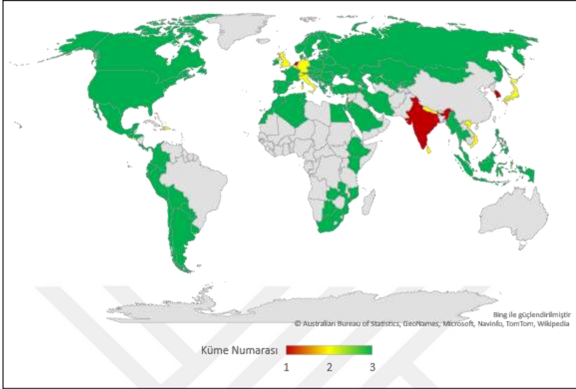
Şekil 5.4. Merkez Bağntı Kümeleme Yöntemi Sonucunun Haritada Gösterimi
