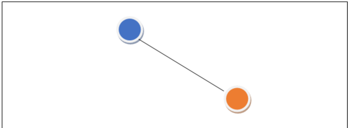
Şekil 3.3. Öklid Uzaklık Ölçütü Şema Çizimi
