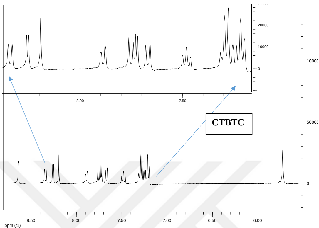
Figure A.5. ^1\text{H} NMR CTBTC monomer
