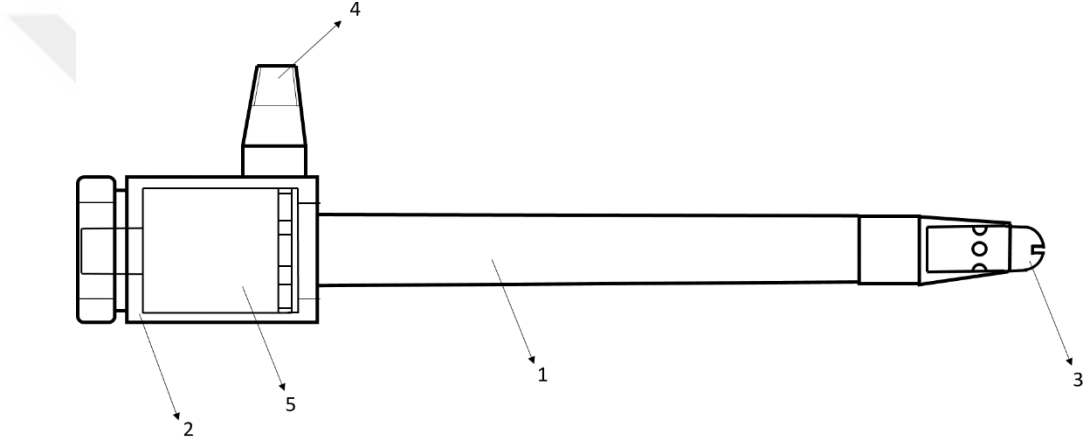
Şekil 4.1. Ana tüp .1) sıcak kanal. 2) soğuk kanal. 3) kontrol valfi. 4) Basınç hava girişi. 5) Generetör.
