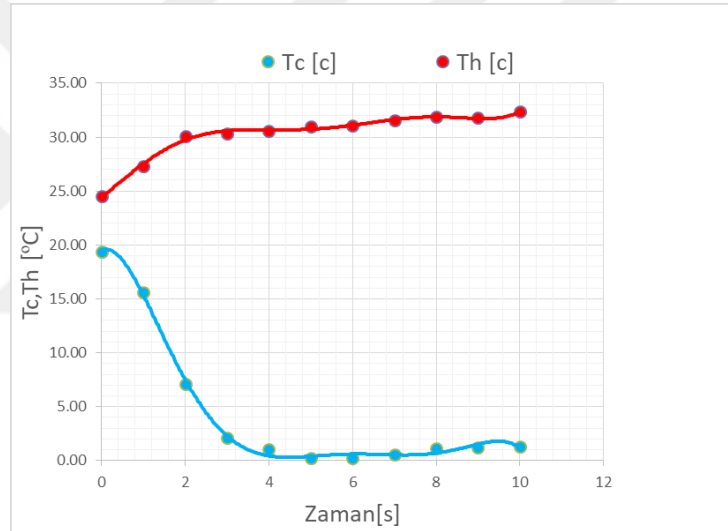
řekil 4.22.        vorteks t p nde meydana gelen soğuk ve sıcak hava sıcaklıklarının zamana g re deęiřimi
