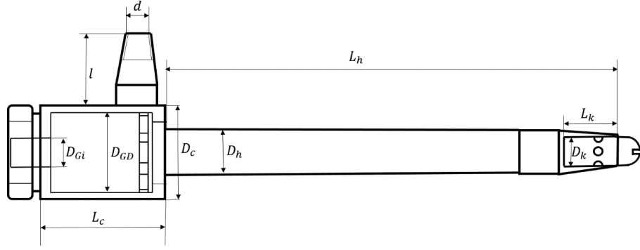
Şekil 4.7. Vorteks tüpün geometrik parametrelerinin sembolleriyle
