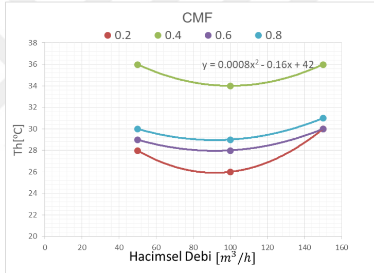
Şekil 4.24. Vorteks tüpünün CMF çeşitli değerlerinde basınçlı hava debinin değişmesiyle sıcak hava sıcaklık derecesinin değişmesi etkisi
