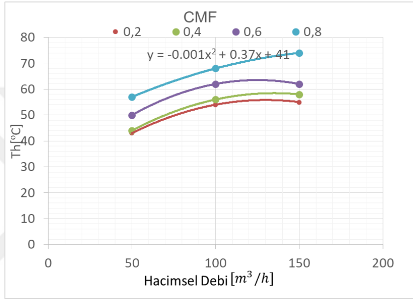
 ekil 4.18. Vorteks t p n n CMF  e itli deęerlerinde basın lı hava debinin deęi mesiyle sıcak hava sıcaklık derecesinin deęi mesie etkisi
