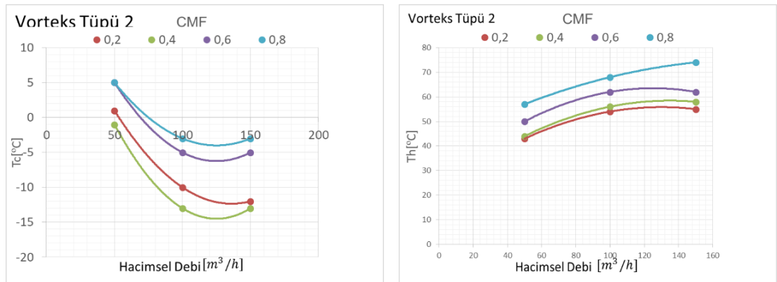
řekil 4.27. 1. ve 2. vortex t plerinde ve x air’da soğuk ve sıcak havanın sıcaklık derecesinin deđiřmesi ile zaman arasındaki iliřkinin karřılařtırılması
