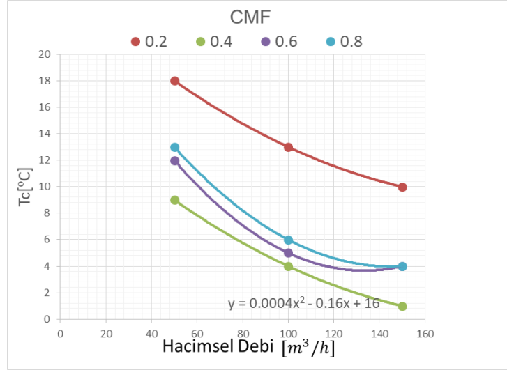
Şekil 4.23. Vorteks tüpünün CMF çeşitli değerlerinde basınçlı hava debinin değişmesiyle soğuk hava sıcaklık derecesinin değişmesi etkisi
