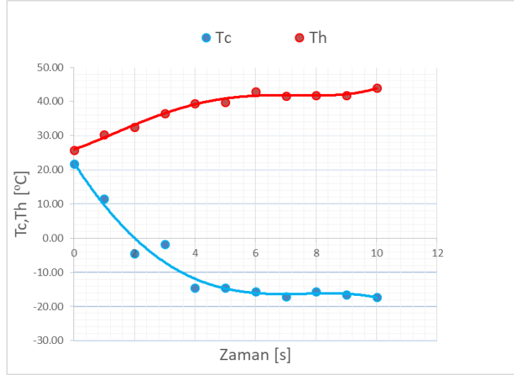
Şekil 4.16. Birinci vorteks tüpünde meydana gelen soğuk ve sıcak hava sıcaklıklarının zamana göre değişimi
