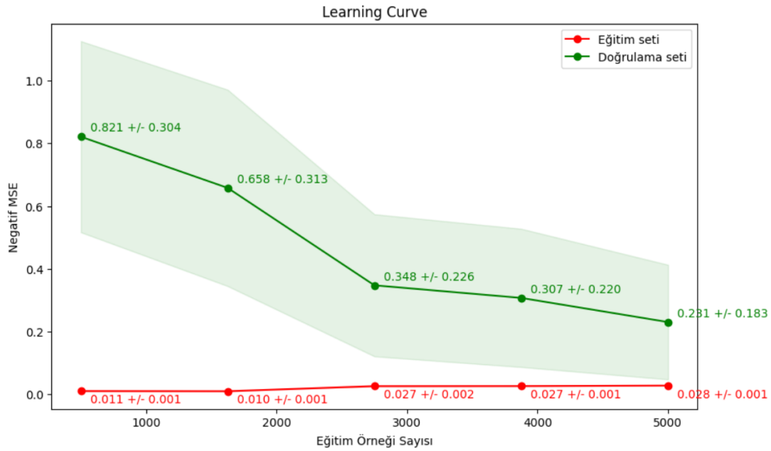
Şekil 4.5. GBR Learning Curve grafiği (Veri seti 1)
