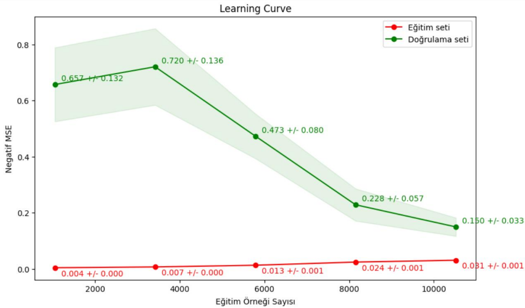
Şekil 4.6. GBR Learning Curve grafiği (Veri seti 2)
