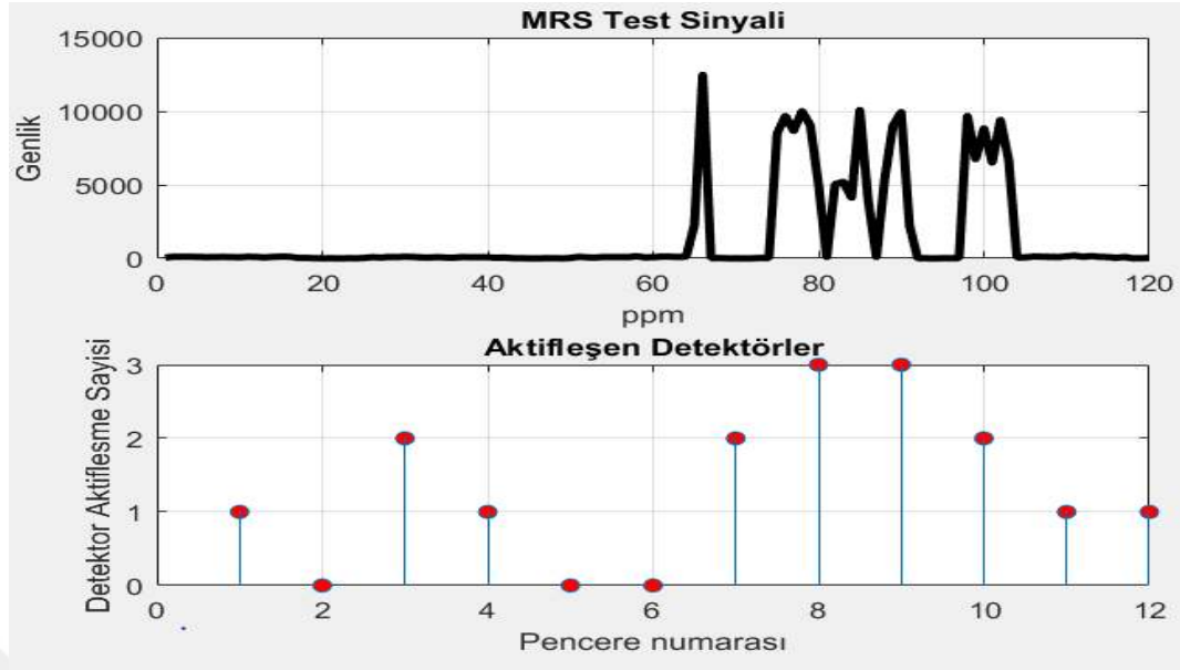
Şekil 4.23. Deneysel Çalışma 7 için anormal web verilerinin bulunduğu sinyalde aktifleştiren detektörler (22. Sinyal örüntüsü)
