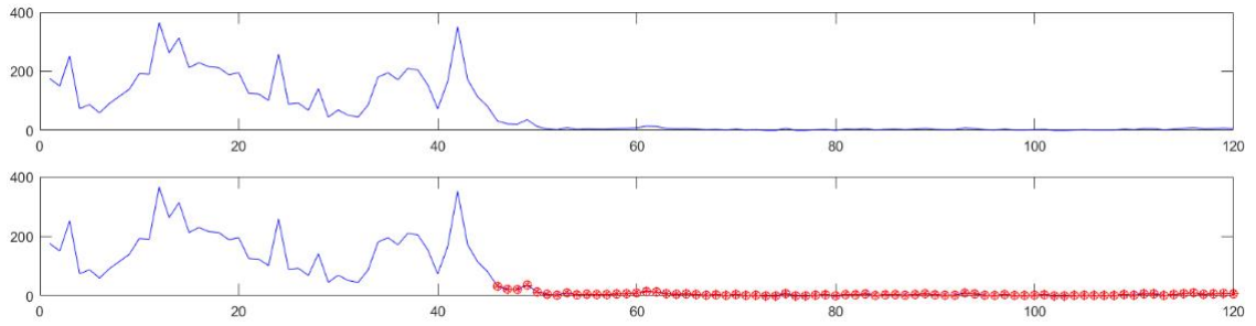
Şekil 4.18. Deneyisel Çalışma 6 için 40. sinyal üzerinde anormal web trafik verisinin bulunduğu sinyal örüntüsü (P10)
