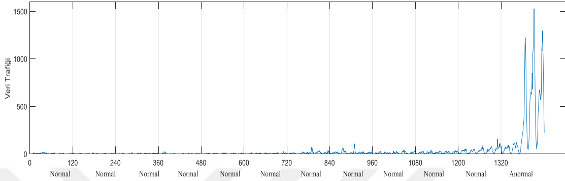
Şekil 3.3. Web trafik verilerin pencerelere bölünmesi
