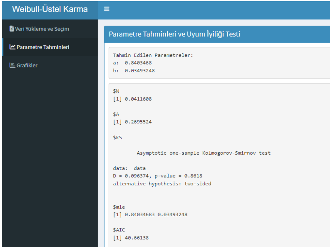
Şekil 5.2: Uygulamanın parametre tahmin paneli
