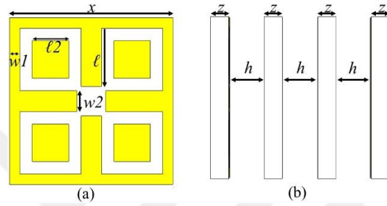
Şekil 3.8. Tasarım 3 Birim Hücre Geometrisi (a) Ön Görünüm (b) Yan Görünüm
