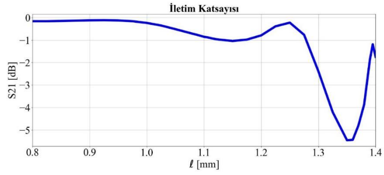
Şekil 3.9. Tasarım 3 Birim Hücresinin 28 GHz'deki İletim Katsayısı
