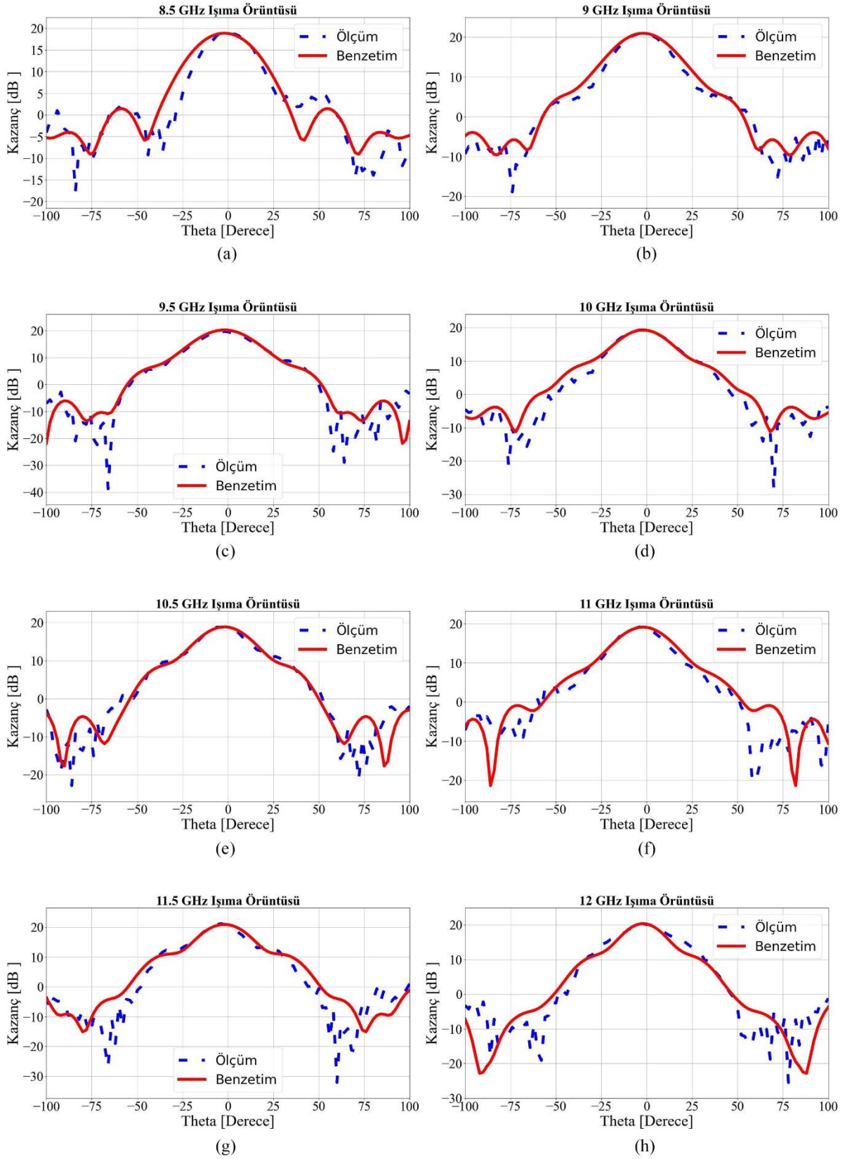
Şekil 5.4. Tasarım 1 İDA'ya ait E-Düzlemi Işıma Örüntüsü Benzetim ve Ölçüm Sonuçları (a) 8,5 GHz (b) 9 GHz (c) 9,5 GHz (d) 10 GHz (e) 10,5 GHz (f) 11 GHz (g) 11,5 GHz (h) 12 GHz
