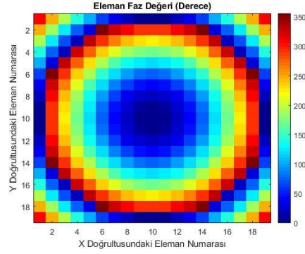
Şekil 4.12. Tasarım 3 İDA Eleman Faz Dağılımı
