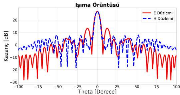
Şekil 4.9. Tasarım 2 İDA için 10 GHz E ve H Düzlemi Işınma Örüntüsü
