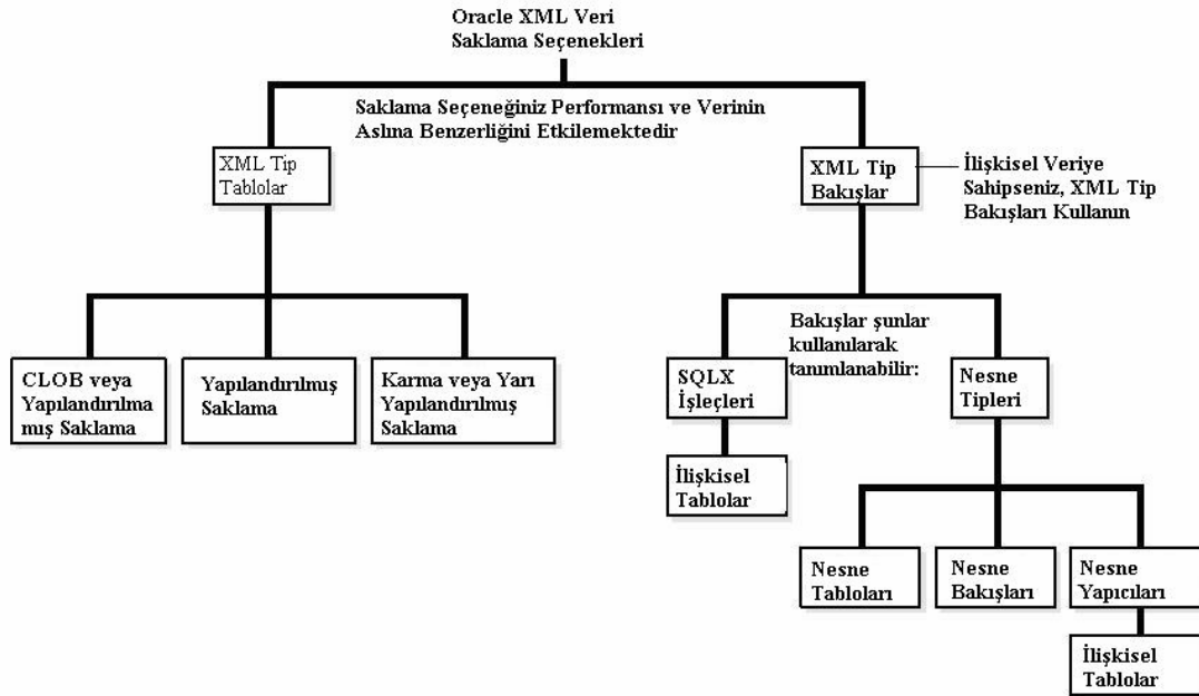
Şekil 3.10: Yapılandırılmış Saklama Seçenekleri [25]
