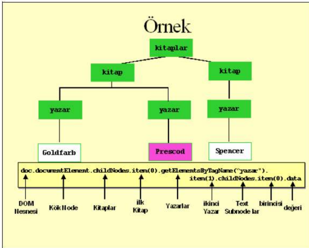
Şekil 2.1: Örnek XML Belgesi.
