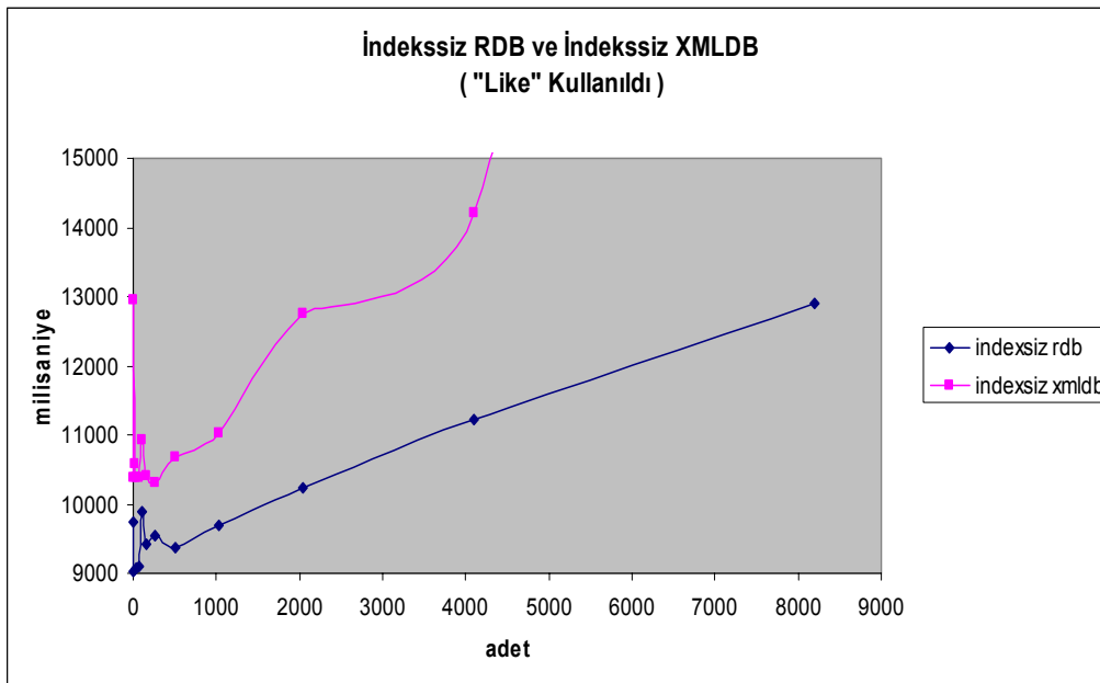
Şekil 4.9: Metin ve XML Belgeleri için Dizinleme Kullanılmadan Yapılan Sorgulama Yukarıdaki şekilde yatay eksen dosya sayısı, dikey eksen ise sorgulama sonucu milisaniye olarak gösterilmiştir. Bununla birlikte mavi eğri dizinleme
