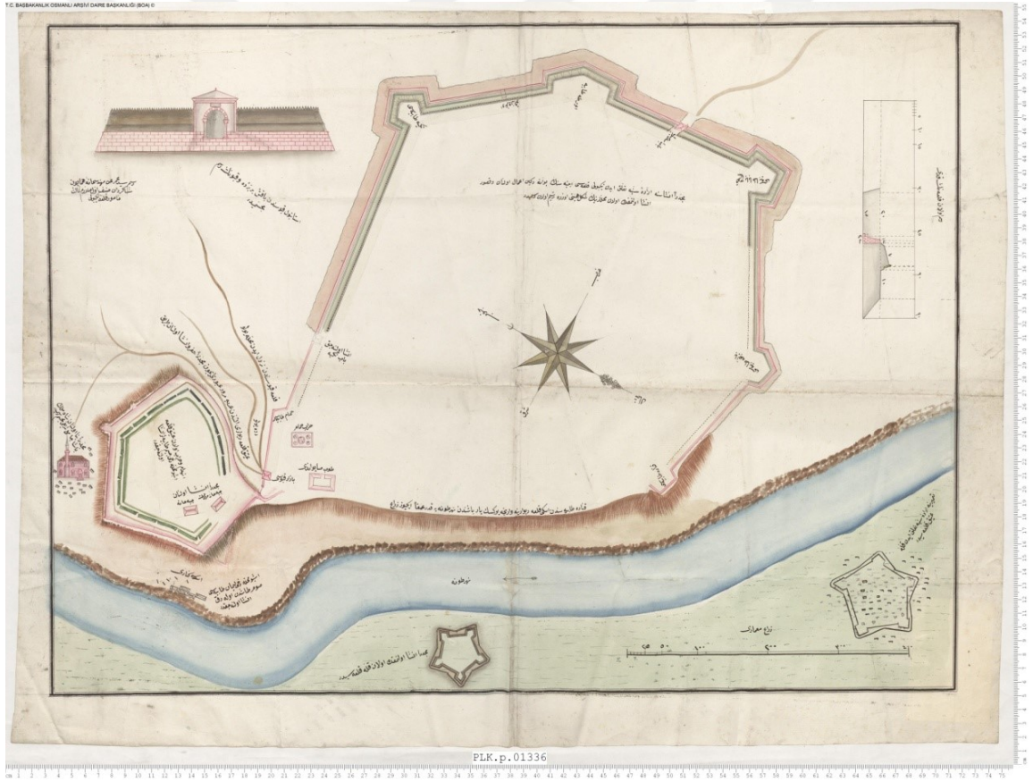
Şekil 2: Niğbolu Kalesi Planı 87
