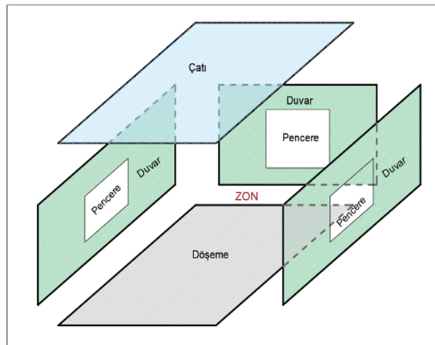
Şekil 15. Isıl denge denklemlerinin tek bölge yapı modelinde yazıldığı yapı elemanlarının şematik gösterimi.
