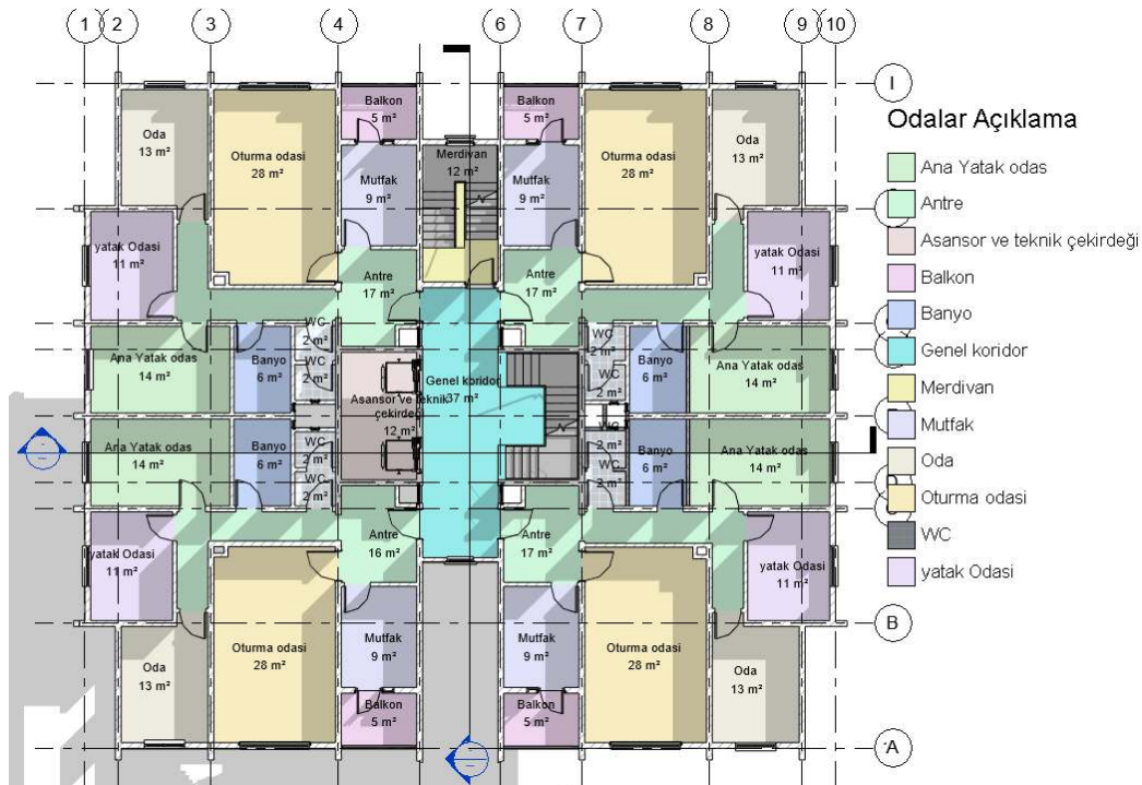
Şekil 23. Daireli TOKİ C tipi konut projesi, Tipik kat planı.
