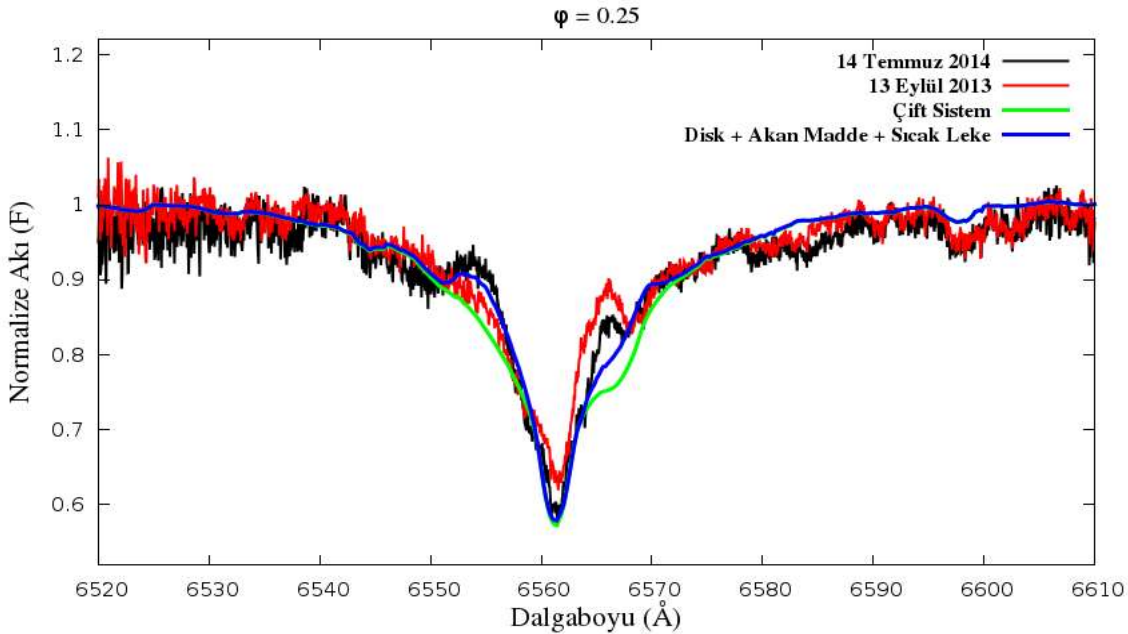
Şekil 4.8. U Sge sisteminin farklı zamanlarda aynı evrede alınmış H_\alpha tayflarında çevresel maddenin değişkenlik göstermesi
