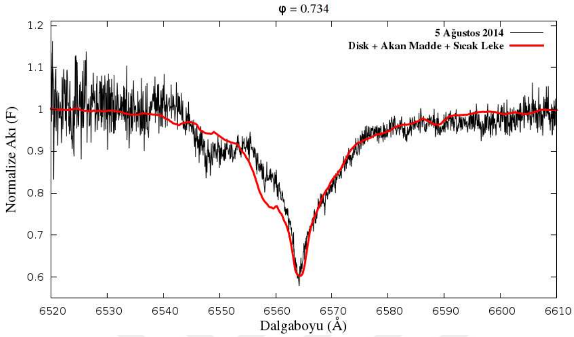
Şekil 4.12. i) U Sge sisteminin \phi = 0.734 evrede gözlenen H_\alpha çizgisi (siyah) ve bu çizgiye yapılan SHELLSPEC modeli (kırmızı)
