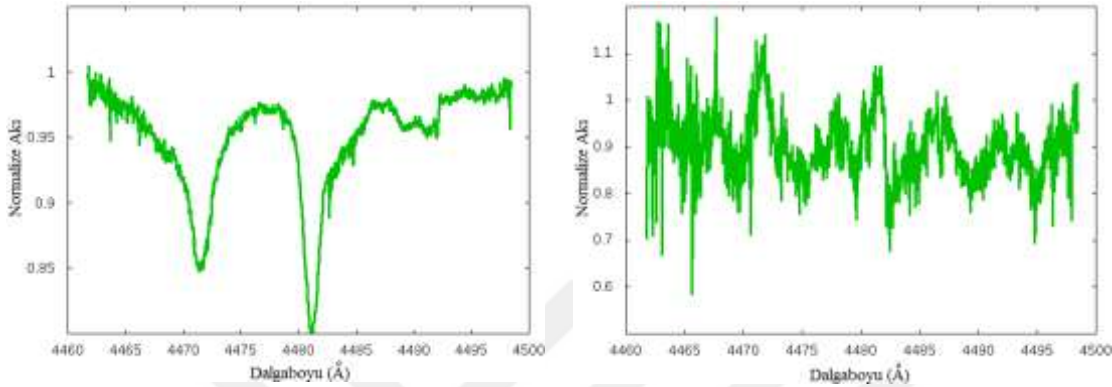
Şekil 4.5. U Sge sistemindeki baş bileşenin (sol) ve yoldaş bileşenin (sağ) ayırıştırılmış tayfları
