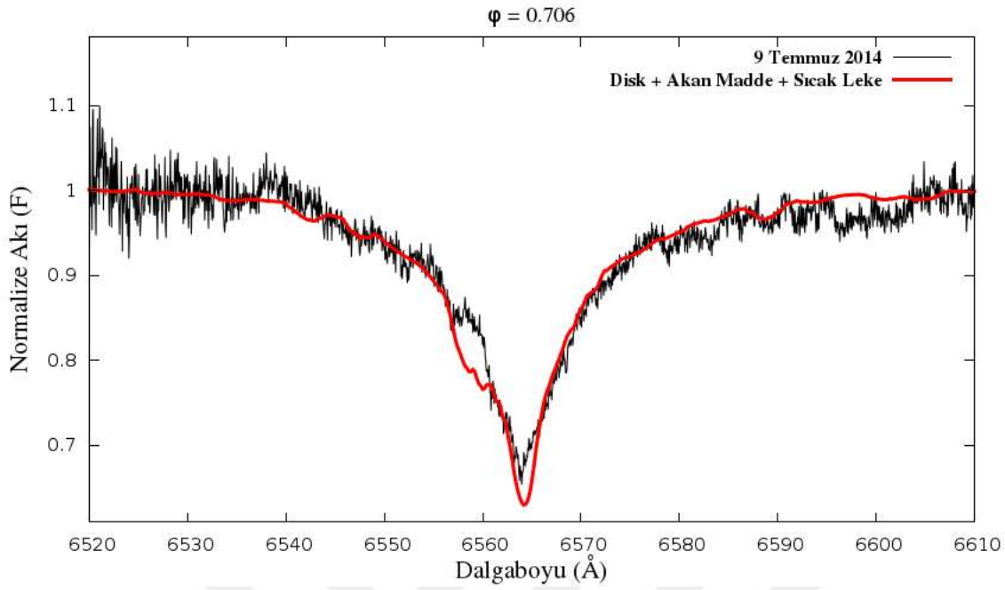
Şekil 4.12. e) U Sge sisteminin \phi = 0.706 evrede gözlenen H_\alpha çizgisi (siyah) ve bu çizgiye yapılan SHELLSPEC modeli (kırmızı)
