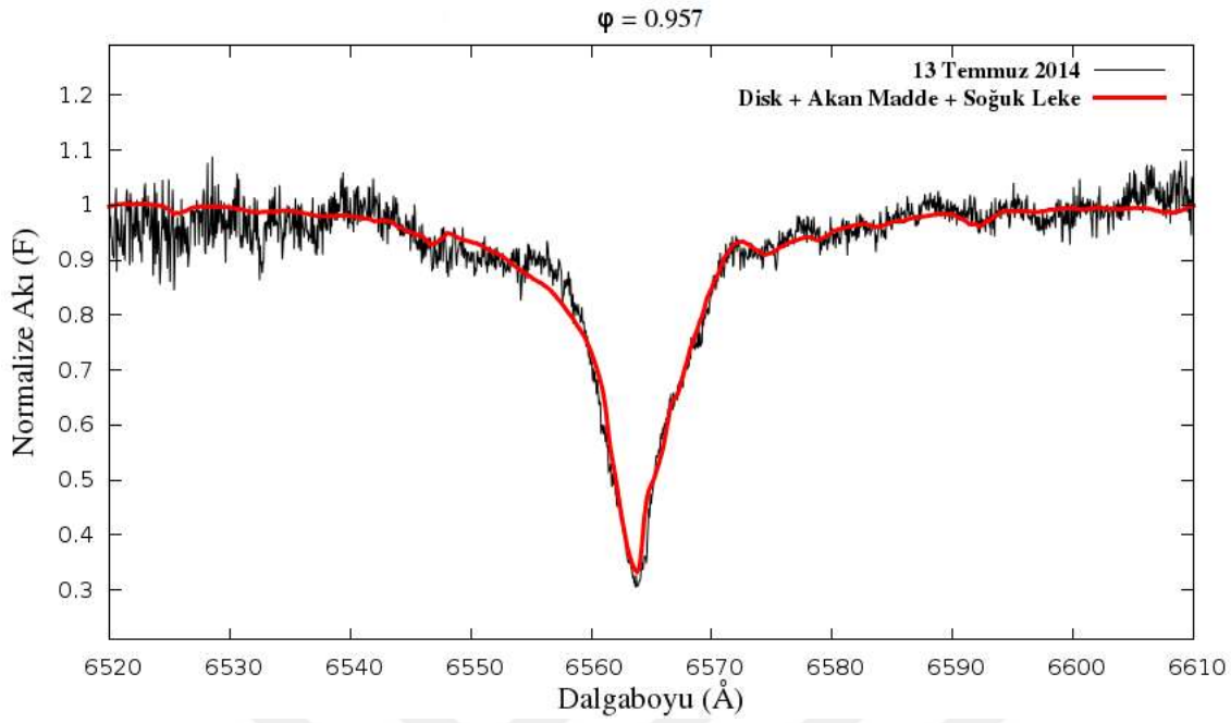
Şekil 4.12. s) U Sge sisteminin \phi = 0.957 evrede gözlenen H_\alpha çizgisi (siyah) ve bu çizgiye yapılan SHELLSPEC modeli (kırmızı)
