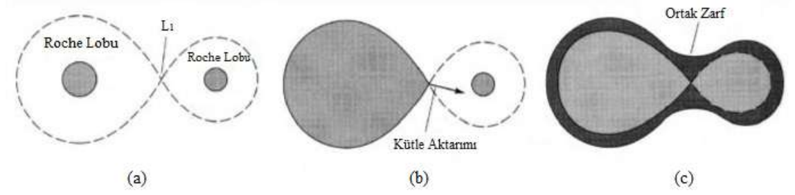
Şekil 2.4. a) Ayırık çift sistem. b) Yarı-ayırık çift sistem. c) Değen çift sistem (Zeilik ve Gregory 1998)
