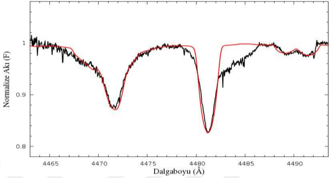
Şekil 4.6. U Sge sisteminin baş bileşenine ait ayrıştırılmış tayfının (siyah) He I (4471.48 Å) ve Mg II (4481.33 Å) çizgilerine yapılan sentetik tayf modeli (kırmızı)
