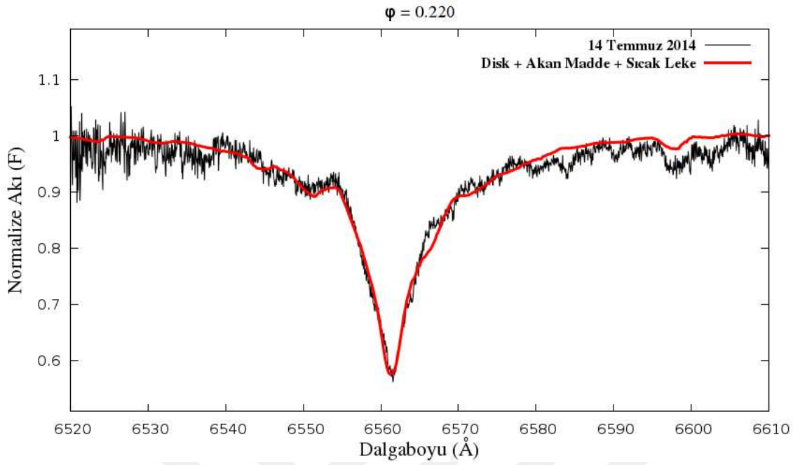
Şekil 4.11. ı) U Sge sisteminin \phi = 0.220 evrede gözlenen H_\alpha çizgisi (siyah) ve bu çizgiye yapılan SHELLSPEC modeli (kırmızı)
