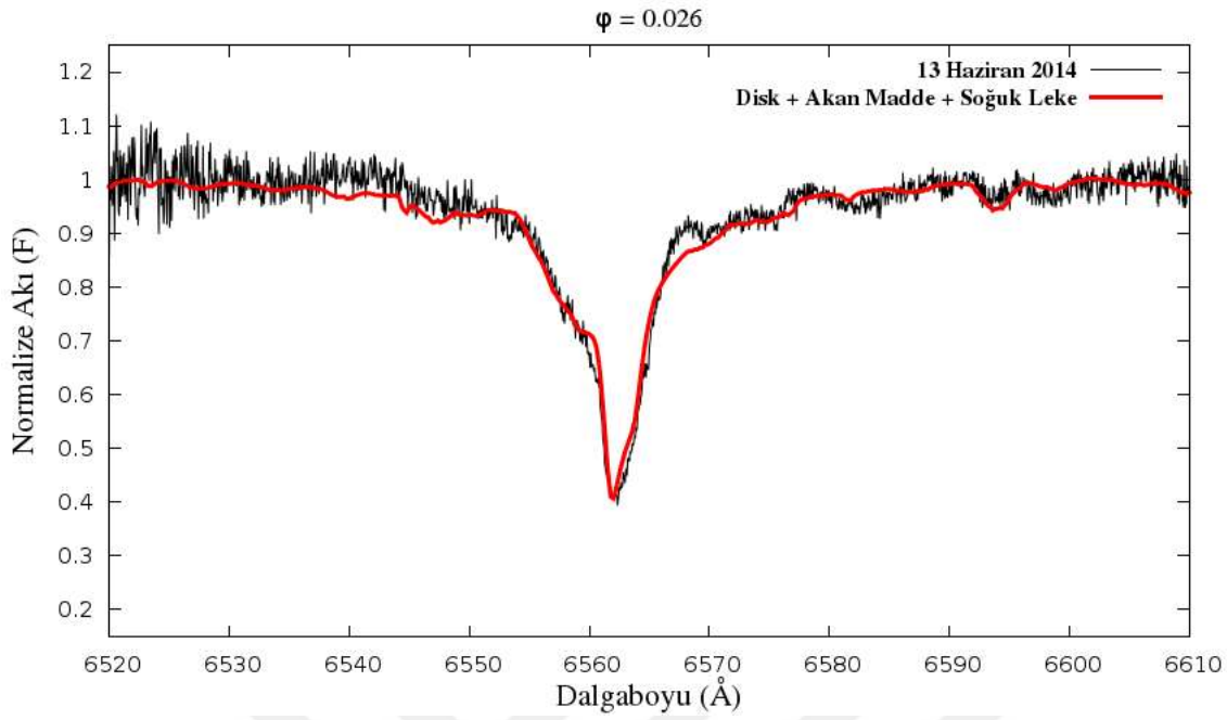
Şekil 4.11. b) U Sge sisteminin \phi = 0.026 evrede gözlenen H_\alpha çizgisi (siyah) ve bu çizgiye yapılan SHELLSPEC modeli (kırmızı)
