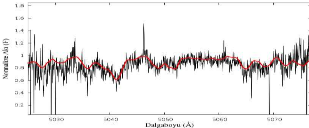
Şekil 4.1. a) Baş bileşenin tamamen örtüldüğü evrede (birinci minimum ortası) 41. échelle dizisi için üretilen sentetik yoldaş bileşen tayfı (kırmızı) ve gözlenen tayf (siyah)
