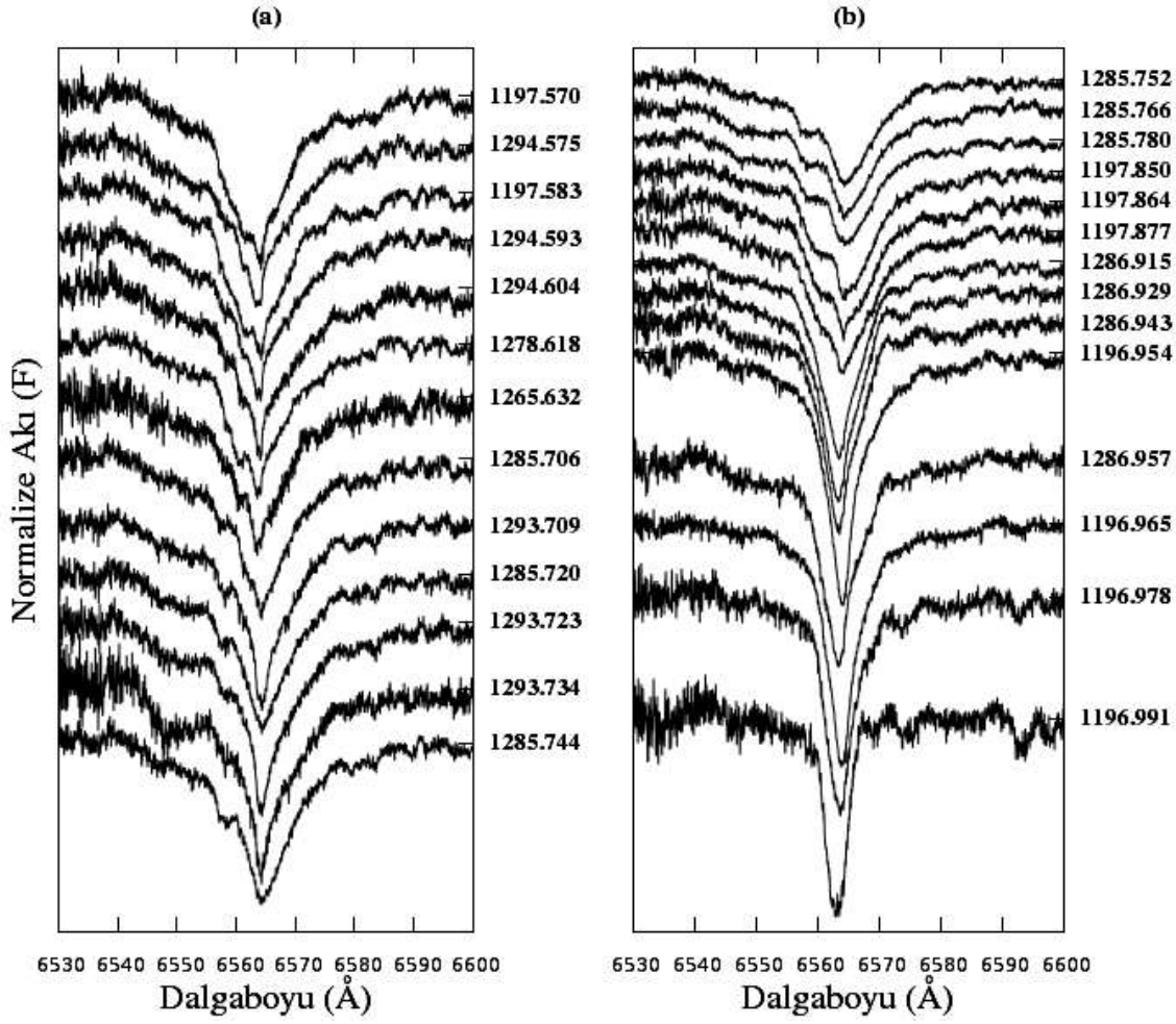
Şekil 3.2. U Sge sisteminin gözlenen tayflarındaki H \alpha çizgisini içeren tayf bölgesinin a) \phi = 0.56 - 0.75 evre aralıklarında b) \phi = 0.75 - 1.00 evre aralıklarında evreye göre sıralanmış tayfları
