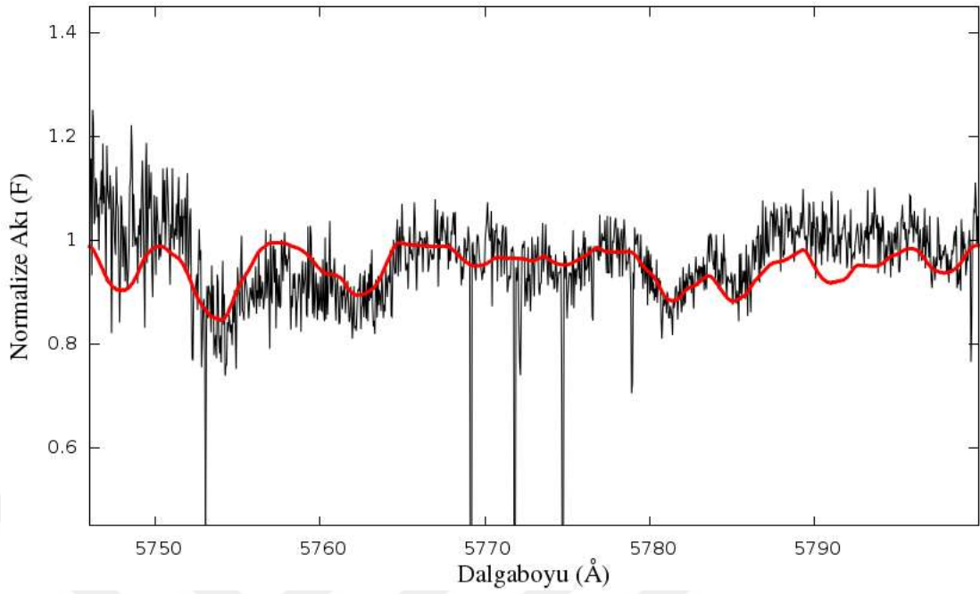
Şekil 4.1. 1) Baş bileşenin tamamen örtüldüğü evrede (birinci minimum ortası) 29. échelle dizisi için üretilen sentetik yoldaş bileşen tayfı (kırmızı) ve gözlenen tayf (siyah)
