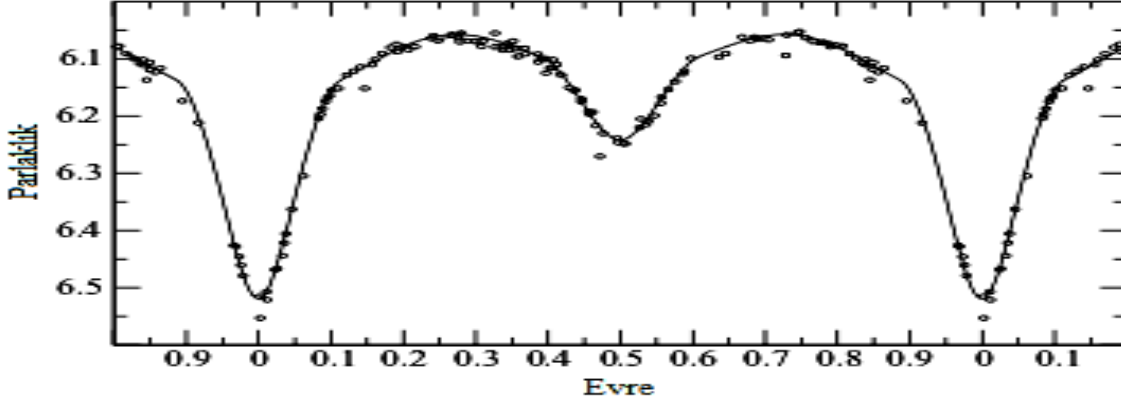
Şekil 2.6. \beta Lyr türü bir çift sistem olan V716 Cen'in ışık eğrisi (Bakış vd 2008)
