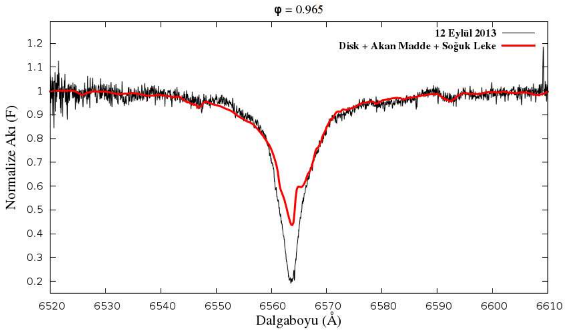
Şekil 4.12. t) U Sge sisteminin \phi = 0.965 evrede gözlenen H_\alpha çizgisi (siyah) ve bu çizgiye yapılan SHELLSPEC modeli (kırmızı)
