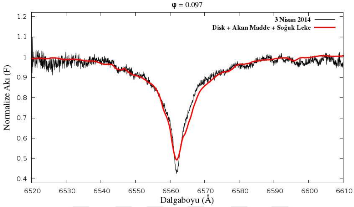
Şekil 4.11. e) U Sge sisteminin \phi = 0.097 evrede gözlenen H_\alpha çizgisi (siyah) ve bu çizgiye yapılan SHELLSPEC modeli (kırmızı)
