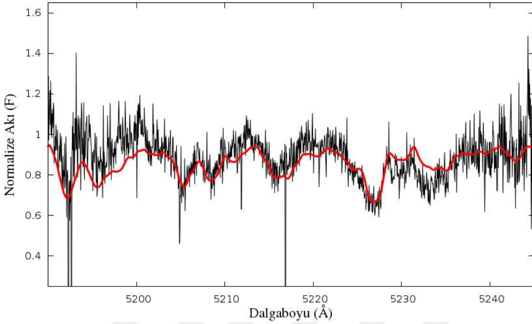
Şekil 4.1. c) Baş bileşenin tamamen örtüldüğü evrede (birinci minimum ortası) 38. échelle dizisi için üretilen sentetik yoldaş bileşen tayfı (kırmızı) ve gözlenen tayf (siyah)
