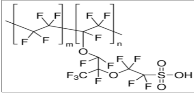
Şekil 2.4. Nafion'un moleküler yapısı
