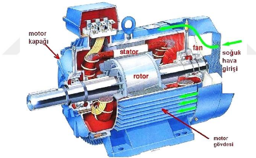
Şekil 3. 5: Alternatif Akım Motoru
