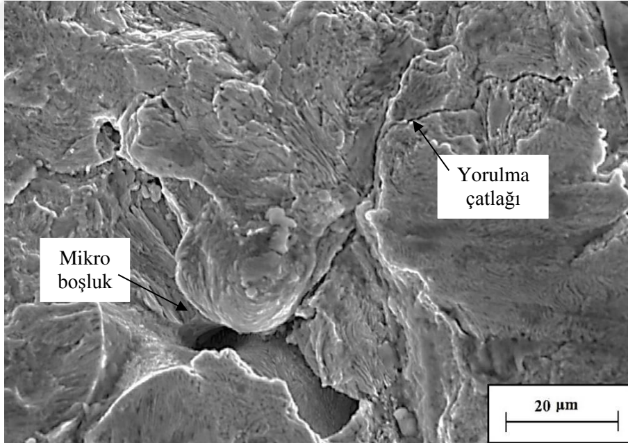
Şekil 24. 119 MPa gerilme değeriinde yorulma deneyine tabi tutulan, dökülmüş durumdaki Zn-27Al-1Cu alaşıma ait numunenin kırılma yüzeyinin detayını gösteren SEM fotoğrafı
