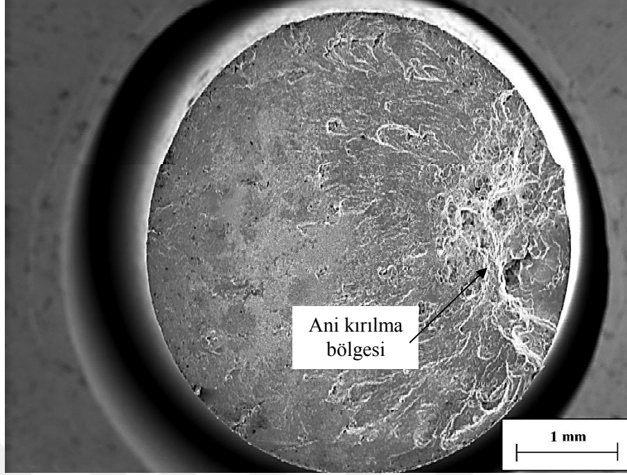
Şekil 25. 174 MPa gerilme değeriinde yorulma deneyine tabi tutulan, 0,5 saat yaşlandırılmış durumdaki Zn-27Al-1Cu alaşıma ait numunenin kırılma yüzeyini gösteren
