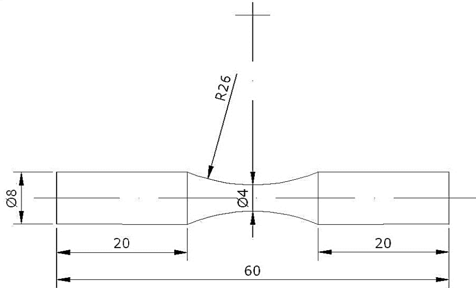
Şekil 6. Yorulma deney numunesinin şekli ve boyutları
