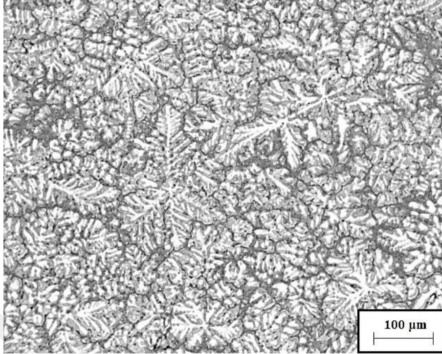
Şekil 7. Zn-27Al-1Cu alaşımlarının dökülmüş durumdaki içyapısı
