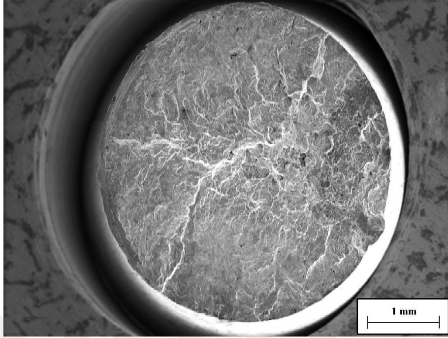
Şekil 21. 146 MPa gerilme değeriinde yorulma deneyine tabi tutulan, dökülmüş durumdaki Zn-27Al-1Cu alaşımina ait numunenin kırılma yüzeyini gösteren SEM fotoğrafı
