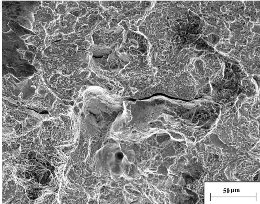
Şekil 26. 174 MPa gerilme değeriinde yorulma deneyine tabi tutulan, 0,5 saat yaşlandırılmış durumdaki Zn-27Al-1Cu alaşıma ait numunenin kırılma yüzeyinin detayını gösteren SEM fotoğrafı
