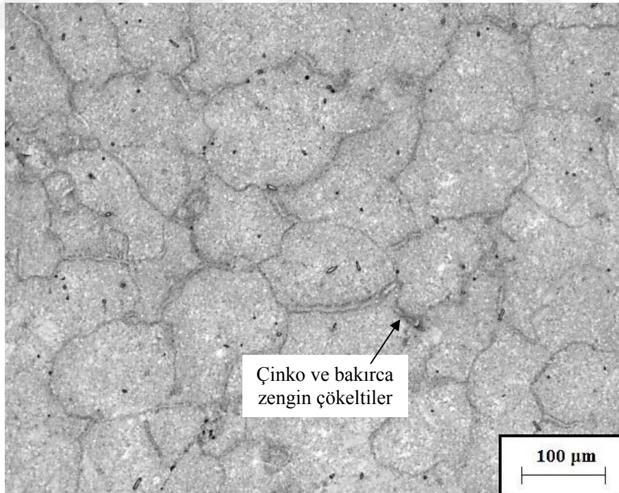
Şekil 10. 100 °C sıcaklıkta 1 saat yaşılandırılan Zn-27Al-1Cu alaşımasının içyapısı
