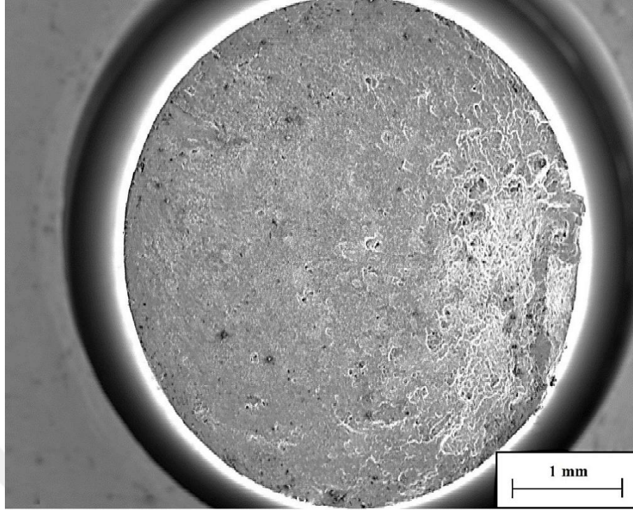
Şekil 27. 160 MPa gerilme değeriinde yorulma deneyine tabi tutulan, 1 saat yaşılandırılmış durumdaki Zn-27Al-1Cu alaşıma ait numunenin kırılma yüzeyini gösteren SEM fotoğrafı
