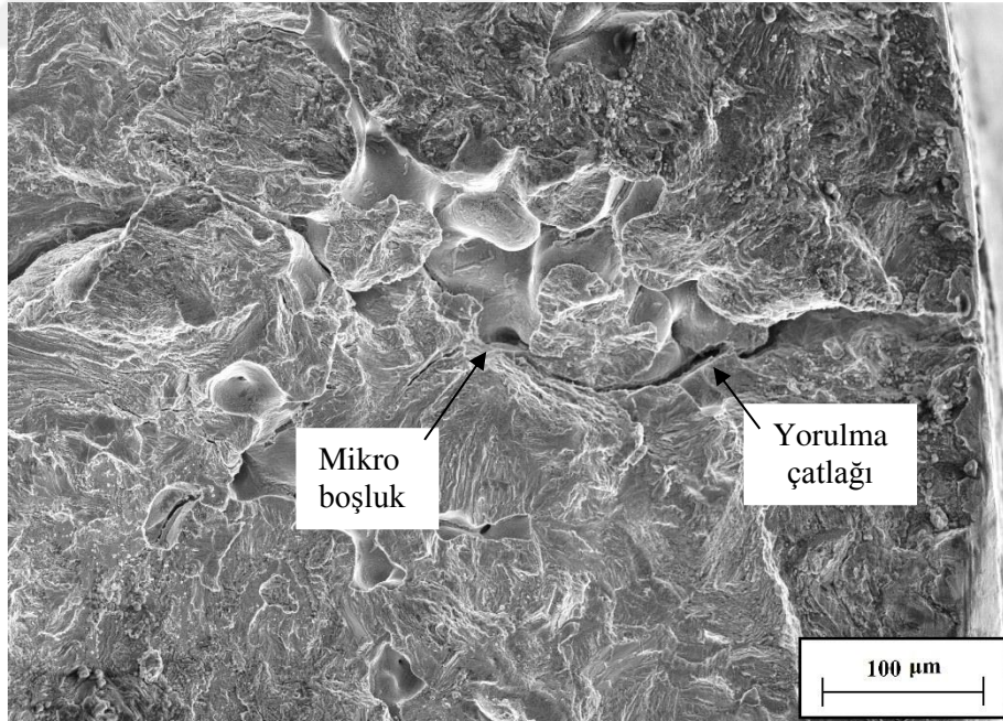
Şekil 22. 146 MPa gerilme değeriinde yorulma deneyine tabi tutulan, dökülmüş durumdaki Zn-27Al-1Cu alaşımina ait numunenin kırılma yüzeyinin detayını gösteren SEM fotoğrafı
