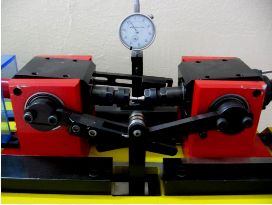
Şekil 5. Deney örneğinin kırılması durumunda açısal hareket serbestliğine sahip yatakların genel görünümü
