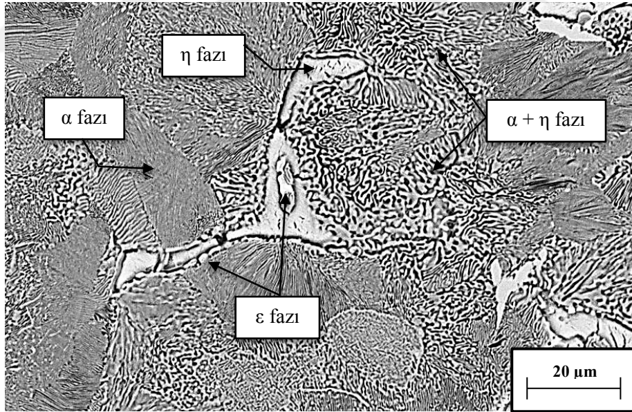
Şekil 8. Zn-27Al-1Cu alaşımlarının dökülmüş durumdaki içyapısının detayını gösteren SEM fotoğrafı
