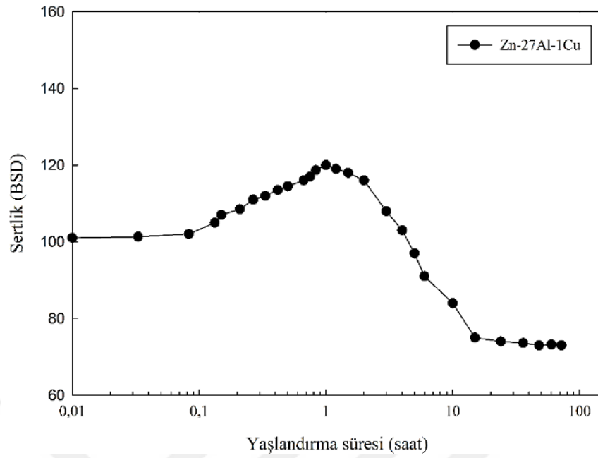
Şekil 14. Zn-27Al-1Cu alaşımasının sertliğinin yaşlandırma süresine göre değişimini gösteren eğri
