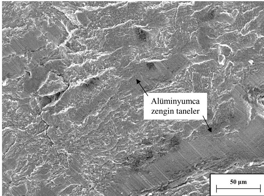
Şekil 28. 160 MPa gerilme değeriinde yorulma deneyine tabi tutulan, 1 saat yaşılandırılmış durumdaki Zn-27Al-1Cu alaşıma ait numunenin kırılma yüzeyinin detayını gösteren SEM fotoğrafı
