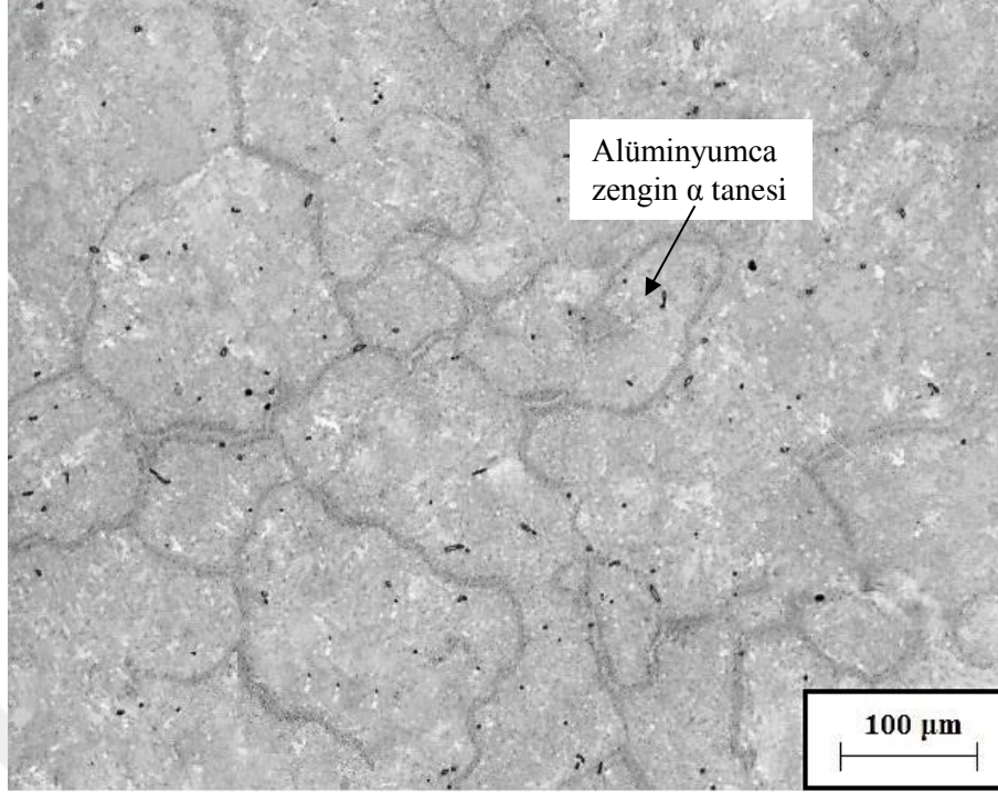
Şekil 9. 100 °C sıcaklıkta 0,5 saat yaşılandırılan Zn-27Al-1Cu alaşımasının içyapısı
