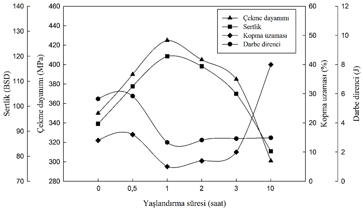
Şekil 16. Dökülmüş ve ısıt işlem görmüş durumlardaki Zn-27Al-1Cu alaşımının mekanik özelliklerinin uygulanan yaşlandırma süresine göre değişim grafiği
