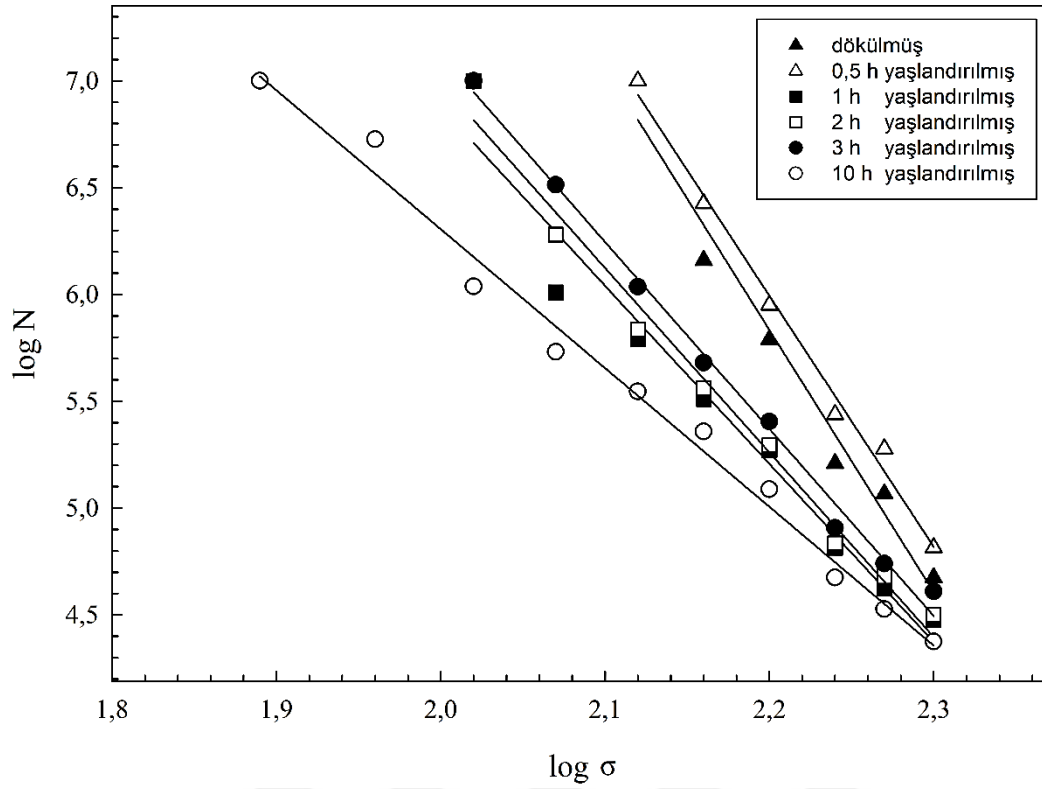
Şekil 20. Dökülmüş ve farklı sürelerde yaşlandırma işlemi uygulanmış Zn-27Al-1Cu alaşımının logN–logσ eğrileri
