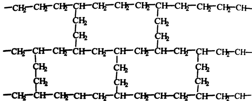
Şekil 2.9 Çapraz bağlı polietilen
