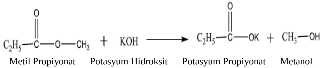
Şekil 3.9 Sabunlaşma tepkimesi
