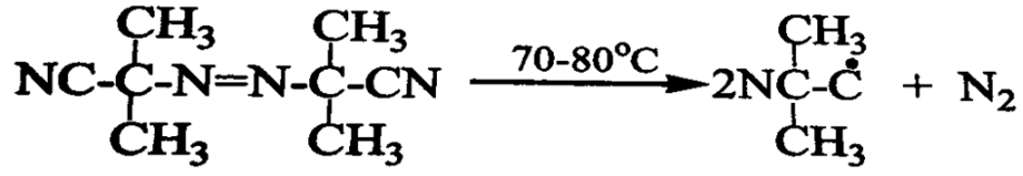
Şekil 2.24 Azobisisobutironitril (AIBN)
