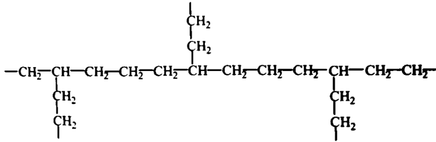
Şekil 2.8 Dallanmış polietilen
