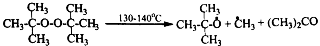
Şekil 2.23 Ter-butil peroksit
