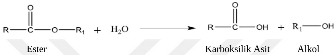
Şekil 3.8 Hidroliz tepkimesi
