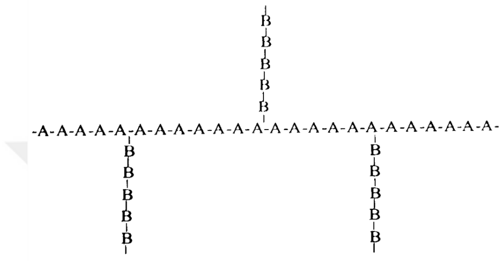
Şekil 2.17 Aşı kopolimer
