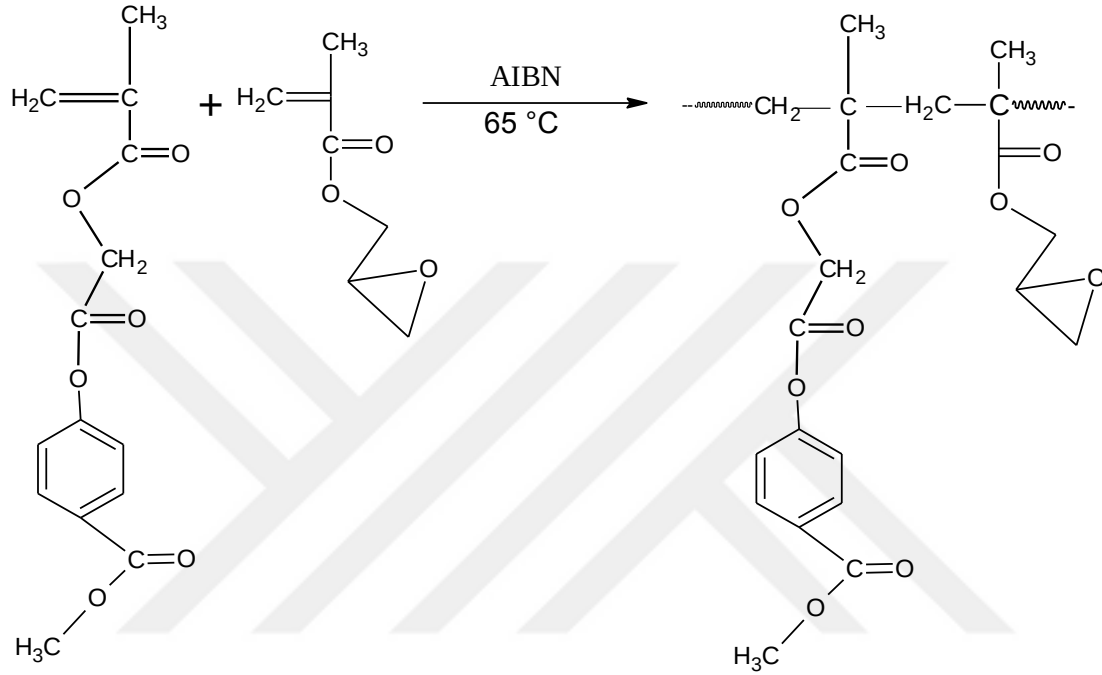
Şekil 7.4 Kopoli(MMOAB-GMA) sentezi
