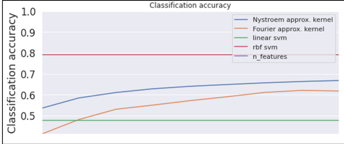
Şekil 5.71. Sınıflandırma doğruluk grafiği ekran görüntüsü
