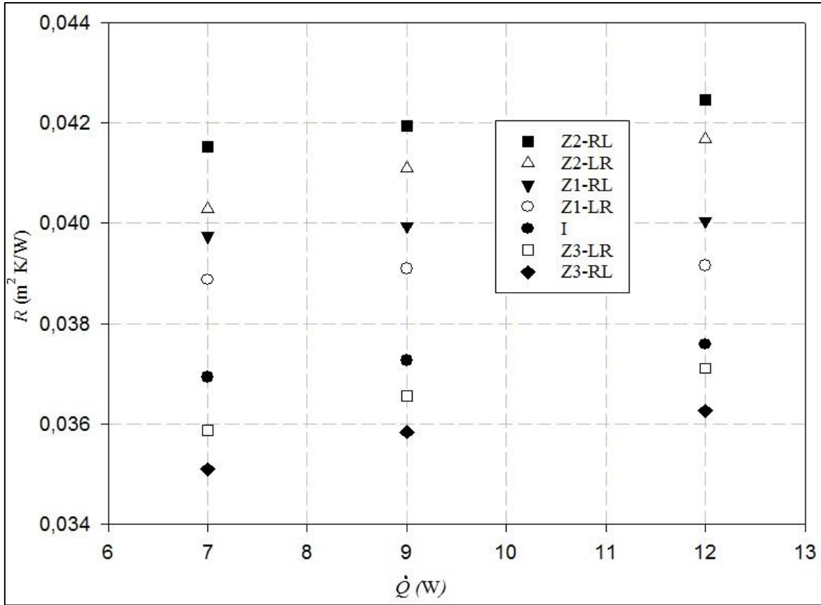
Şekil 29. Deney örneklerinde eşdeğer termal direncin ısıl güce bağlı olarak değişimi
