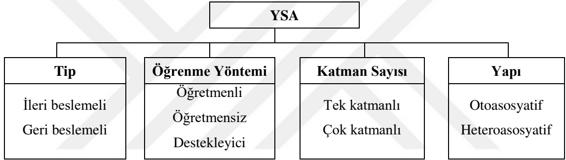
Şekil 5. YSA'ların sınıflandırılması
