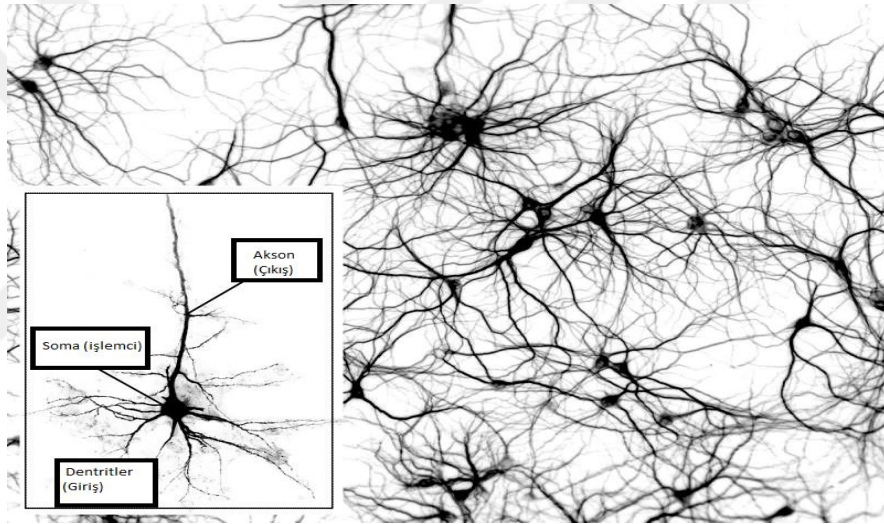
Şekil 3.15. Çok sayıda enterkonnekte nöronlardan oluşan biyolojik sinir ağının teorik gösterimi [25]
