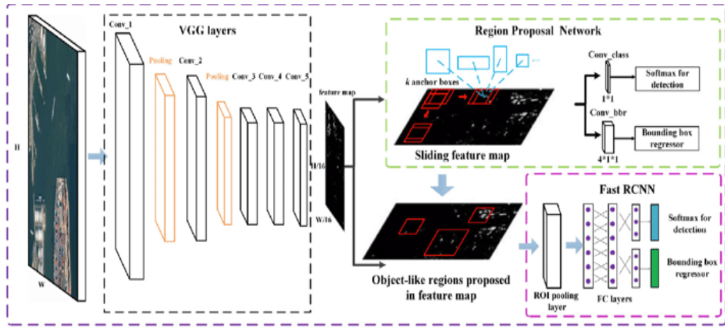
Şekil 24. Faster R-CNN mimarisi (Li vd., 2018)
