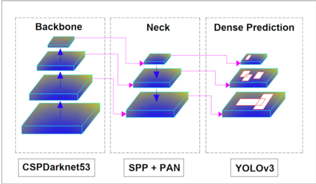
Şekil 28. YOLOv4 mimarisi (Park vd., 2021)
