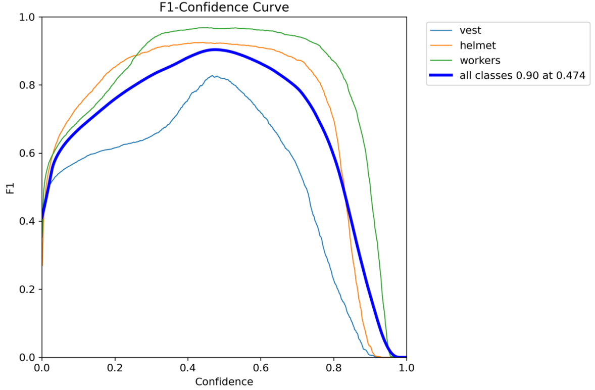
Şekil 33. YOLOv5 F1-Güven eğrisi
