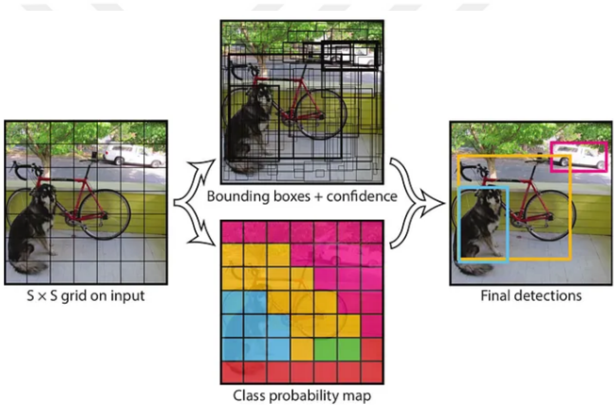
Şekil 26. YOLOv1 (Zhang, 2020)
