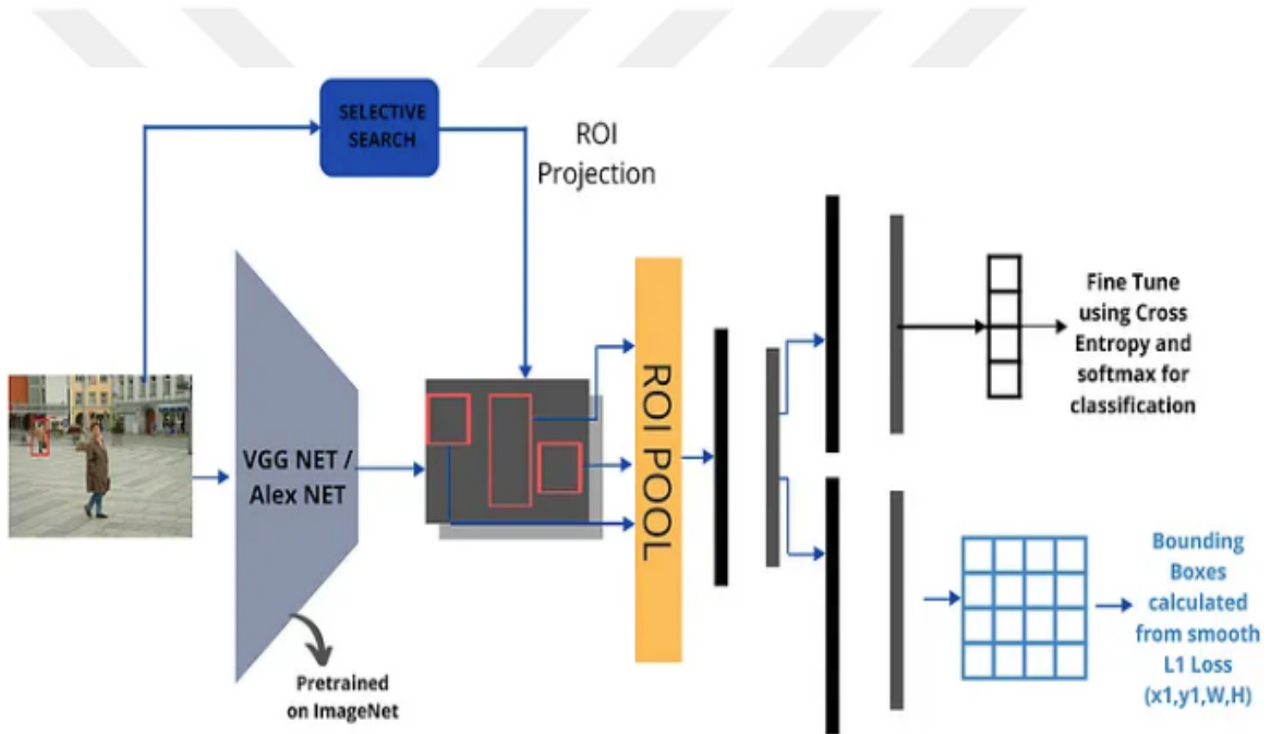
Şekil 14. Fast R-CNN
