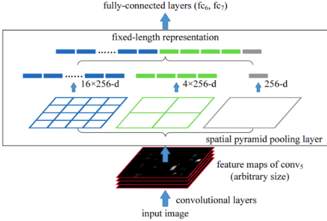
Şekil 16. SPPNet
