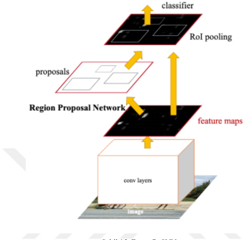
Şekil 15. Faster R-CNN
