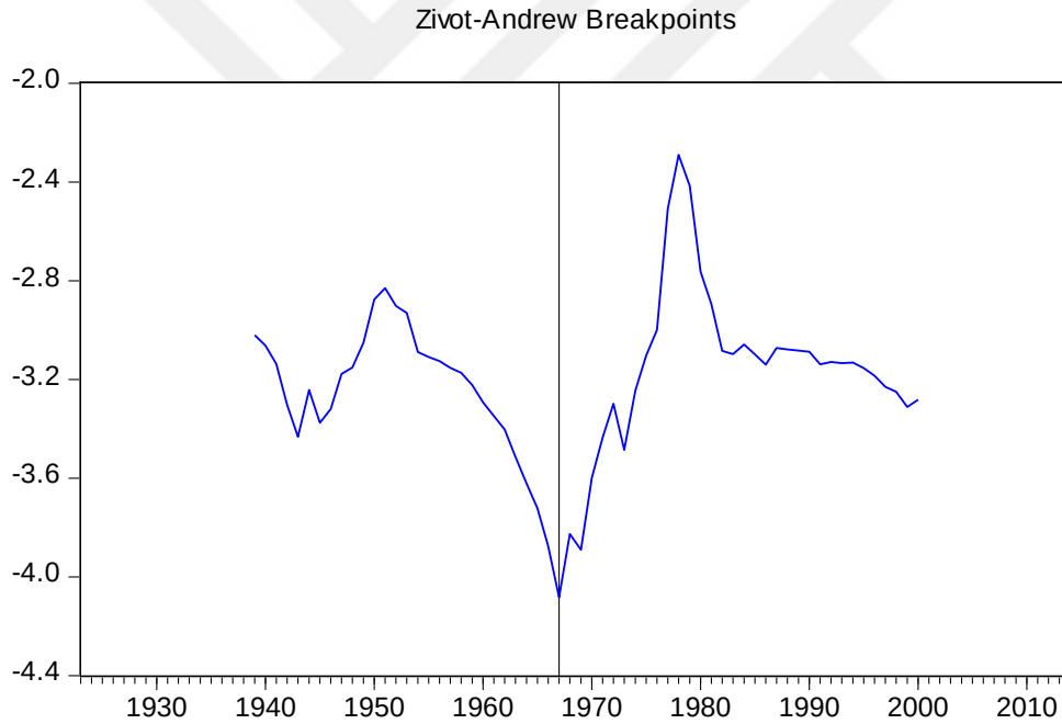
Şekil 4.1 Zivot-Andrews (1992) Kırılma Grafiği
