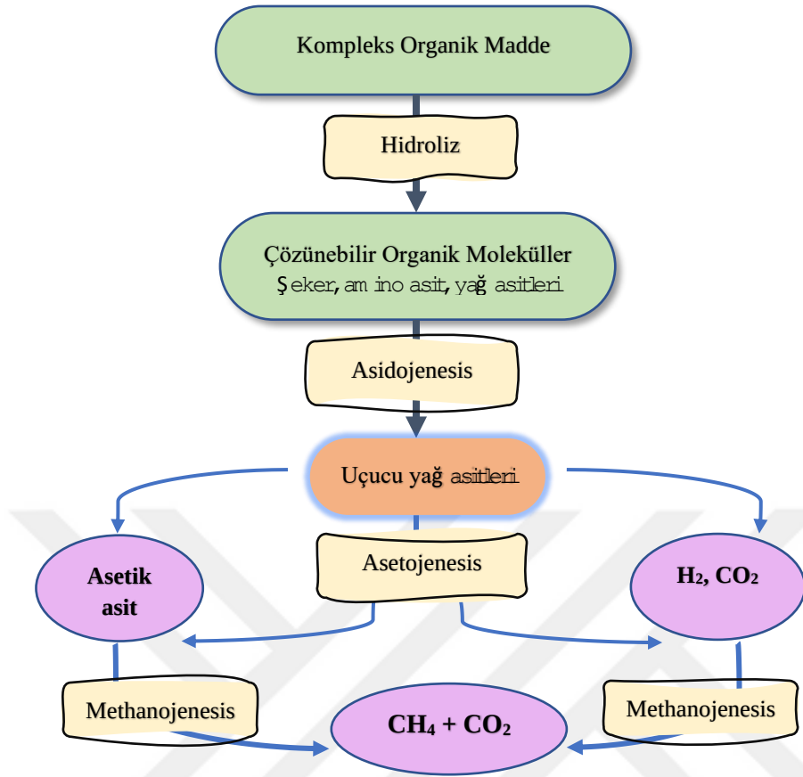
Şekil 2.6. Anaerobik parçalanma basamakları ve ürünler
