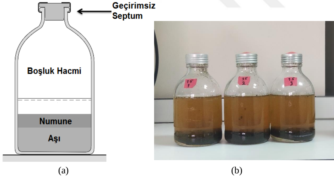
Şekil 3.2. (a) BMP reaktör konfigürasyonu, (b) BMP testi için hazırlanılmış reaktörler
