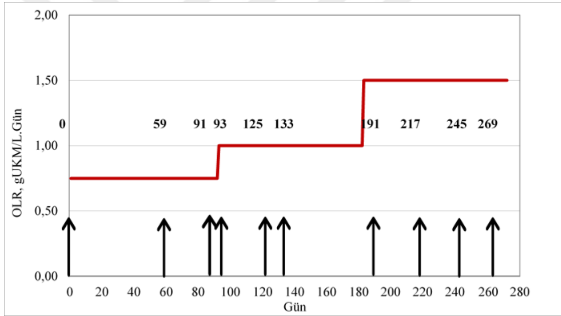
Şekil 3.12. Farklı organik madde yükleme değerlerinde yarı sürekli anaerobik reaktörden numune alım günleri
