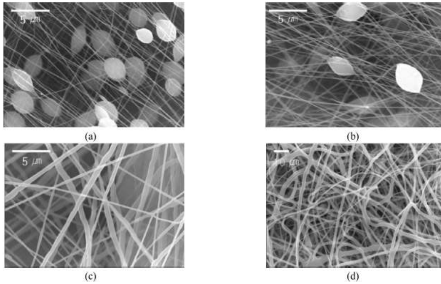
řekil 2.10.Deėiřik konsantrasyonlarda hazırlanan zeltilerden elde edilen PCL nanofiberlerin SEM grntleri. PCL konsantrasyonları; (a) %8, (b) %10, (c) %12, (d) %16 [74].
