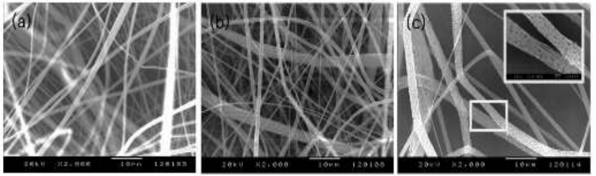
Şekil 2.15. %2.5'luk PLDLA çözeltisinin nem oranının fiber morfolojisi üzerindeki etkisi (akış hızı= 0.005mL/min, voltaj= 20kV): (a) %30 nem oranı, (b) %50 nem oranı, (c) %70 nem oranı.
