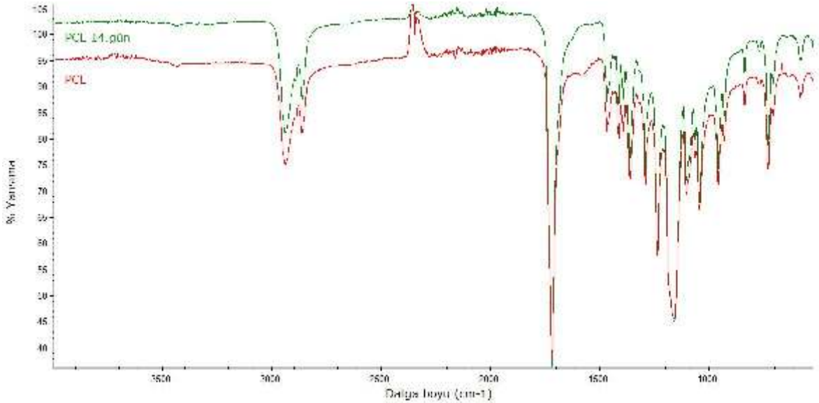
Şekil 4.14. Bozunma öncesi ve 14 gün süresince bozunmaya uğratılmış PCL doku iskelelerine ait FTIR spektrumları.
