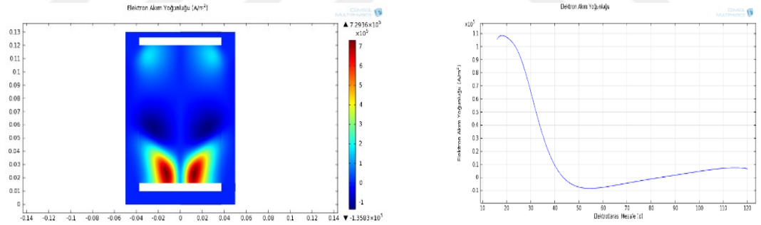
Şekil 2.17. (devam) 220 Torr basınç ve d = 100 \mu m için elektron akım yoğunluğu desenleri a) GaAs b) ZnSe c) CdS d) GaP e) InP
