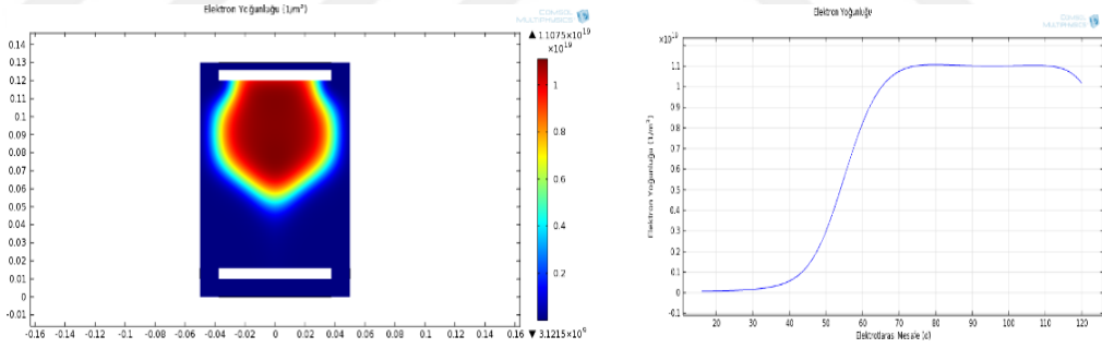
Şekil 2.10. (devam) 100 Torr basınç ve d = 100 \mu\text{m} için elektron yoğunluğu desenleri a) GaAs b) ZnSe c) CdS d) GaP e) InP
