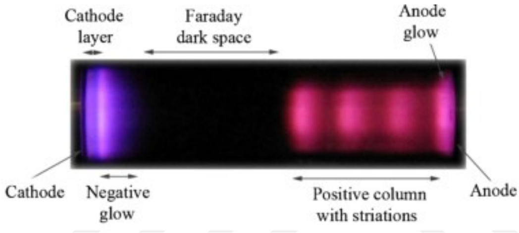
Şekil 1.5. Pozitif bölgeyle nitrogen bir DC glow boşalmasının yapısı
