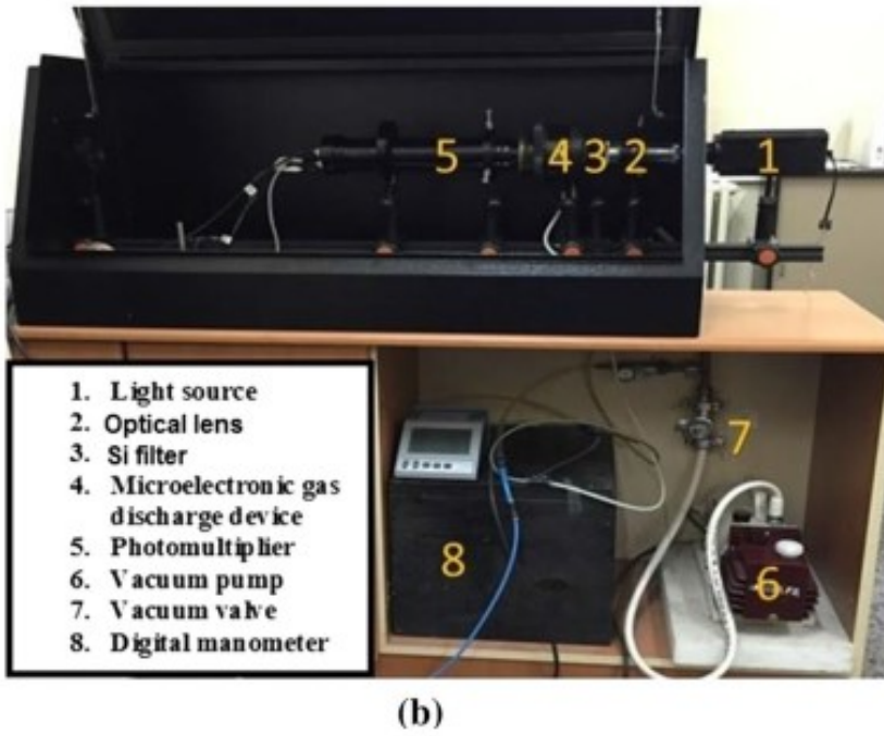
Şekil 4.12. a) Yarıiletken plazma hücresinin IR görüntü çeviricisi için olan sistemi 1) Işık kaynağı 2) Si filtre 3) IR ışık demeti 4) Yarıtransparan altın kontakt 5) ZnS ve ZnSe materyalleri 6) Gaz yük boşalma hücresi 7) Mika 8) UV-görünür ışık demeti 9) transparan iletkenli SnO 2 kontakt 10) Cam disk b) ZnSe ve ZnS elektrotlarının gaz plazma sistemi
