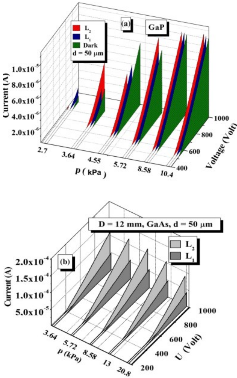
Şekil 3.5. 50 \mu m elektrotlararası mesafe için farklı aydınlatma şiddetleri altındaki AVK değerleri a) GaP b) GaAs
