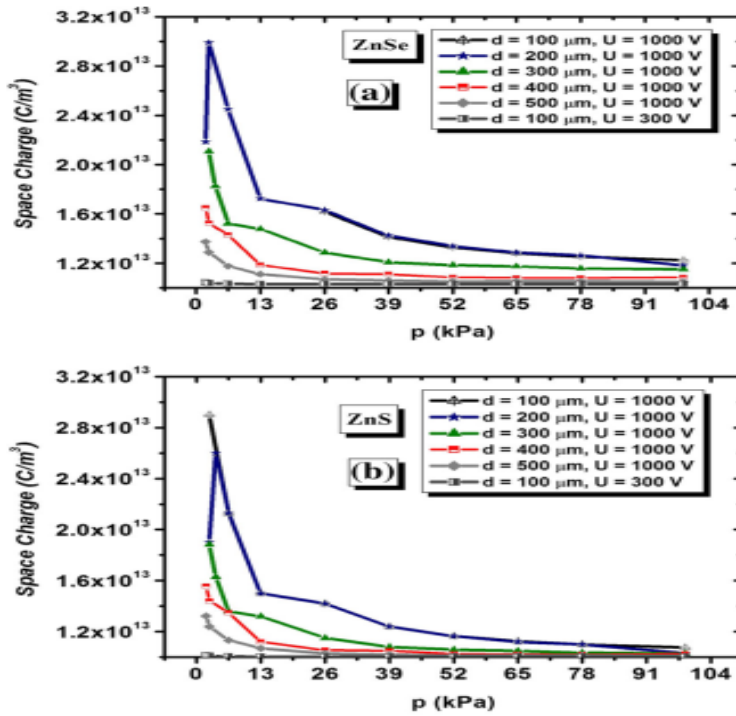
Şekil 4.5. Aynı plazma parametre değerleri için uzaysal yük yoğunluğu a) ZnSe b) ZnS
