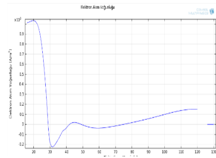
Şekil 2.14. 160 Torr basınç ve d = 100 \mu\text{m} için elektron akım yoğunluğu desenleri a) GaAs b) ZnSe c) CdS d) GaP e) InP
