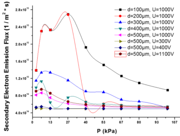
Şekil 5.6. Elektrotlarası geçiş ve uygulanan voltaj için ikincil elektron emisyonu – gaz basıncı eğrisi
