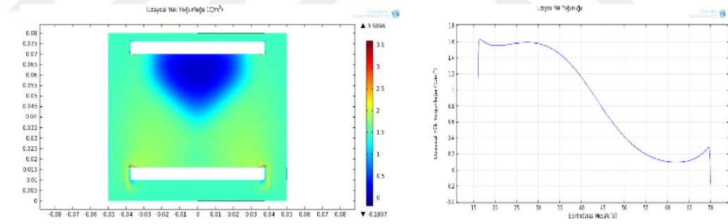
Şekil 2.6. (devam) 220 Torr basınç ve d = 50 \mu\text{m} için uzaysal yük yoğunluğu desenleri a) GaAs b) ZnSe c) CdS d) GaP e) InP
