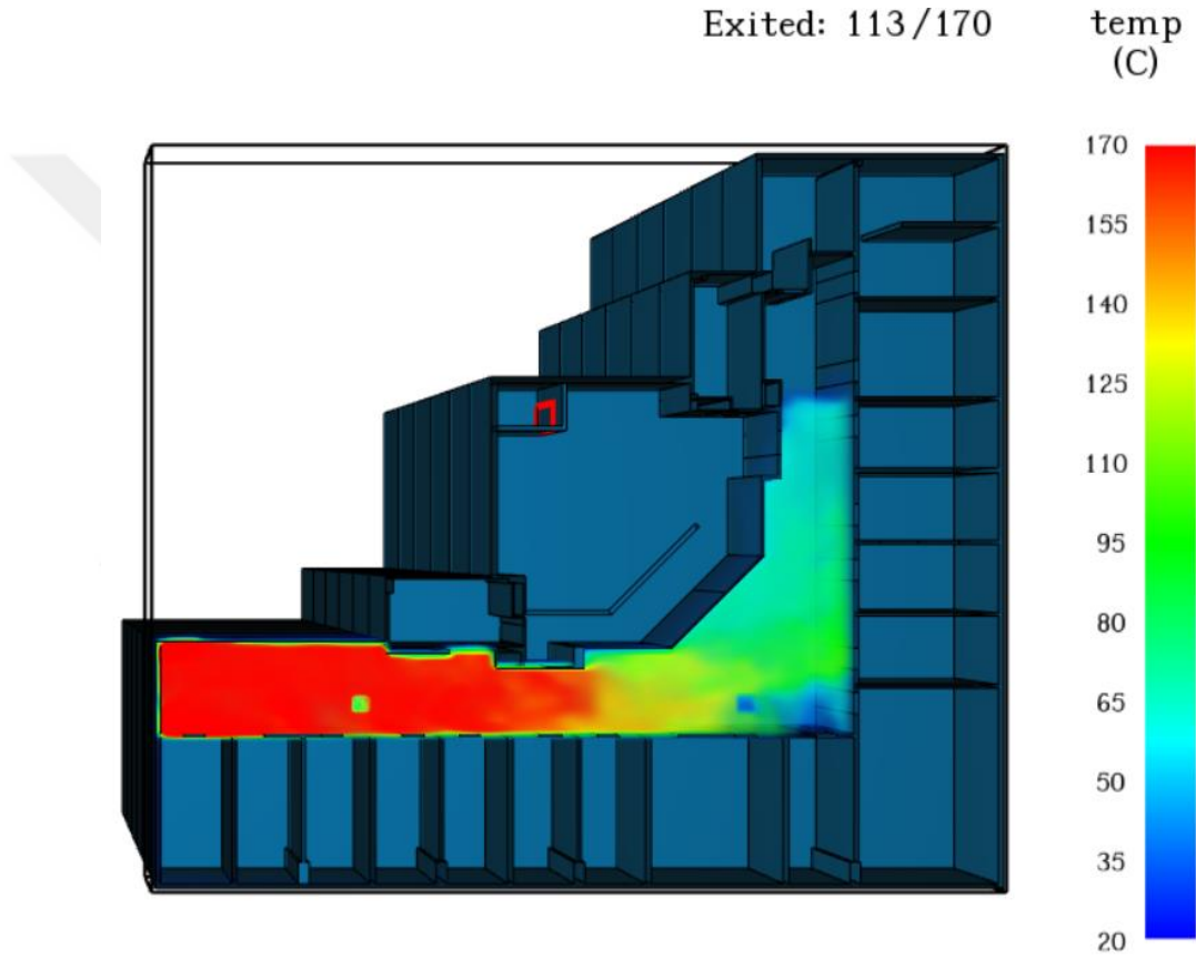
Şekil 6.100. Senaryo4'e göre 250. saniyede koridorda oluşan sıcaklık değerleri (°C)
