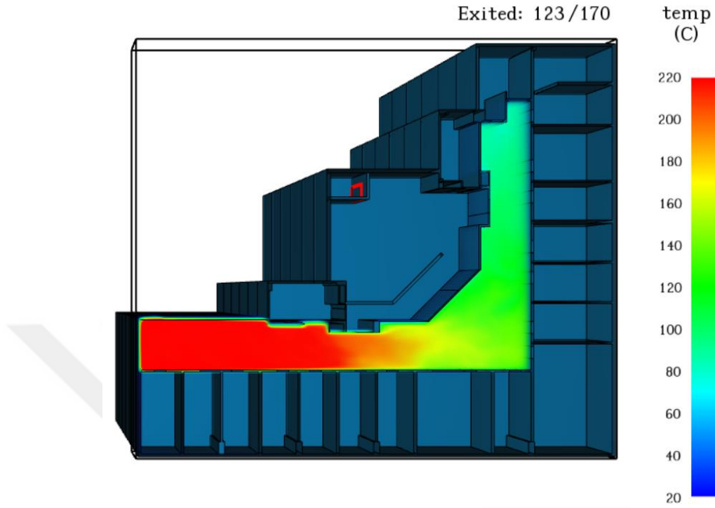
Şekil 6.6. Senaryo1'e göre 250. saniyede koridorda oluşan sıcaklık değerleri (°C)
