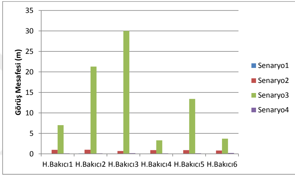
Şekil 6.4. 1,8 metrede görüş mesafelerinin en düşük değerinin grafik ile karşılaştırılması (5 m 3 /s)
