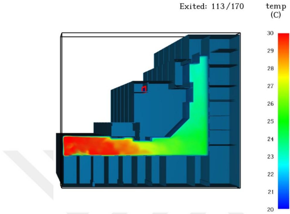
Şekil 6.8. Senaryo2'ye göre 250. saniyede koridorda oluşan sıcaklık değerleri (°C)
