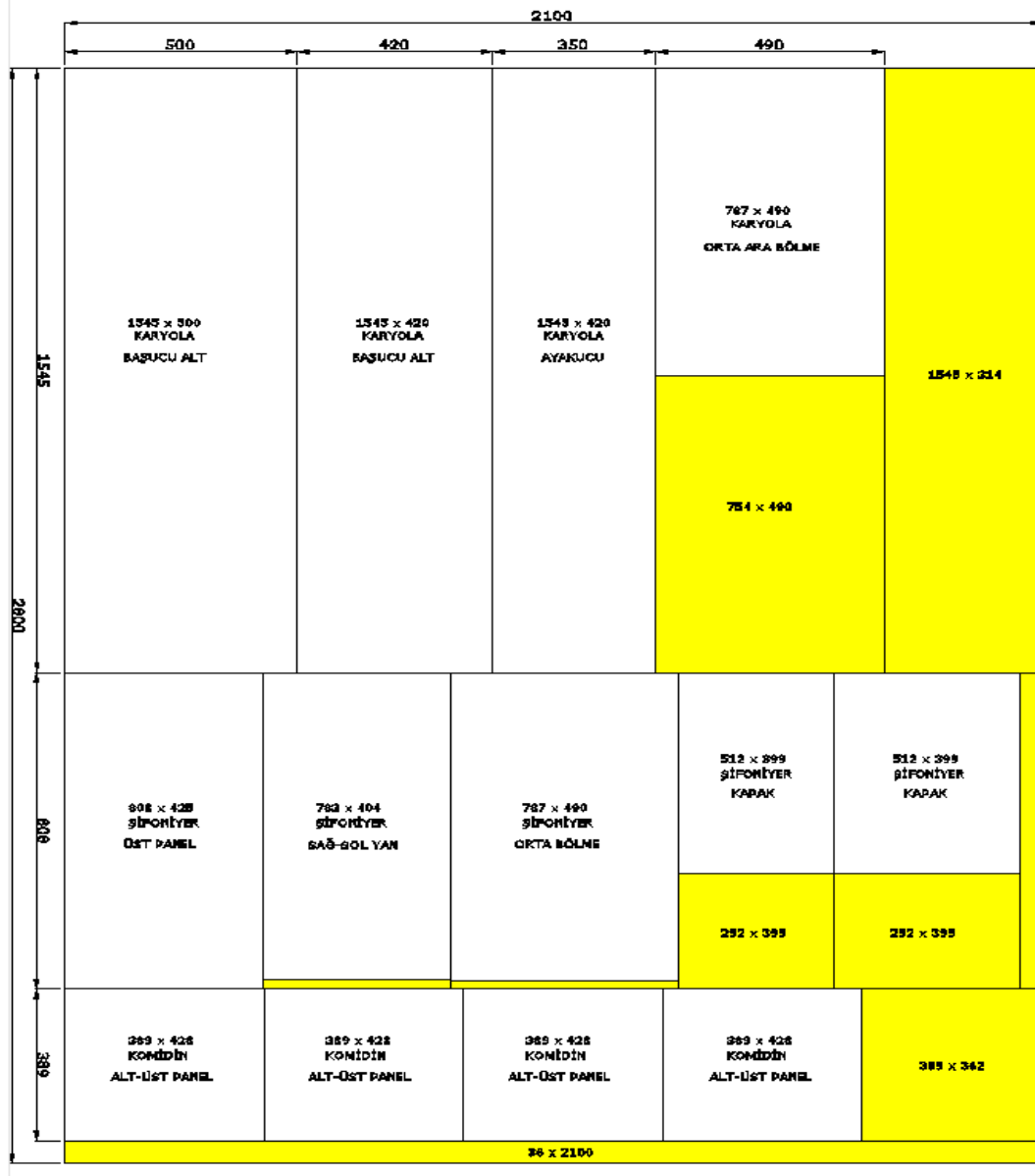
Şekil 14. Levha boyutlandırma makinesinde 3. kesme işlemine ait kesim planı
