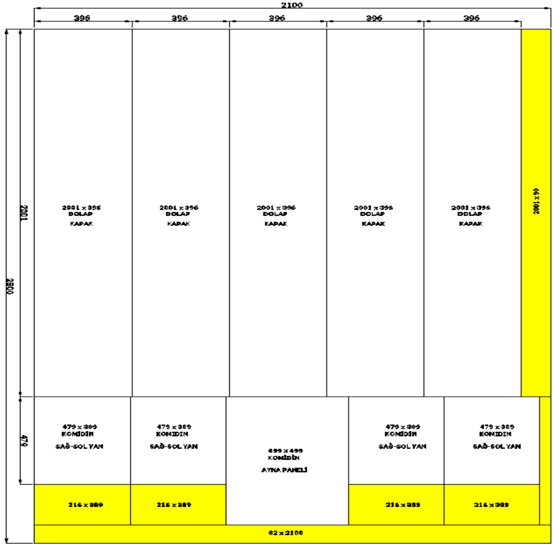
Şekil 15. Levha boyutlandırma makinesinde 4. kesme işlemine ait kesim planı
