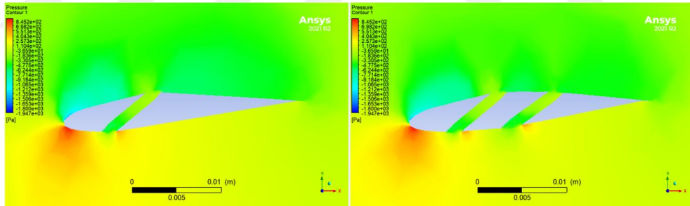
Şekil 5.5. 3. ve 4. simülasyonun hava akış yarıkların basınç dağılımı.
