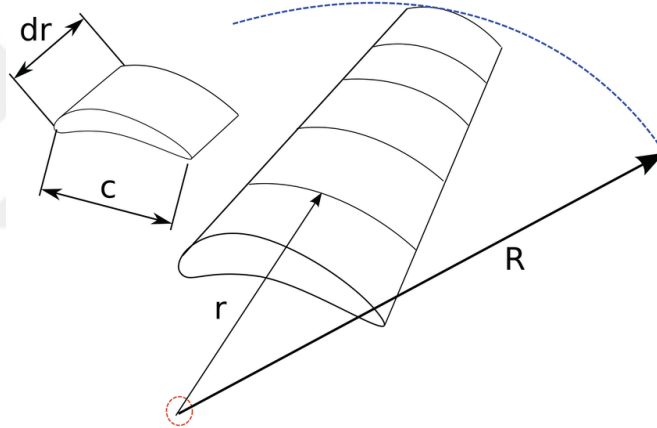
Şekil 3.4. Rüzgar türbini kanadı üzerinde kanat elemanı teorisinin çizimi.
