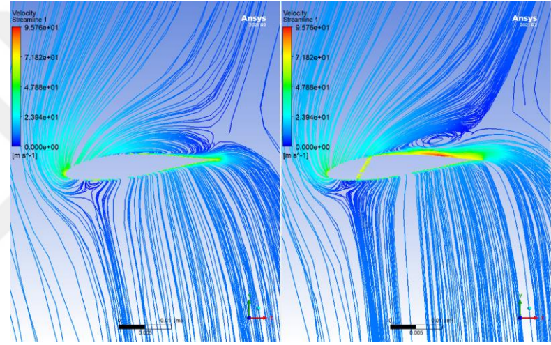
Şekil 5.14. 160 rad/s açısai hızında kanat profilin üzerindeki akış çizgileri.
