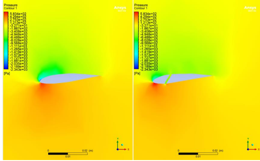
Şekil 5.17. 80 rad/s açısal hızında kanat profilin üzerindeki basınç dağılımı.
