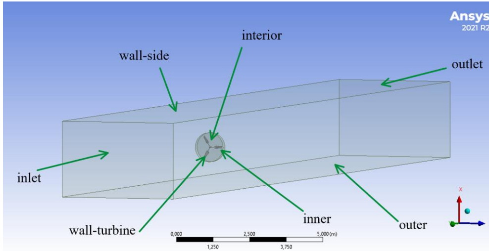
Şekil 4.22. Sınır koşulları.
