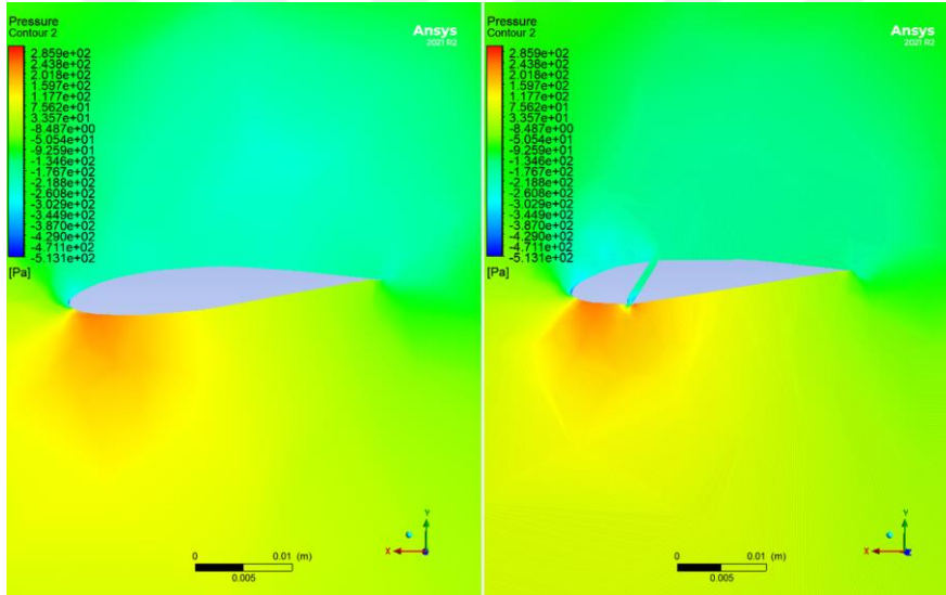
Şekil 5.16. 40 rad/s açısal hızında kanat profilin üzerindeki basınç dağılımı.
