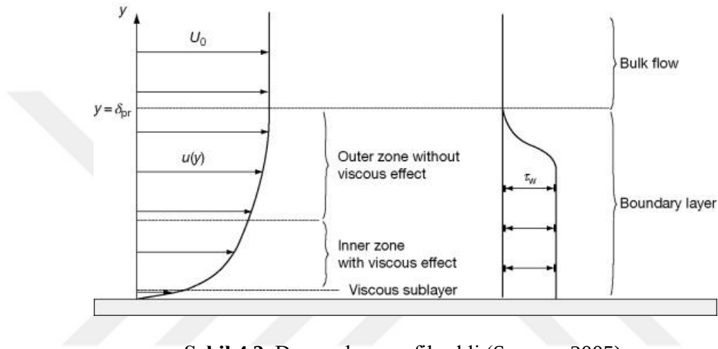
Şekil 4.2. Duvar alanı profil şekli (Somers, 2005).
