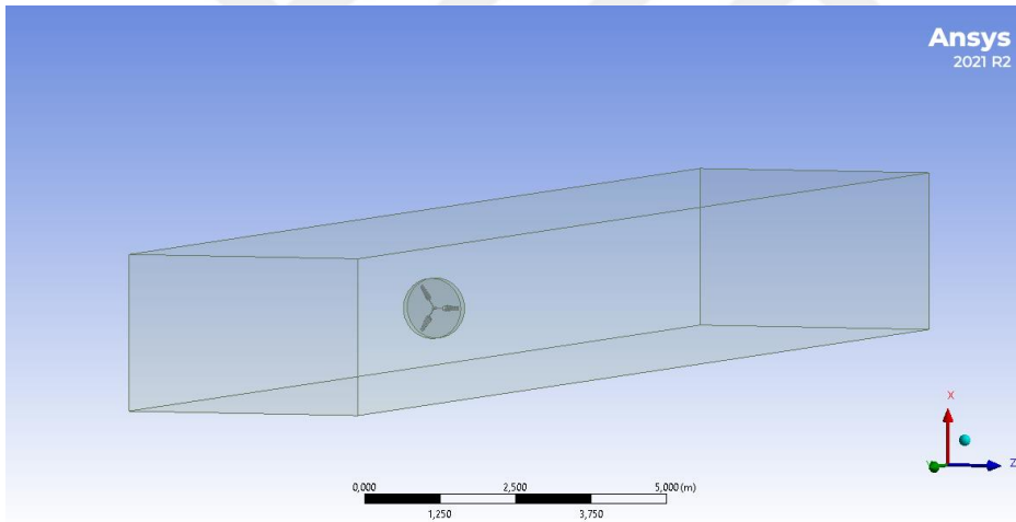
Şekil 4.21. Deneyisel araştırmaya benzer rüzgar tüneli.
