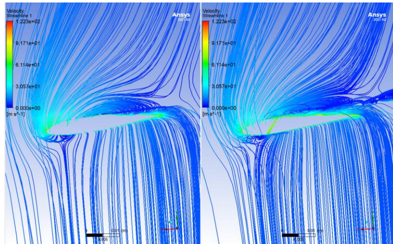
Şekil 5.15. 180 rad/s açısai hızında kanat profilin üzerindeki akış çizgileri.
