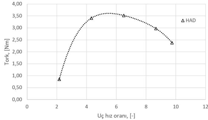
Şekil 4.33. Rüzgar türbinin torku.
