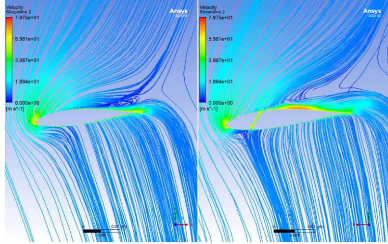
Şekil 5.13. 120 rad/s açısai hızında kanat profilin üzerindeki akış çizgileri.
