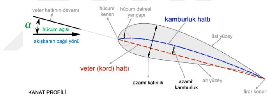
Şekil 2.2. Kanat profili.
