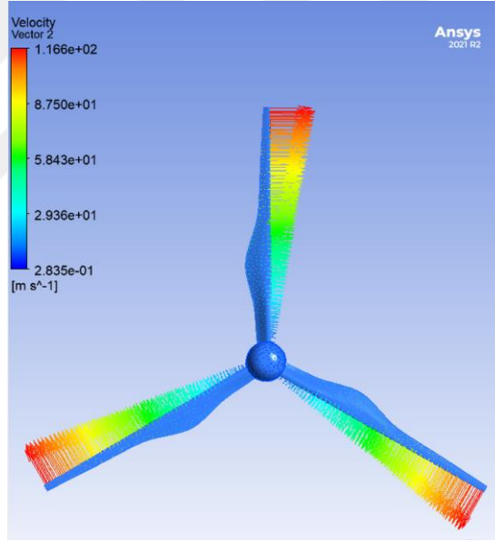
Şekil 5.10. 180 rad/s açısıl hızında Y vektörü yönüne göre hız vektörleri.
