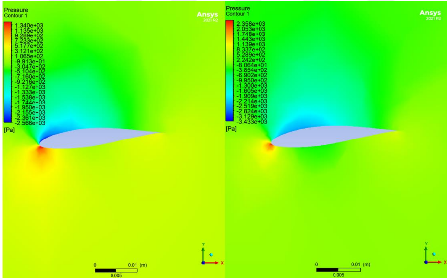
Şekil 4.31. Kanadın 0,4 m, 120 rad/s (sol) ve 160 rad/s (sağ) açısall hızında kanat profili üzerindeki basınç dağılımı.
