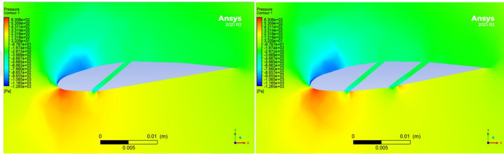
Şekil 5.4. 1. ve 2. simülasyonun hava akış yarıkların basınç dağılımı.
