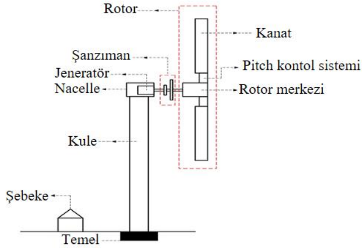
Şekil 2.1. Rüzgar türbininin ana bileşenleri.
