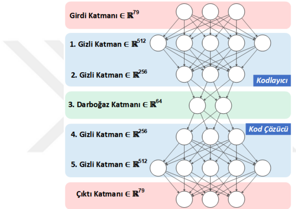
Şekil 2.7. Modellerde kullanılan AE ve VAE'nin mimari diyagramı.
