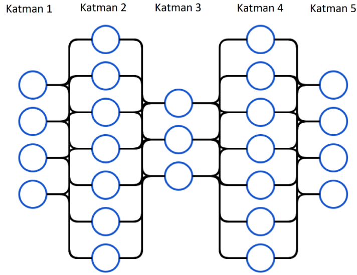
Şekil 3.3. Tekrarıcı sinir ağının örnek bir diyagramı [136]
