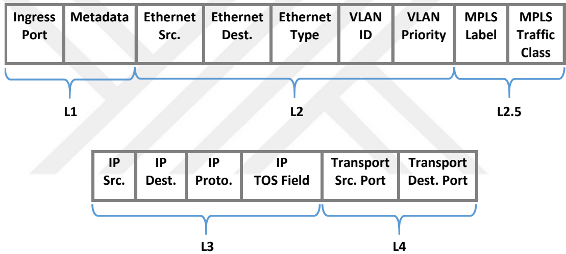
Şekil 3.2. OpenFlow'da akış [119]
