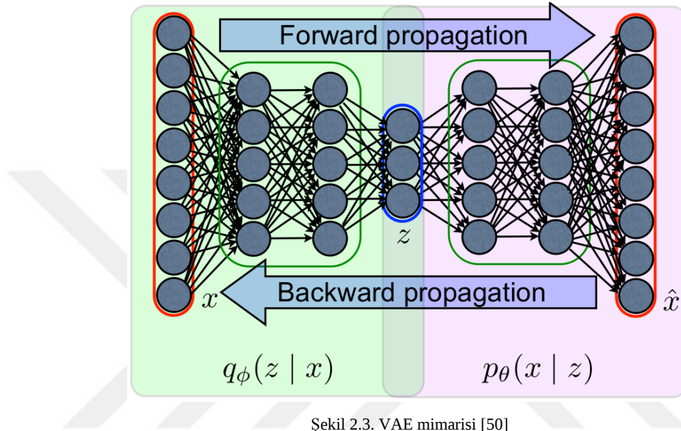
Şekil 2.3. VAE mimarisi [50]
