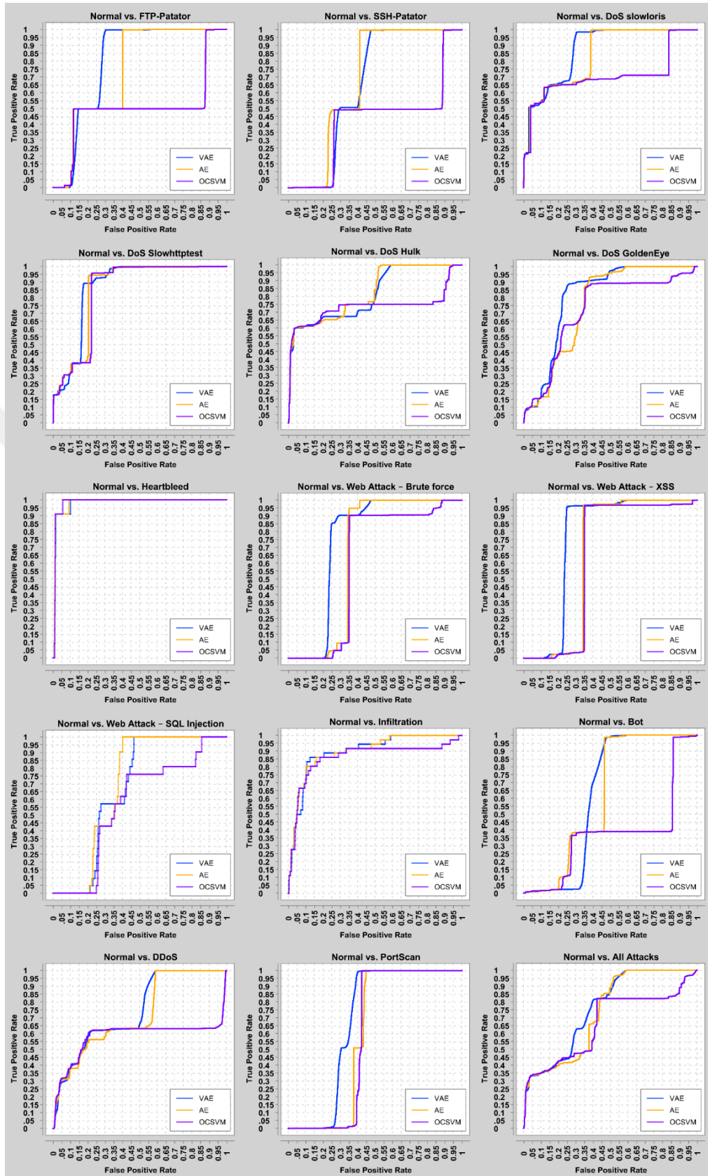
Şekil 2.8. ROC eğrileri
