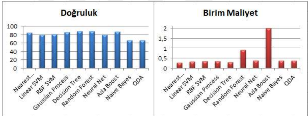
Şekil 6.8. Sport-stdddev öznitelik çifti doğruluk ve birim maliyet oranları
