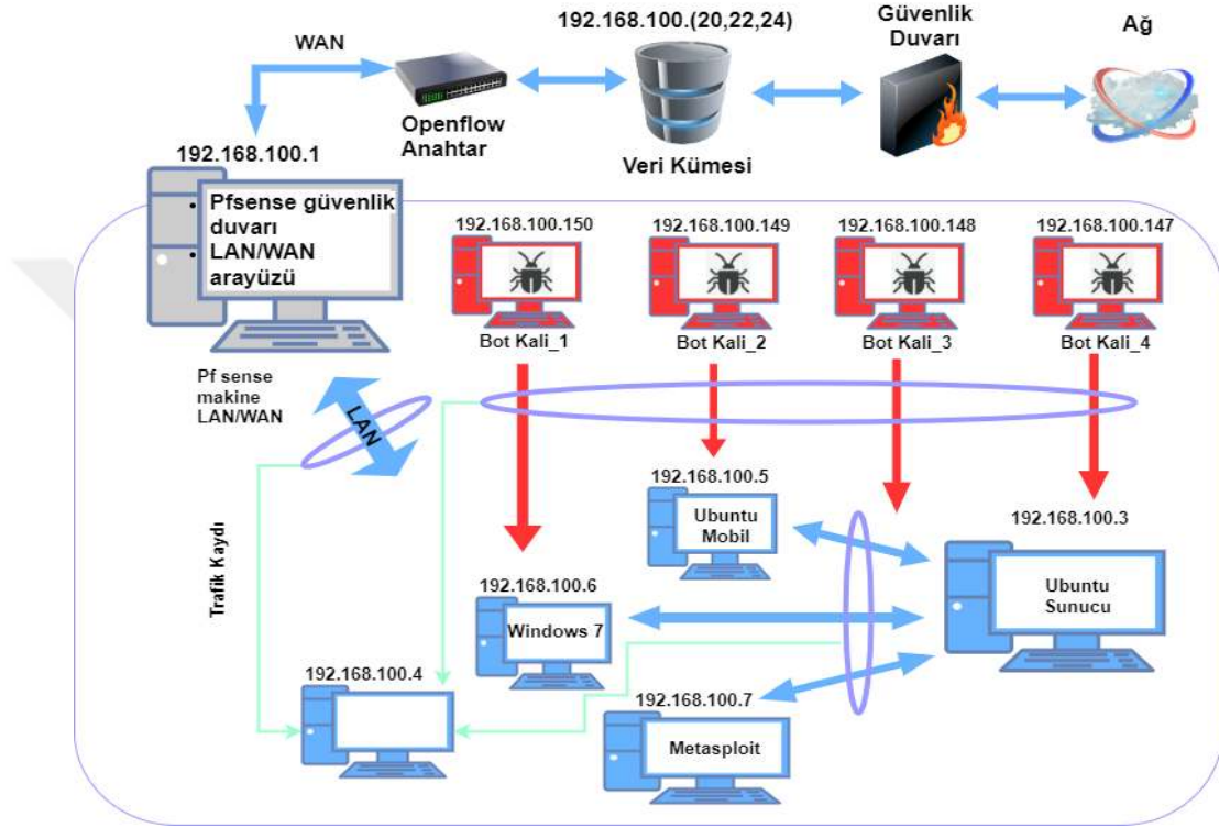
Şekil 6.2. Çalışmada oluşturulan topoloji
