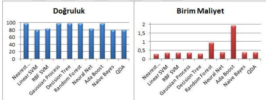
Şekil 6.24. Dport-drate öznelik çifti doğruluk ve birim maliyet oranları
