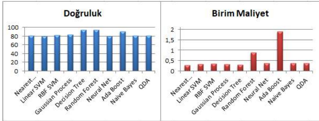
Şekil 6.15. Sport-srate öznitelik çifti doğruluk ve birim maliyet oranları
