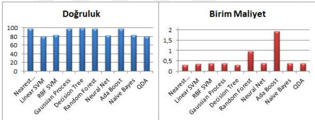
Şekil 6.26. Dport- max öznelik çifti doğruluk ve birim maliyet oranları
