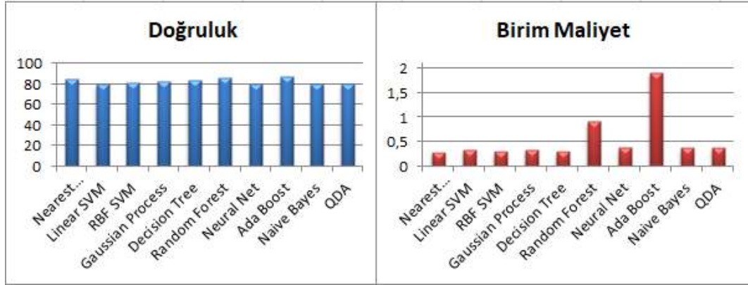
Şekil 6.63. Mean-drate öznelilik çifti doğruluk ve birim maliyet oranları
