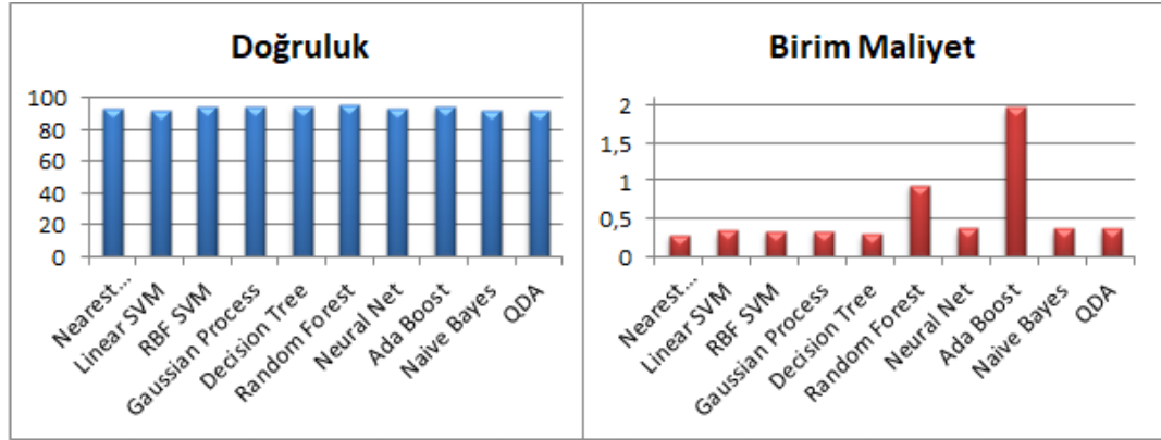
Şekil 6.31. Seq-mean öznitelik çifti doğruluk ve birim maliyet oranları
