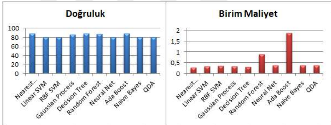
Şekil 6.54. Min-drat öznelik çifti doğruluk ve birim maliyet oranları
