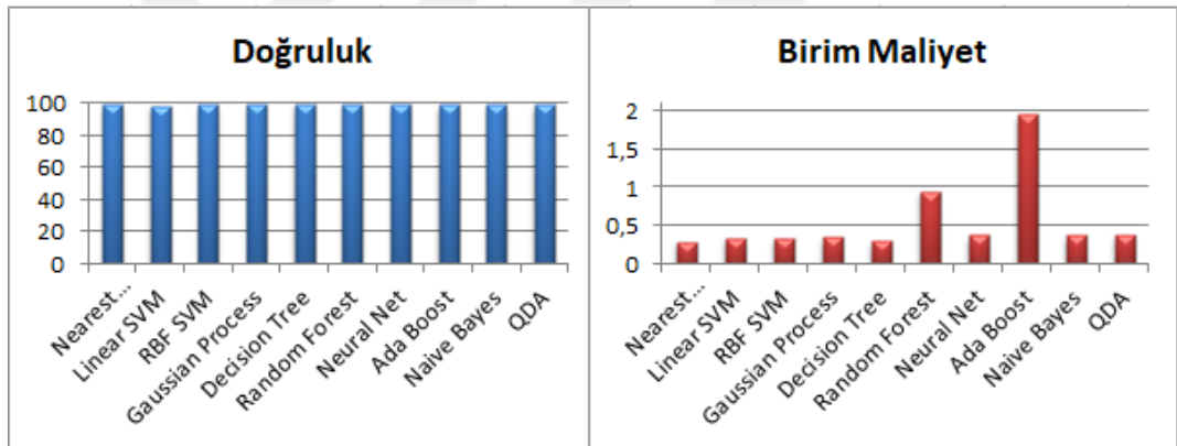
Şekil 6.32. Seq-N...DstIP öznitelik çifti doğruluk ve birim maliyet oranları
