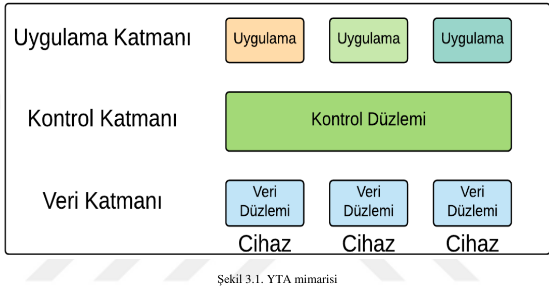
Şekil 3.1. YTA mimarisi
