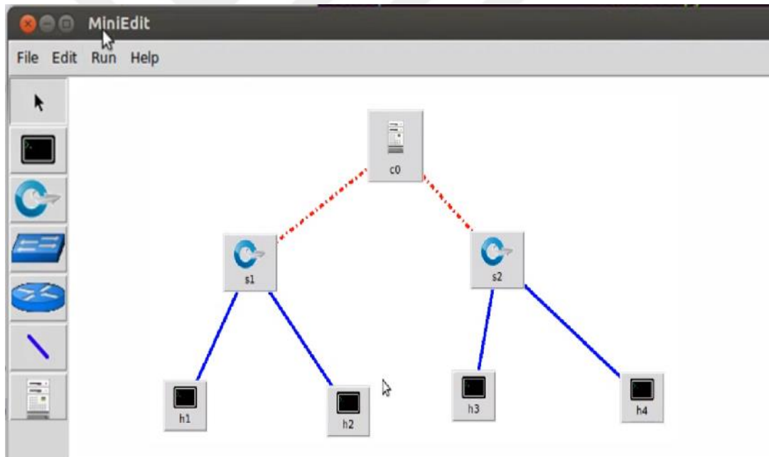
Şekil 5.1. Mininet arayüzü
