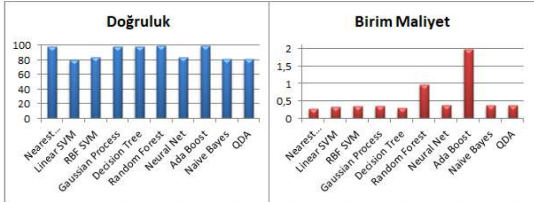
Şekil 6.25. Dport-srate öznelik çifti doğruluk ve birim maliyet oranları
