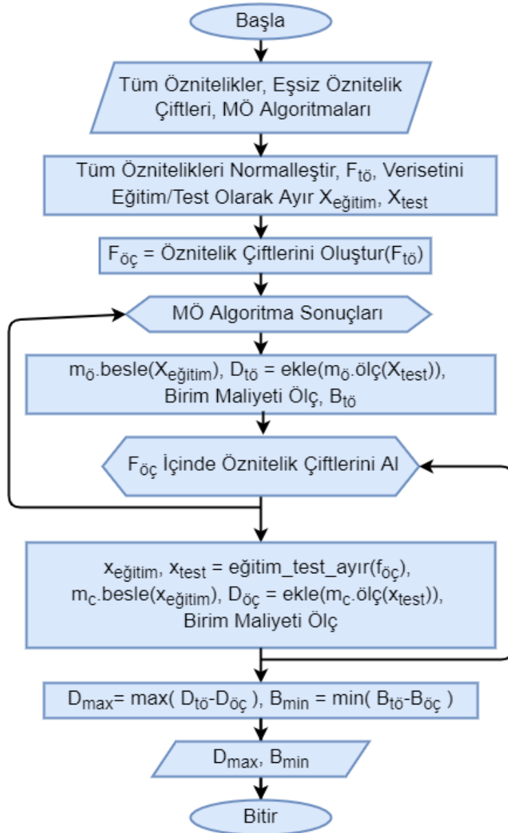
Şekil 6.1. Sistem Topolojisi
