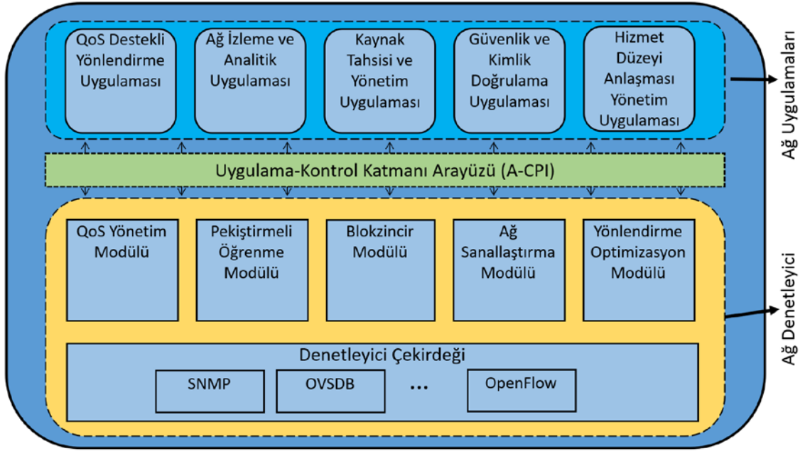
Şekil 6. Yazılım tanımlı çoklu ağlarda makine öğrenmesi ve blokzincir ile geliştirilmiş servis kalitesi destekli yönlendirme mimarisinde ağ denetleyicinin genel yapısı.
