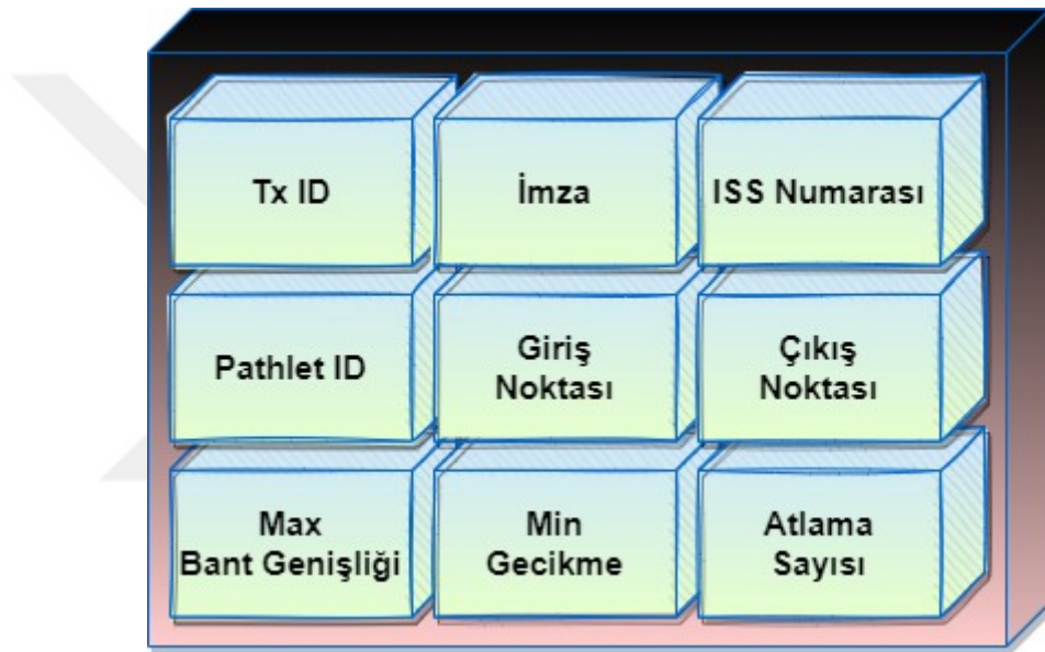
Şekil 5. Blokzincir özellikli hizmet kalitesi uyumlu ağlar arası yönlendirmedeki bir işlemin veri yapısı
