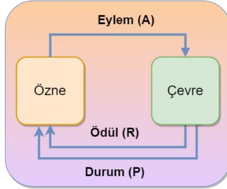
Şekil 3. Pekiştirmeli Öğrenme Mimarisi
