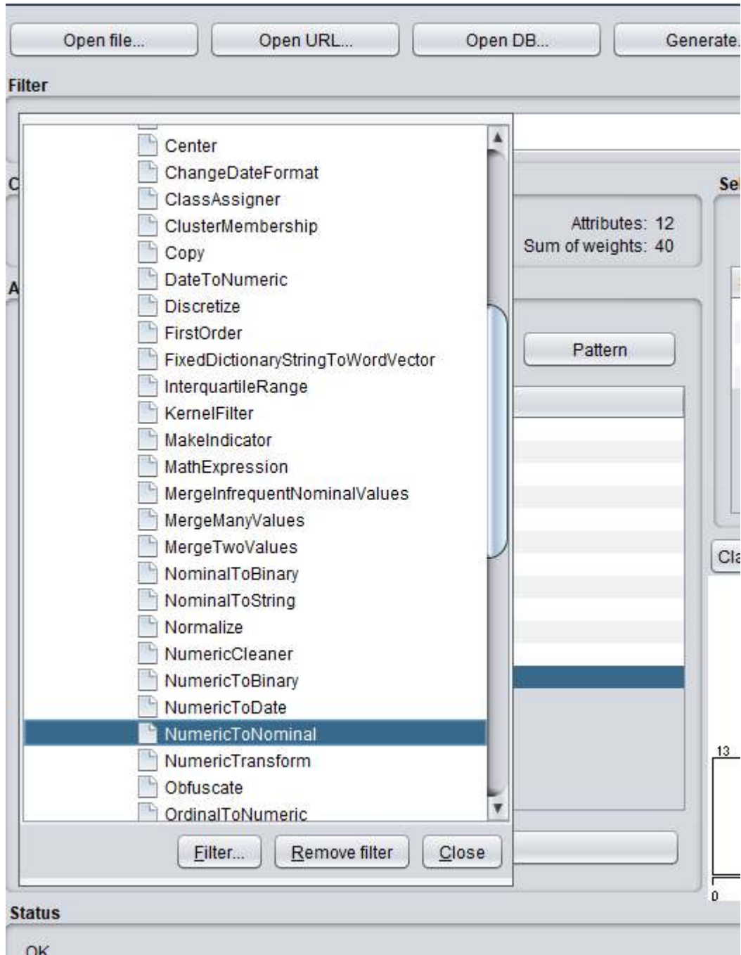
Görsel 2-2 Weka veri seti için filtreleme seçenekleri
