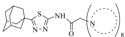
(3a-3j)
