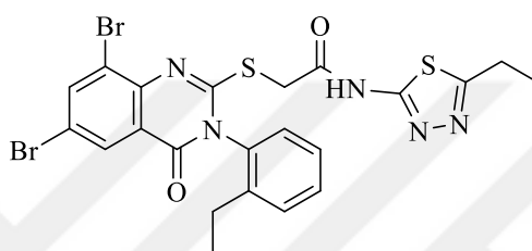
Figure 2.25. 2-((6,8-Dibromo-3-(2-ethylphenyl)-4-oxo-3,4-dihydroquinazolin-2-yl)thio)-N-(5-ethyl-1,3,4-thiadiazol-2-yl)acetamide
