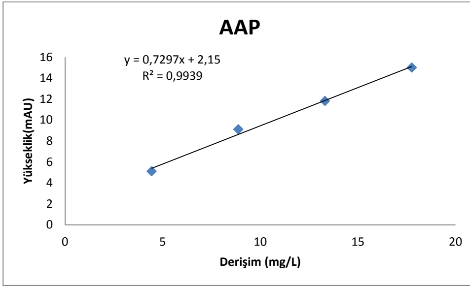
Şekil 4.10 AAP eklenen çözelti ilavesiyle değışen derişimine karşılık pik yüksekliğı kalibrasyon grafiğı
