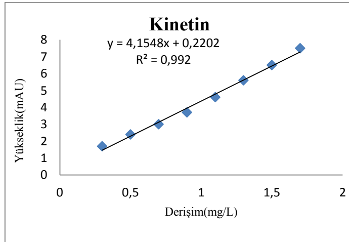
Çizelge 4.2 Kinetin için derişim ve pik yükseklięi deęerleri ve kalibrasyon grafięi
