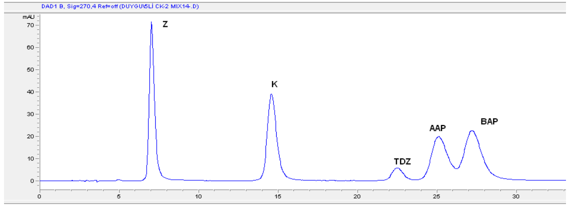
d) pH:5.48 40 mmol İzokratik elüsyon Akış hızı:1ml/min %20 ACN/Fosfat tamponu dalga boyu:270nm T:22 0 C enjeksiyon hacmi:10µl
