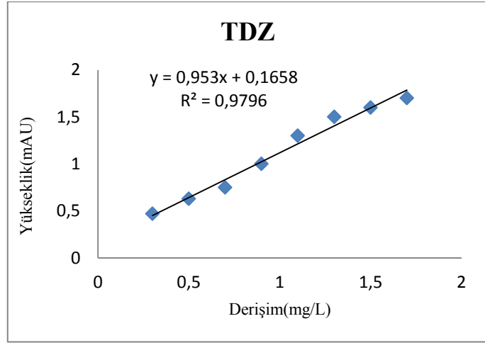
Çizelge 4.3 Thidiazuron için derişim ve pik yüksekliği değerleri ve kalibrasyon grafiğı
