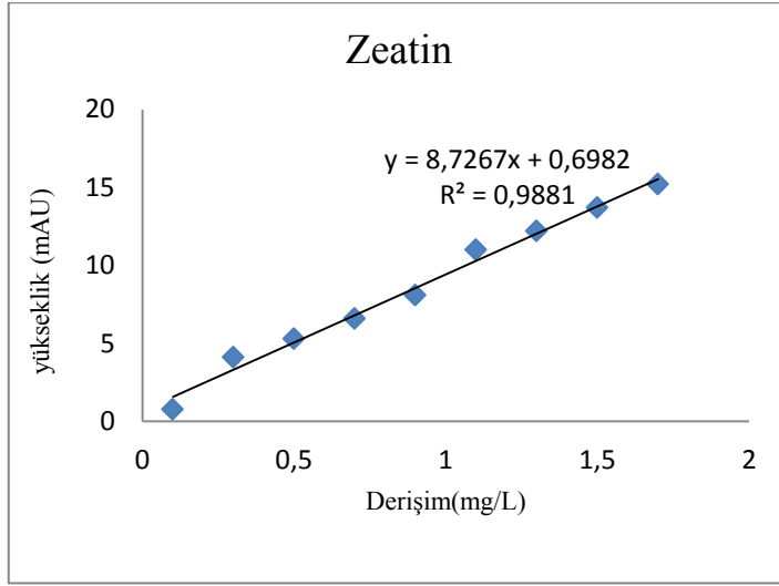
Çizelge 4.1. Zeatin için derişim ve pik yükseklięi deęerleri ve kalibrasyon grafięi
