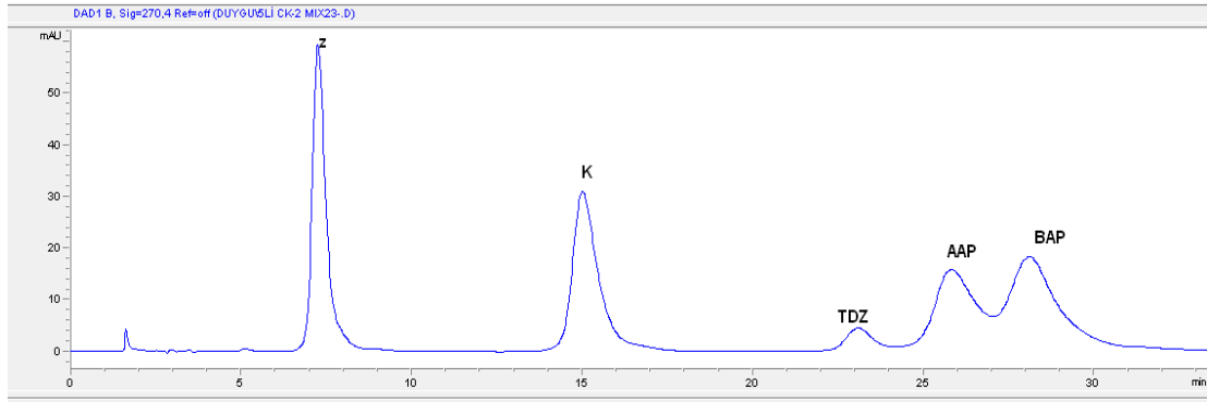
a) pH:5.48 10 mmol İzokratik elüsyon akış hızı:1ml/dk %20 ACN/fosfat tamponu dalga boyu :270nm enjeksiyon hacmi:10µl T:20 0 C
