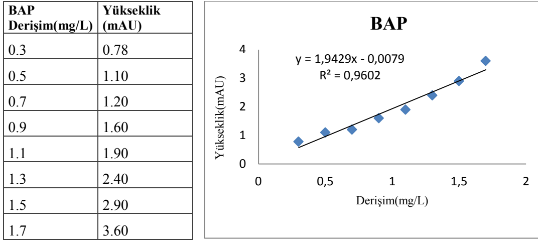
Çizelge 4.5 Benzilaminopürin için derişim ve pik yüksekliği değerleri ve kalibrasyon grafiğı
