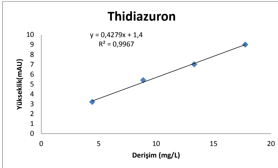
Şekil 4.9 Thidiazuron eklenen çözelti ilavesiyle değışen derişimine karşılık pik yüksekliğı kalibrasyon grafiğı
