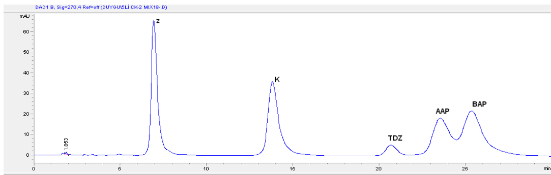
b) pH:5.48 10 mmol İzokratik elüsyon akış hızı:1ml/dk %20 ACN/fosfat tamponu dalga boyu :270nm enjeksiyon hacmi:10µl T:25 0 C
