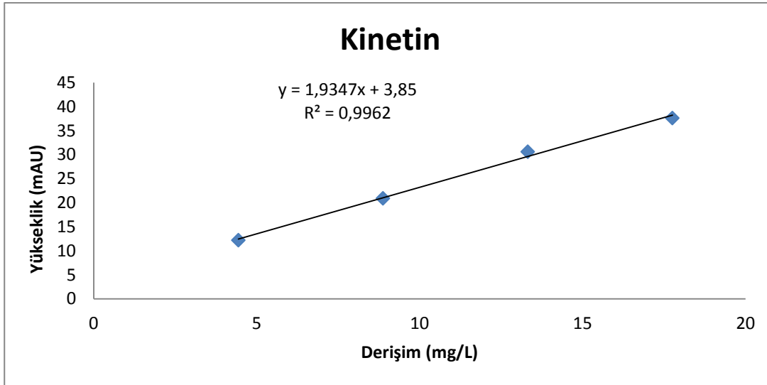
Şekil 4.8 Kinetinin eklenen çözelti ilavesiyle değışen derişimine karşılık pik yüksekliğı kalibrasyon grafiğı
