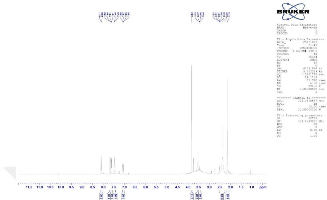
Şekil 5.63. Bileşik 4m'ye ait ^1\text{H} -NMR spektrumu
