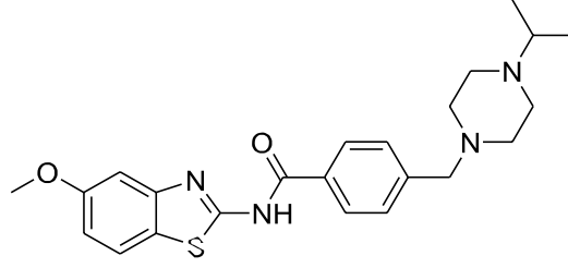
Şekil 5.56. 4-((4-izopropilpiperazin-1-il)metil)-N-(5-metoksibenzo[d]tiyazol-2-il)benzamid (4l)
