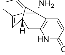
Şekil 2.6. Huperzin-A'nın kimyasal yapısı
