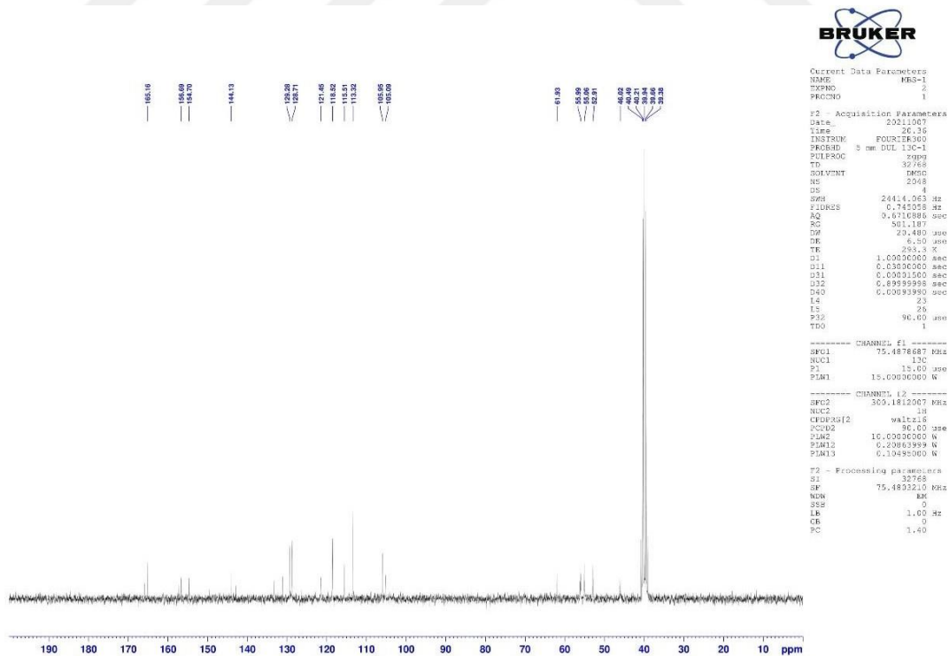
Şekil 5.39. Bileşik 4h'ye ait ^{13}\text{C} -NMR spektrumu
