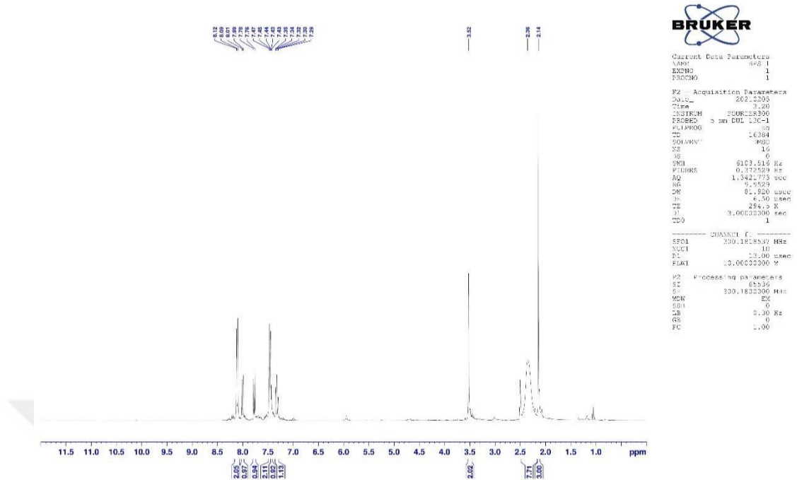
Şekil 5.3. Bileşik 4a'ya ait ^1\text{H} -NMR spektrumu
