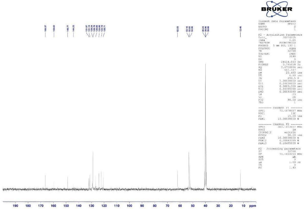
Şekil 5.9. Bileşik 4b'ye ait ^{13}\text{C} -NMR spektrumu
