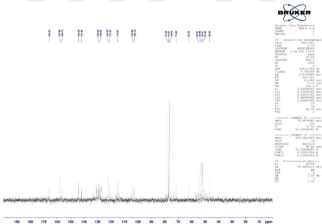
Şekil 5.54. Bileşik 4k'ye ait ^{13}\text{C} -NMR spektrumu
