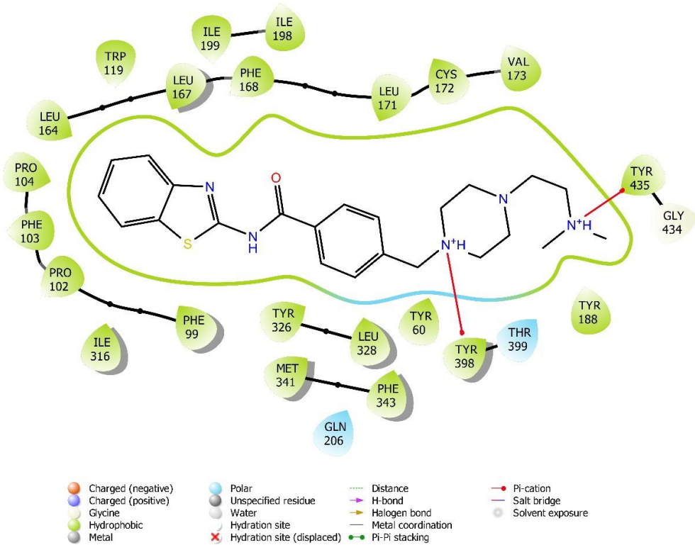
Şekil 5.78. Bileşik 4f 'nin MAO-B enzim aktif bölgesiyle etkileşiminin iki boyutlu görünümü.
