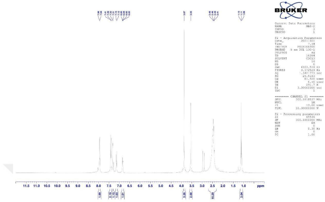
Şekil 5.43. Bileşik 4i'ye ait ^1\text{H} -NMR spektrumu
