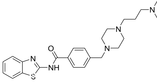
Şekil 5.31. N-(benzo[d]tiyazol-2-il)-4-((4-(3-(dimetilamino)propil)piperazin-1-il)metil)benzamid (4g)
