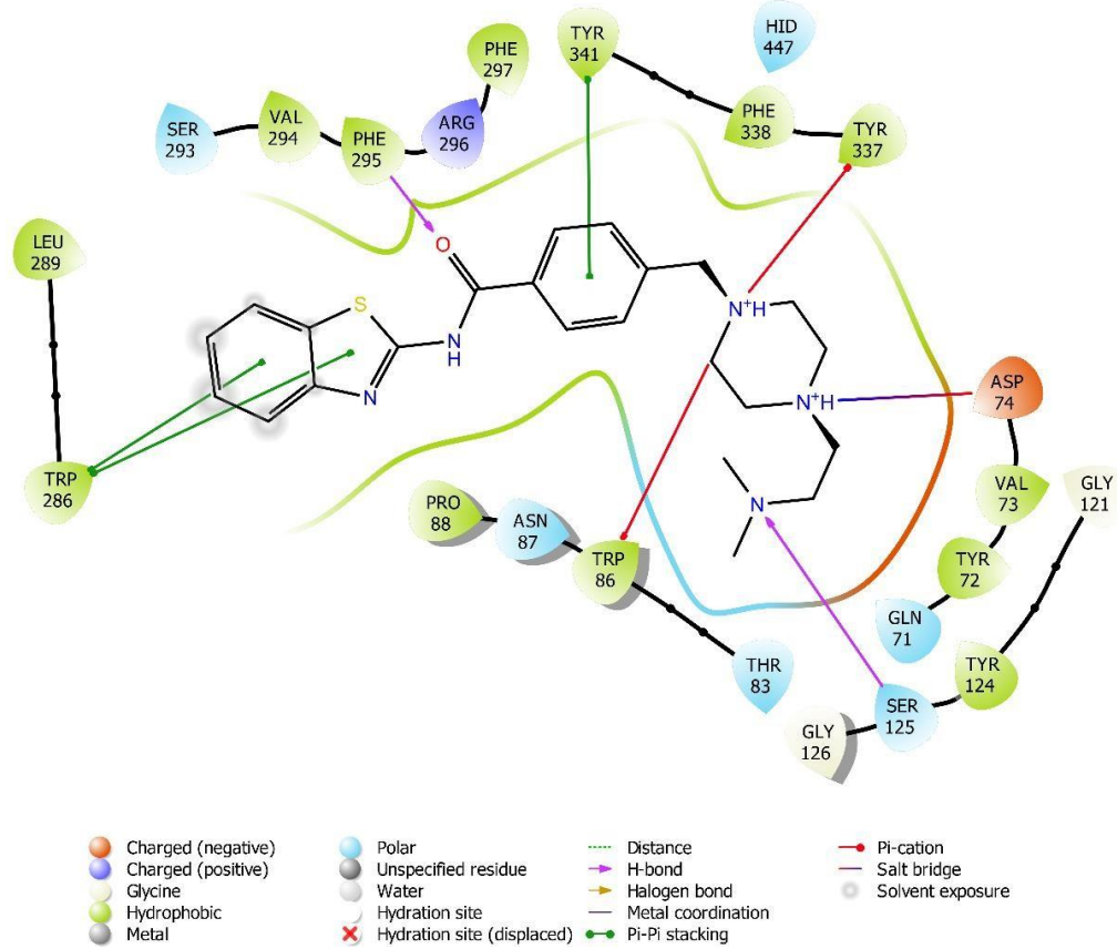
Şekil 5.75. Bileşik 4f'nin AChE enzim aktif bölgesiyle etkileşiminin iki boyutlu görünümü.
