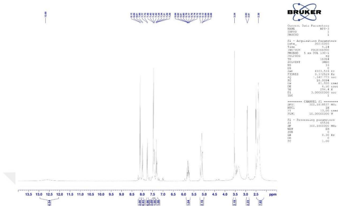
Şekil 5.13. Bileşik 4c'ye ait ^1\text{H} -NMR spektrumu
