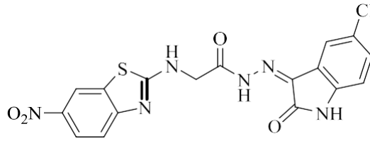
Şekil 2.28 N'-(5-Kloro-2-oksoindolin-3-iliden)-2-(6-nitrobenzotriazol-2-ilamino)asetohidrazid bileşiğine ait kimyasal yapı
