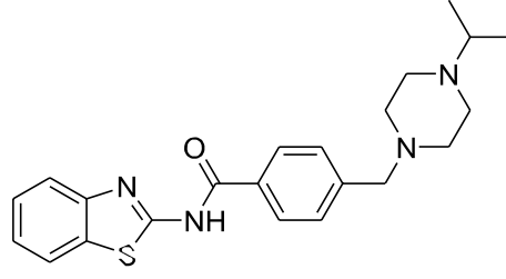
Şekil 5.21. N -(benzo[d]tiyazol-2-il)-4-((4-izopropilpiperazin-1-il)metil)benzamid ( 4e )
