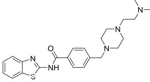
Şekil 5.26. N-(benzo[d]tiyazol-2-il)-4-((4-(2-(dimetilamino)etil)piperazin-1-il)metil)benzamid (4f)
