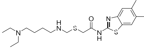
Şekil 2.21 2-[[[(4-(Dietilamino)bütıl)amino)metil]tio]-N-(5,6-dimetilbenzo[d]tiyazol-2-il)asetamid bileşiğine ait kimyasal yapı
