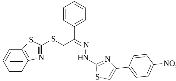
Şekil 2.33 2-((2-(2-(4-(4-Nitrofenil)tiyazol-2-il)hidraziniliden)-2-feniletil)tiyo)benzotiyazol bileşiğıne ait kimyasal yapı
