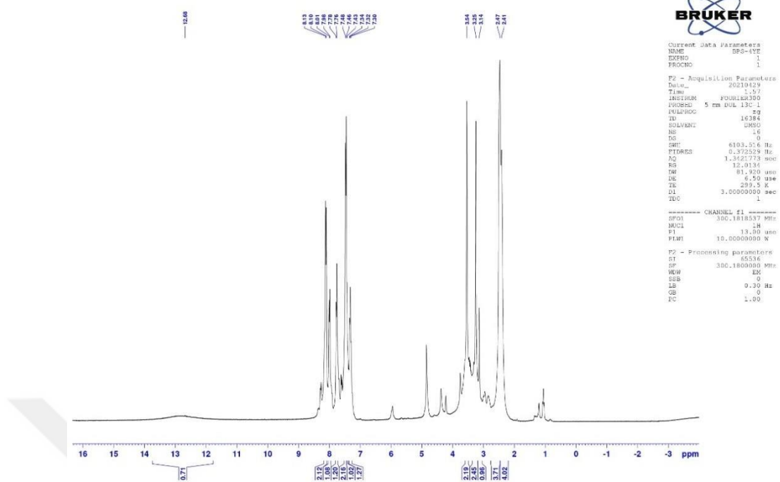
Şekil 5.18. Bileşik 4d'ye ait ^1\text{H} -NMR spektrumu
