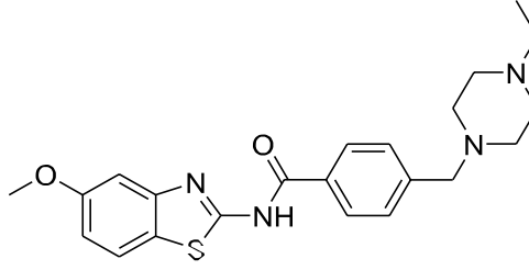
Şekil 5.41. 4-((4-etilpiperazin-1-il)metil)-N-(5-metoksibenzo[d]tiyazol-2-il)benzamid ( 4i )
