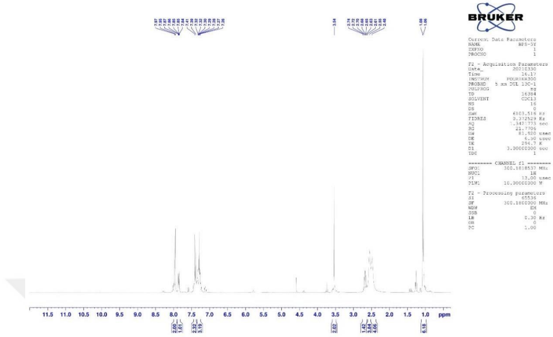
Şekil 5.23. Bileşik 4e'ye ait ^1\text{H} -NMR spektrumu
