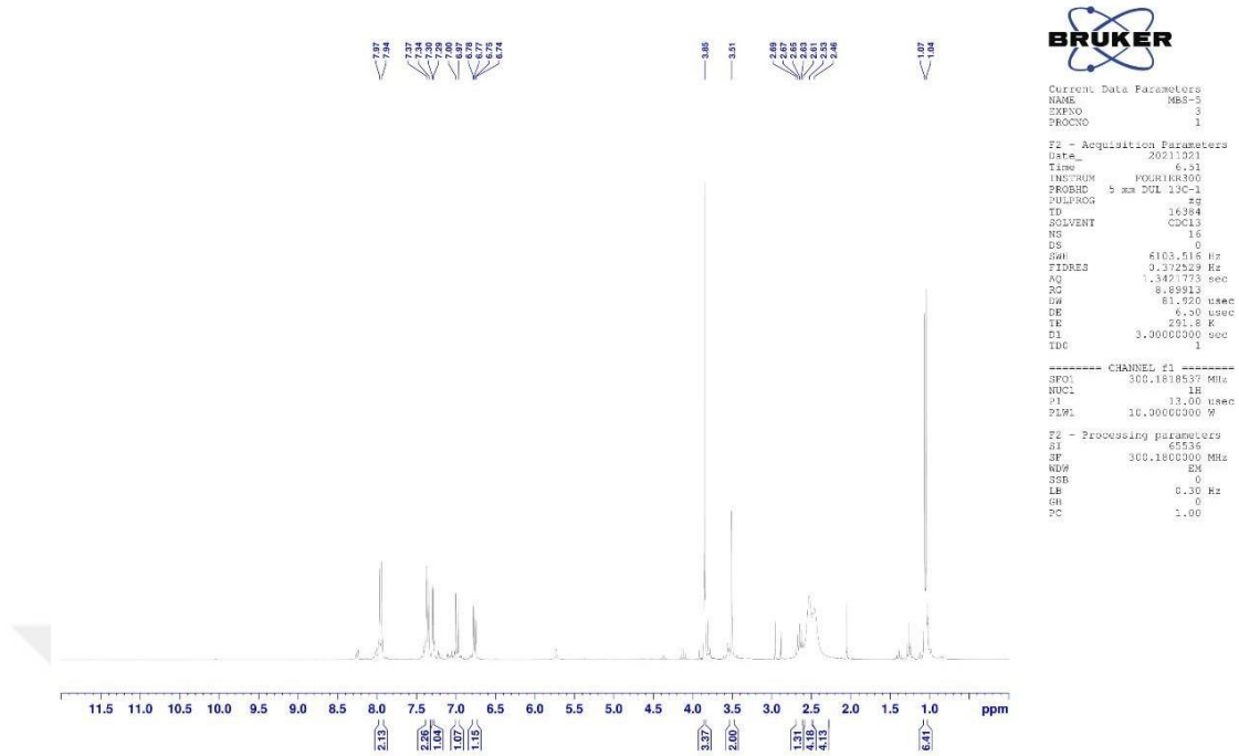
Şekil 5.58. Bileşik 4I'ye ait ^1\text{H} -NMR spektrumu
