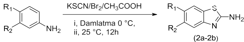
Şekil 4.2. 2-Aminobenzotiyazol türevlerinin sentezi
