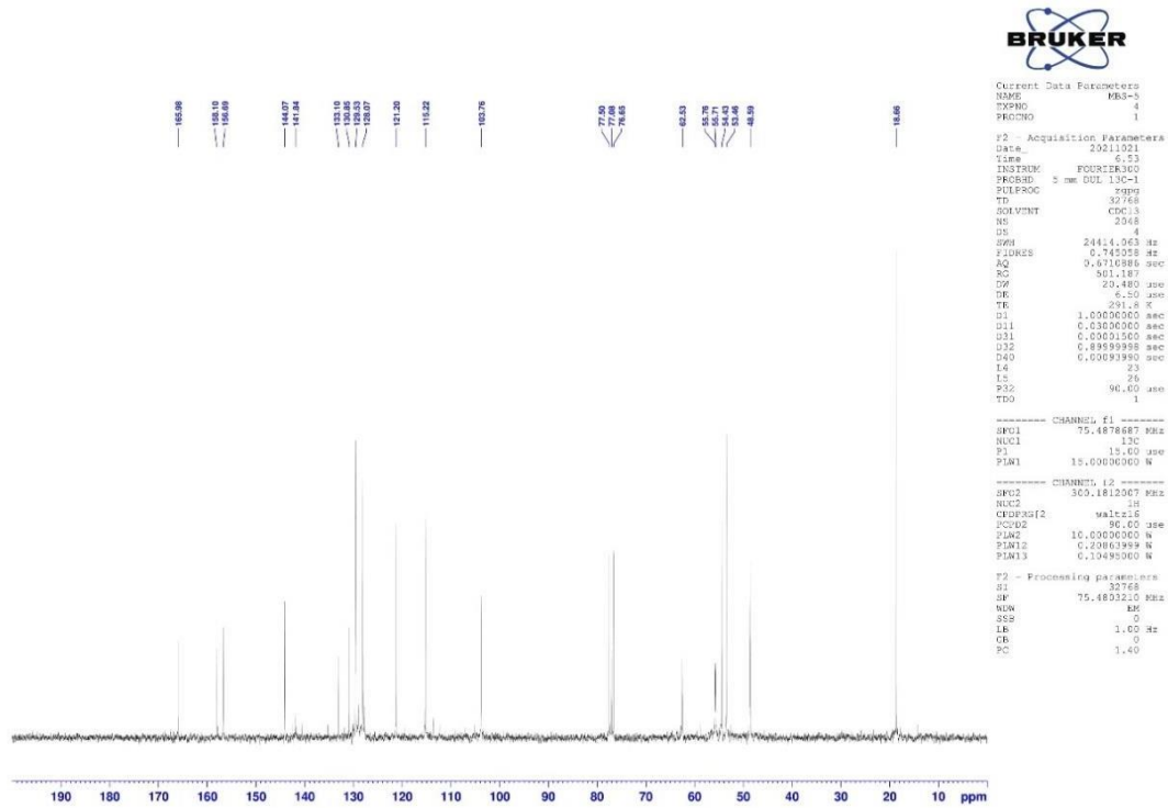
Şekil 5.59. Bileşik 4I'ye ait ^{13}\text{C} -NMR spektrumu
