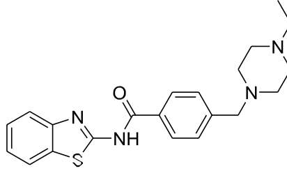
Şekil 5.6. N-(benzo[d]tiyazol-2-il)-4-((4-etilpiperazin-1-il)metil)benzamid (4b)
