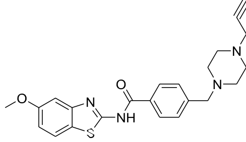
Şekil 5.51. N -(5-metoksibenzo[d]tiyazol-2-il)-4-((4-(prop-2-in-1-il)piperazin-1-il)metil)benzamid ( 4k )
