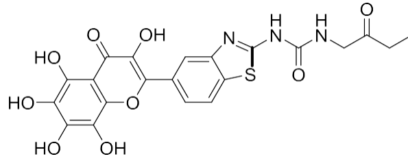
Şekil 2.14 1-(2-oksobütil)-3-(5-(3,5,6,7,8-pentahidroksi-4-okso-4H-kromen-2-il)benzo[d]tiyazol-2-il)üre bileşiğine ait kimyasal yapı
