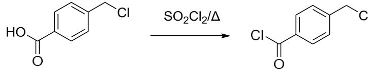
Şekil 4.1. 4-(Klorometil)benzoil klorür sentezi
