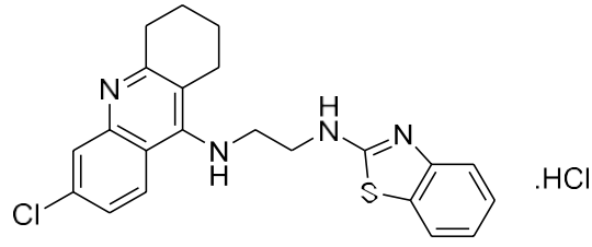
Şekil 2.26 N 1 -(benzo[d]tiyazol-2-il)- N 2 -(6-kloro-1,2,3,4-tetrahidroakridin-9-il)etan-1,2-diamin hidroklorid bileşiğine ait kimyasal yapı
