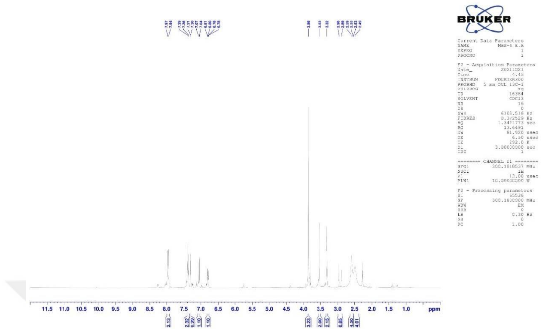
Şekil 5.53. Bileşik 4k'ye ait ^1\text{H} -NMR spektrumu
