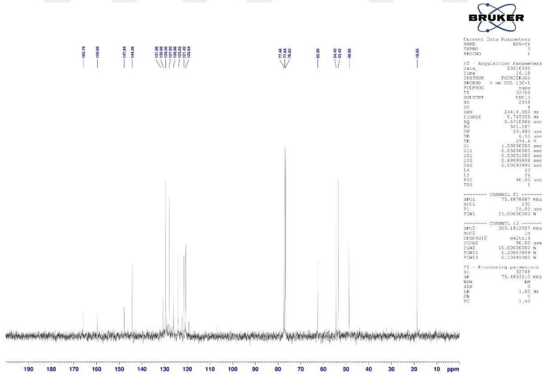
Şekil 5.24. Bileşik 4e'ye ait ^{13}\text{C} -NMR spektrumu
