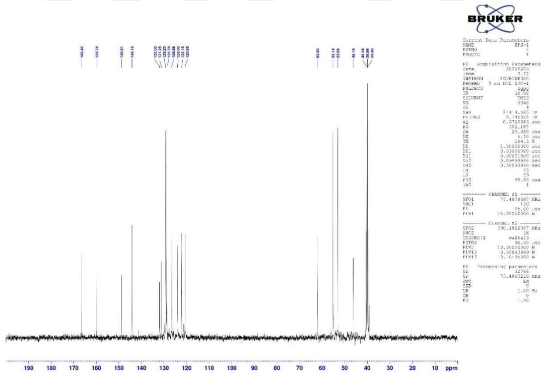
Şekil 5.4. Bileşik 4a'ya ait ^{13}\text{C} -NMR spektrumu
