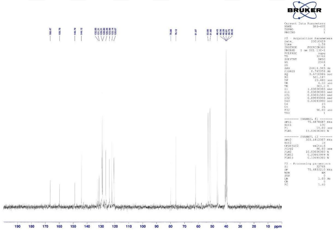
Şekil 5.19. Bileşik 4d'ye ait ^{13}\text{C} -NMR spektrumu
