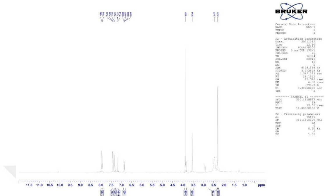
Şekil 5.38. Bileşik 4h'ye ait ^1\text{H} -NMR spektrumu
