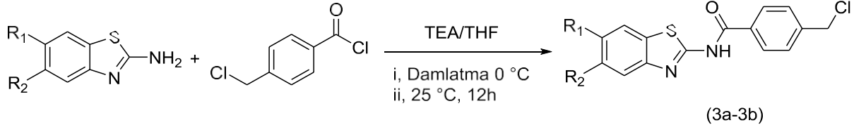
Şekil 4.3. 4-(Klorometil)-N-(5,6-süstitübenzo[d]tiyazol-2-il)benzamid sentezi
