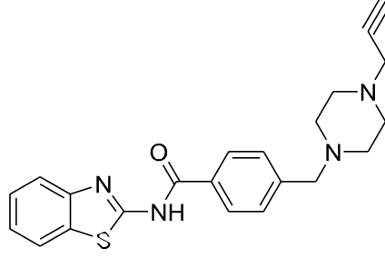
Şekil 5.16. N-(benzo[d]tiyazol-2-il)-4-((4-(prop-2-in-1-il)piperazin-1-il)metil)benzamid ( 4d )
