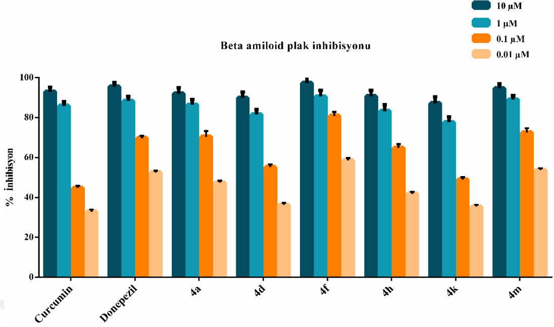
Şekil 5.73. 4a, 4d, 4f, 4h, 4k ve 4m kodlu bileşiklerin Beta amiloid plak inhibisyonu (%)
