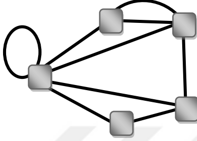
Şekil 2.12: Pseudo Graf Örneği
