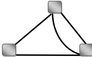
Şekil 2.11: Çoklu Graf Örneği
