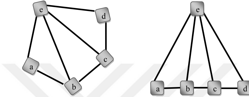
Şekil 2.31: İzomorfik Graflar
