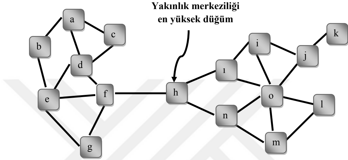
Şekil 3.5: Yakınlık Merkezilik Ölçütü ile İlgili Bir Sosyal Ağ Örneği
