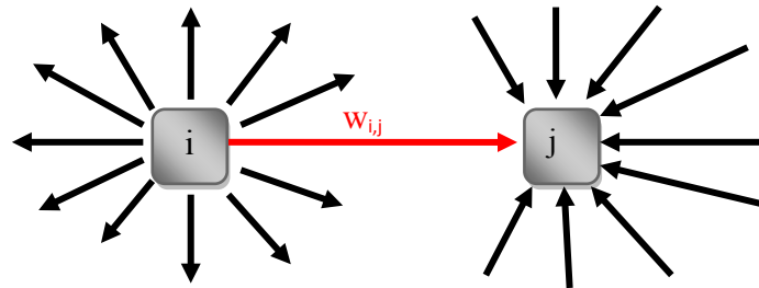
Şekil 4.1: i düğümünden j düğümüne giden çoklu kenar w_{ij}
