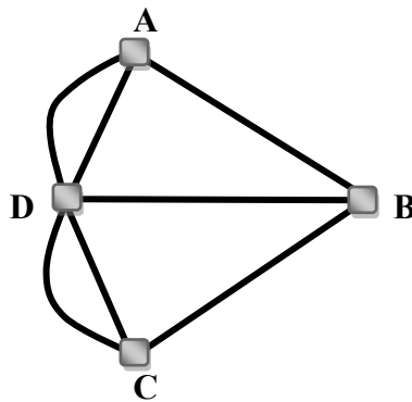
Şekil 2.29: Euler Döngüsü
