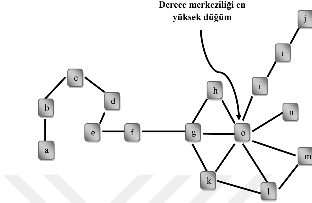
Şekil 3.2: Derece Merkezilik Ölçütü ile İlgili Bir Sosyal Ağ Örneği
