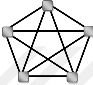
Şekil 2.17: Tam Graf Örneği
