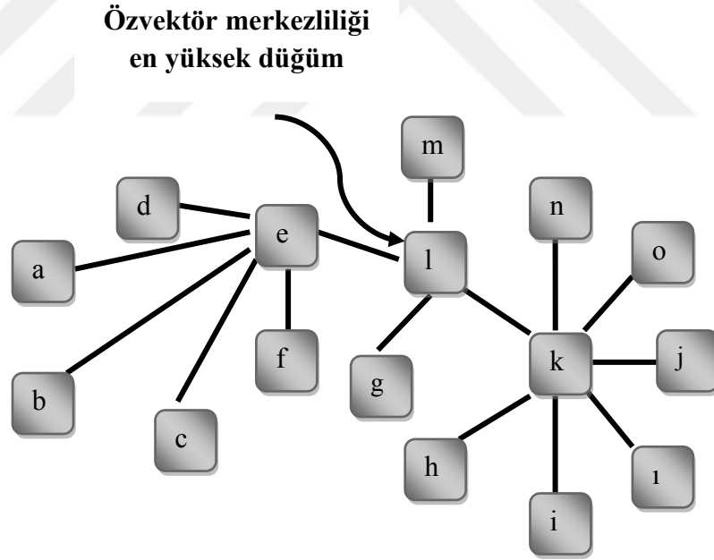
Şekil 3.7: Özvektör Merkezilik Ölçütü ile İlgili Bir Sosyal Ağ Örneği
