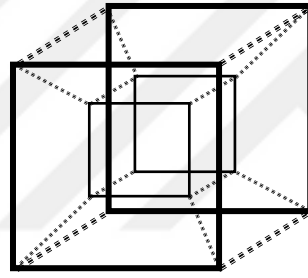
Şekil 2.22: Hiperküp Graf Örneği
