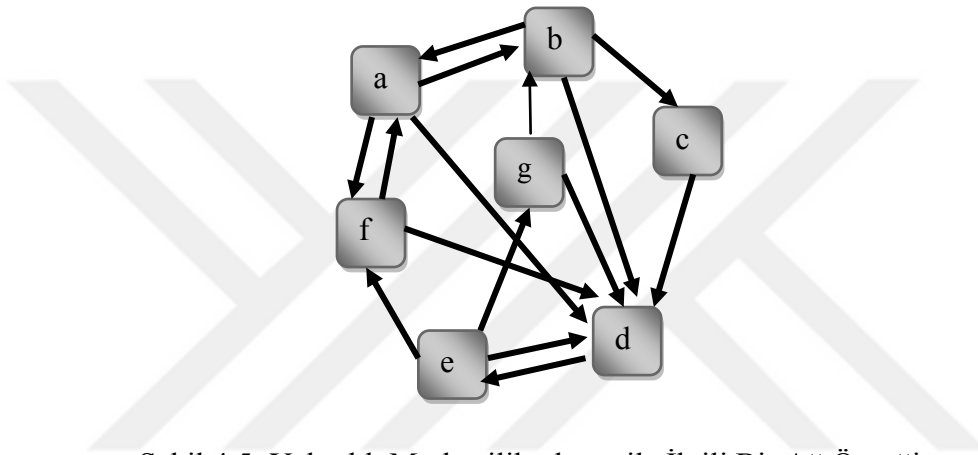
Şekil 4.5: Yakınlık Merkezilik ölçütü ile ilgili bir ağ örneği
