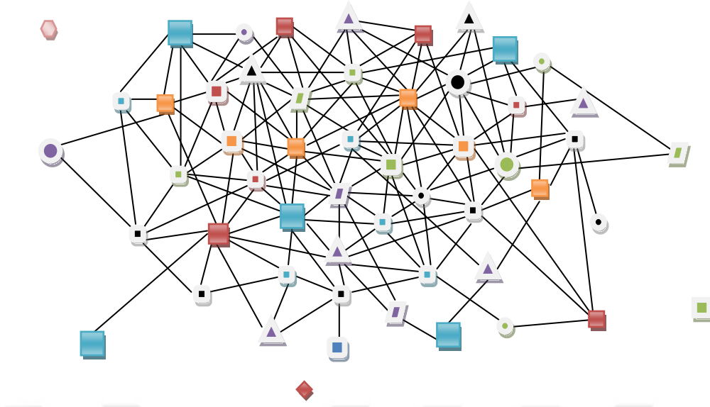
Şekil 3.1: Karmaşık Bir Ağ Yapısı Örneği
