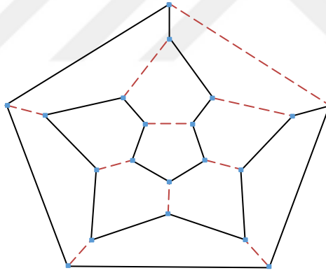
Şekil 2.30: Hamilton Döngüsü
