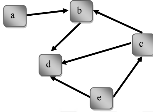
Şekil 2.32: Yönlü Graf Örneđi
