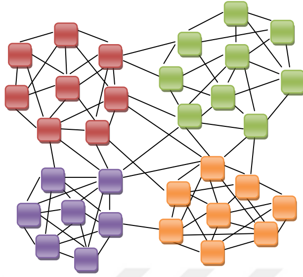
Şekil 2.34: Bir Graftaki D ğ m K melerinin G sterimi
