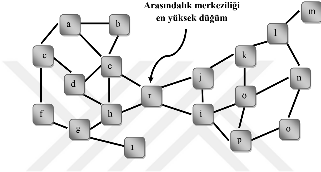
Şekil 3.6: Arasındalık Merkezilik Ölçütü ile İlgili Bir Sosyal Ağ Örneği
