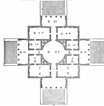
Figure 16 - Villa Rotonda in the Quattro Libri Dell'Architettura - Palladio -1570 60
