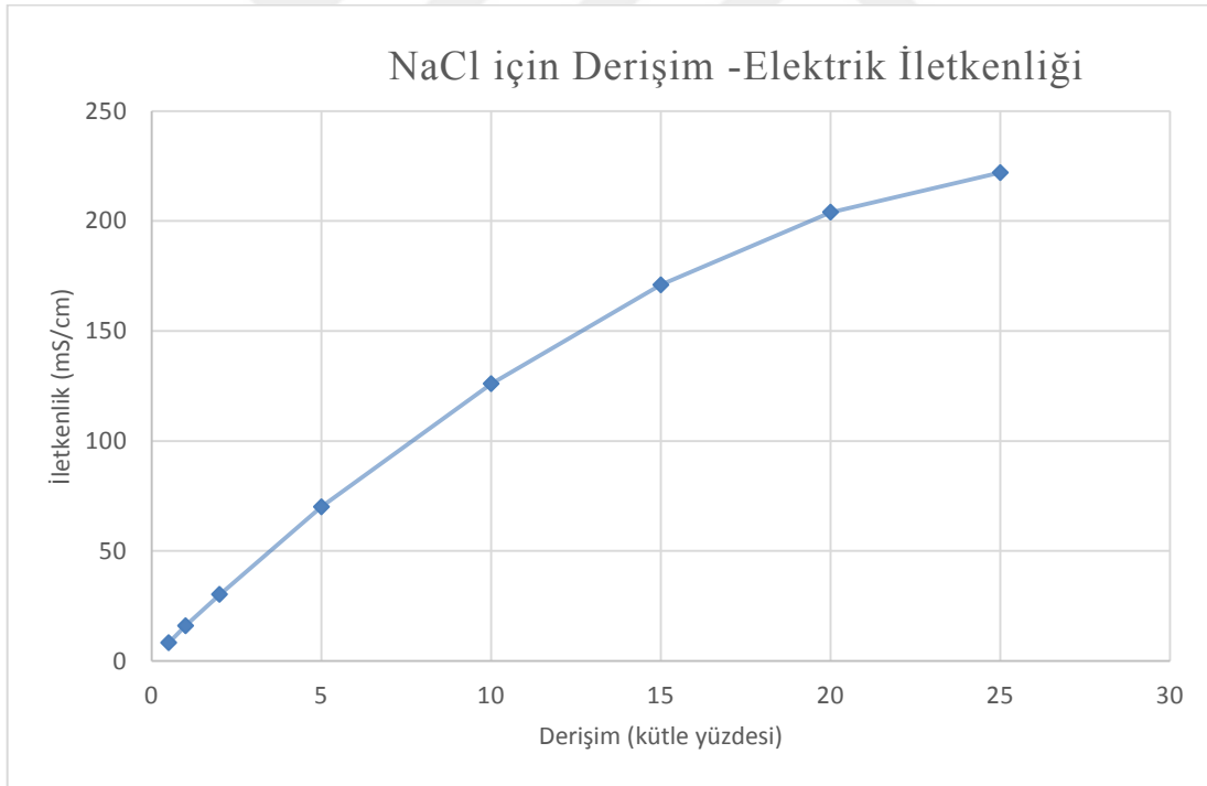
Şekil 3-2. NaCl'e ait Derişim-İletkenlik grafiğı
