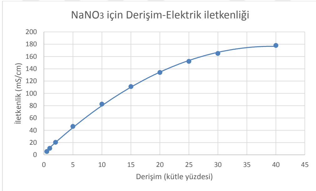
Şekil 3-4. NaNO 3 'e ait Derişim-İletkenlik grafiđi
