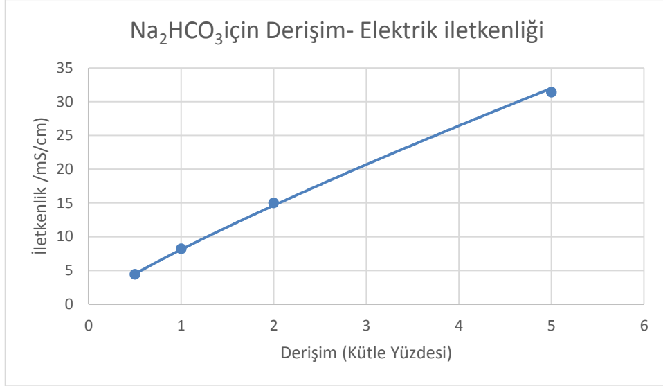
Şekil 3-5. Na 2 HCO 3 'e ait Derişim-İletkenlik grafiđi
