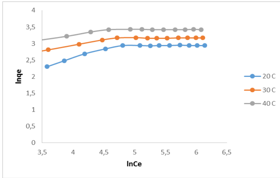
Şekil 4.16. Farklı sıcaklıklarda YNK'nın Pb^{+2} biyosorpsiyonu için freundlich izoterm grafiği
