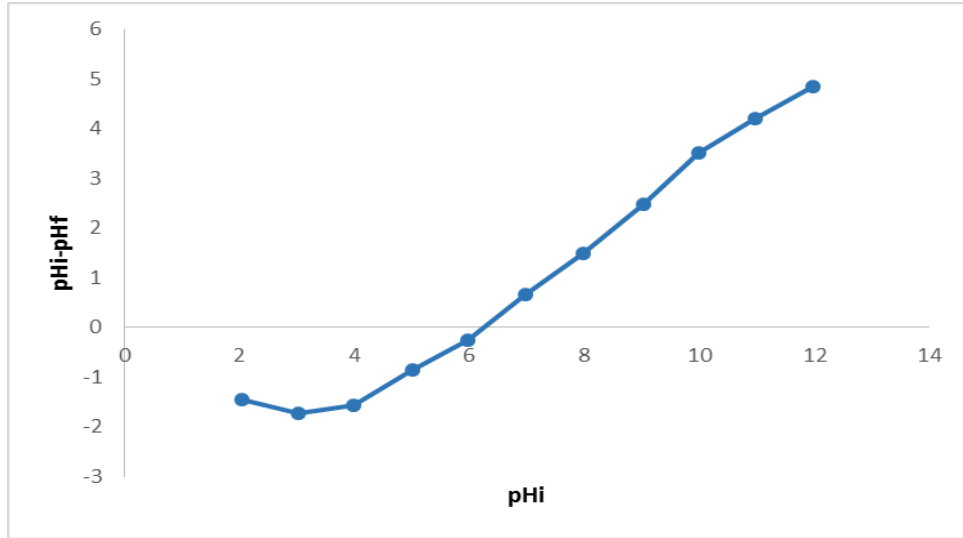
Şekil 4.7. YNK için pH_{syn} belirlenmesine ilişkin grafik
