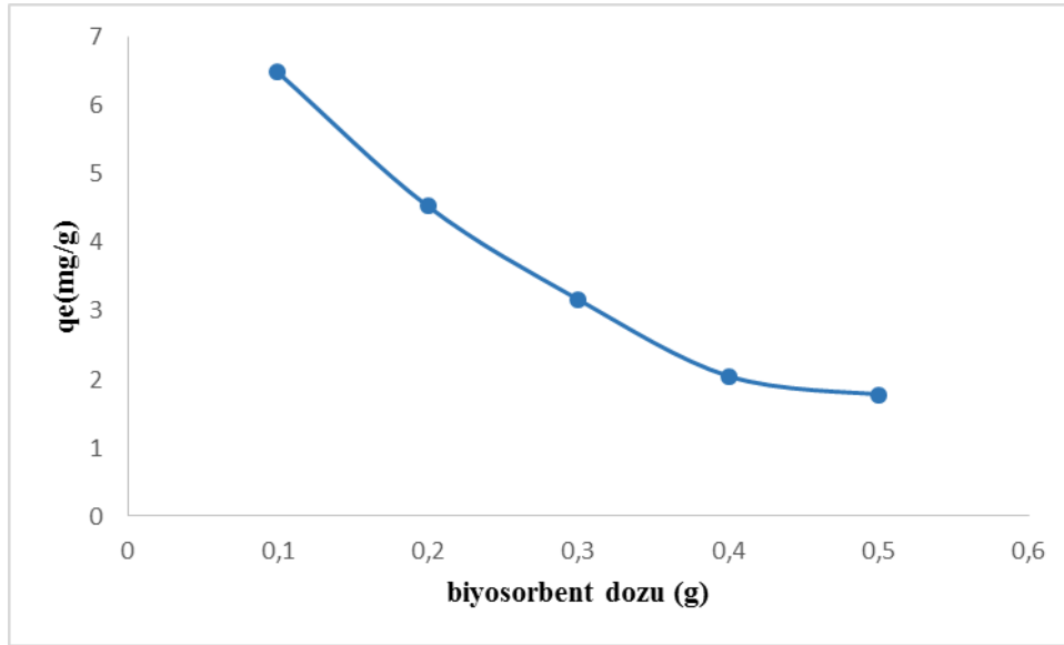
Şekil 4.19. DCF biyosorsiyonunda, biyosorbent dozunun biyosorplama kapasitesine etkisi
