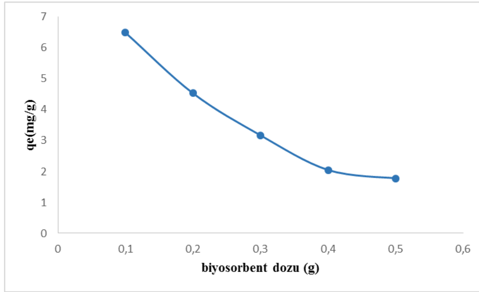
Şekil 4.8. Pb^{+2} biyosorpsiyonunda, biyosorbent dozunun biyosorplama kapasitesine etkisi
