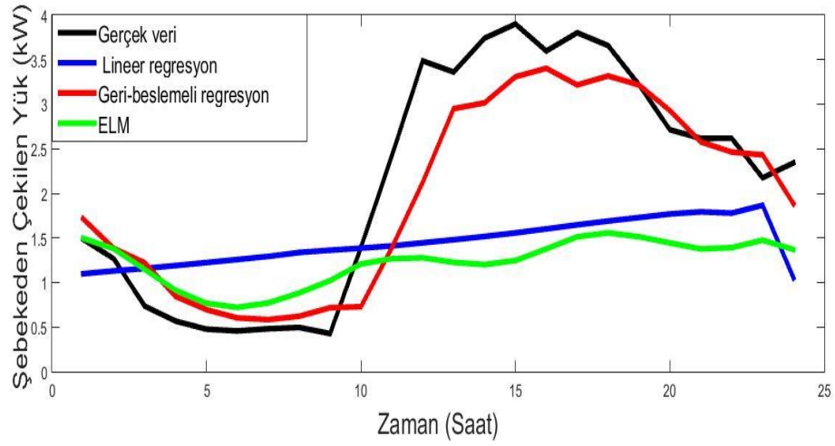
Şekil 7.8. 2714 numaralı meskene ait bir günlük şebeke yük tahmini eğrileri
