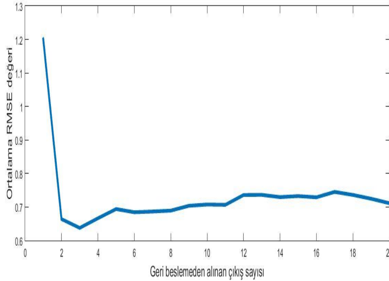
Şekil 7.2. 1135 numaralı mesken için GBLR metodunda geri besleme eleman sayısına göre ortalama RMSE değişimleri
